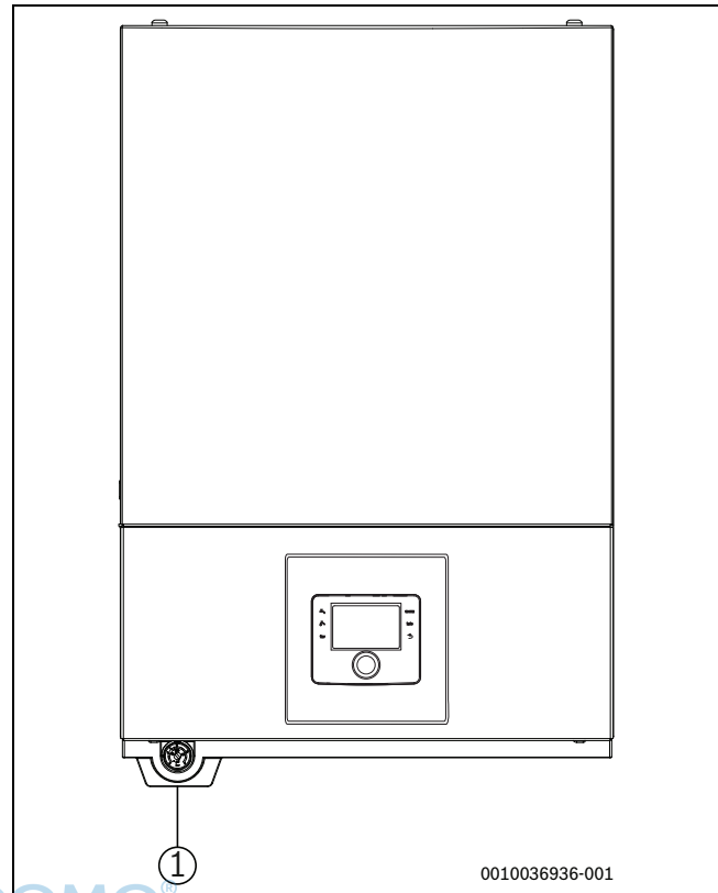
Bild 5 Inneneinheit AWS E (Ansicht mit Auffangbehälter)
