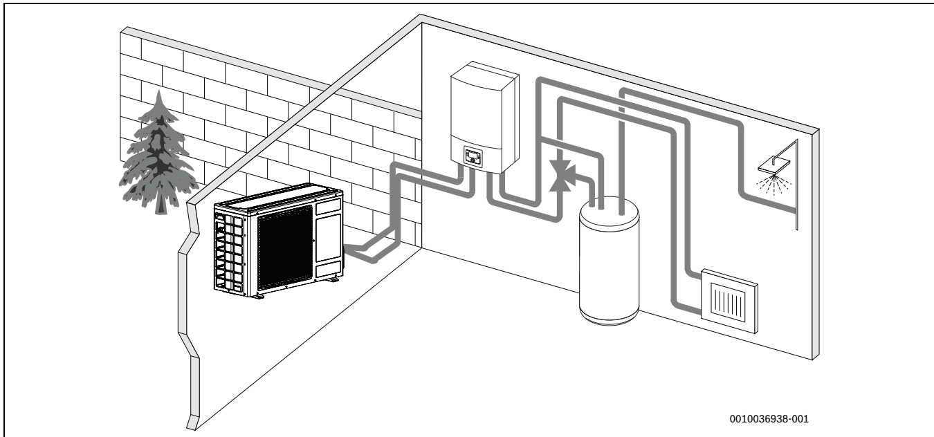
Bild 2 Wärmepumpe als Außeneinheit, Inneneinheit AWS E mit integriertem Warmwasserspeicher und elektrischem Zuheizer
