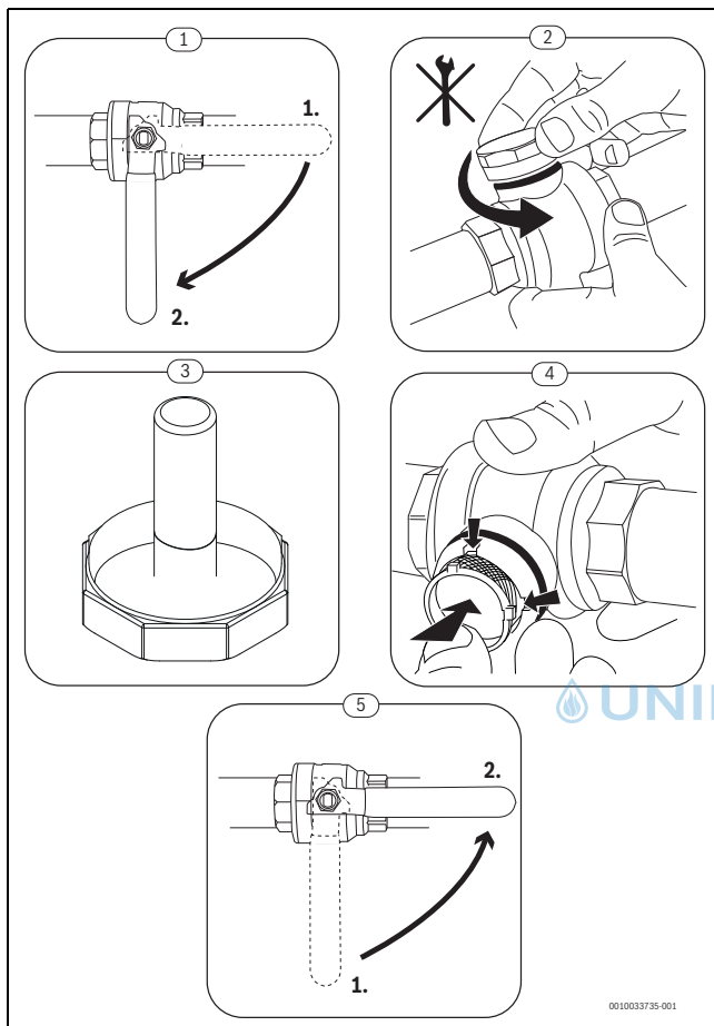
Bild 6 Siebreinigung
