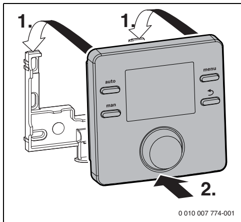
Bild 5 Bedieneinheit einhängen
