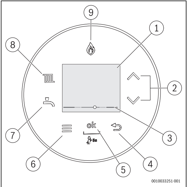
Bild 6 Bedienfeld
