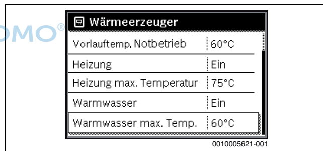
Bild 18 Maximale Warmwassertemperatur
