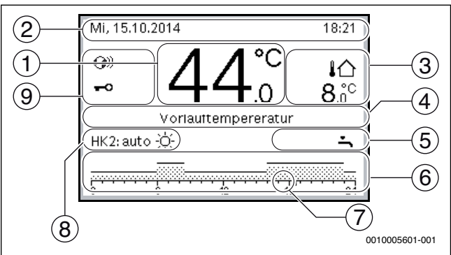
Bild 3 Beispiel für die Standardanzeige bei einer Anlage mit mehreren Heizkreisen
