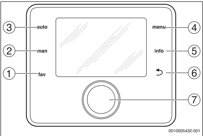
Bild 2 Bedienelemente
