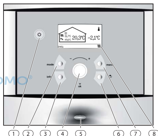
Bild 3 Bedienfeld
