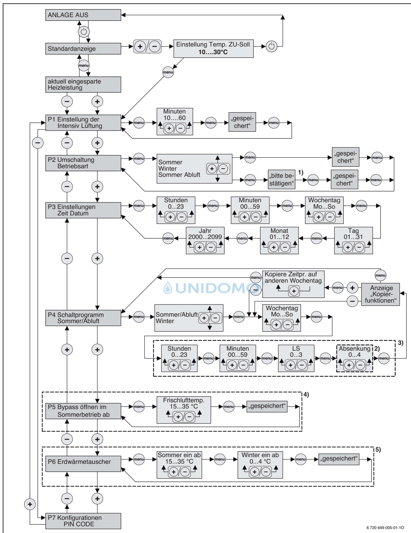
Bild 7 Menüstruktur der Benutzerebene
