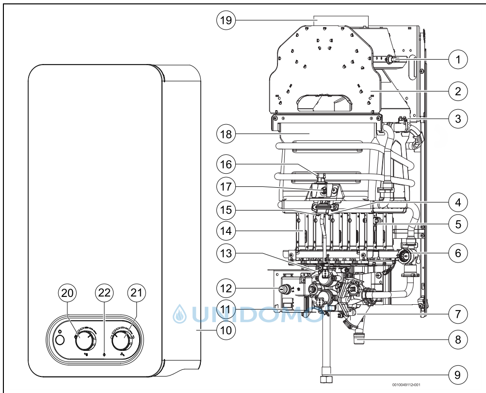
Bild 2 Gerätedesign
