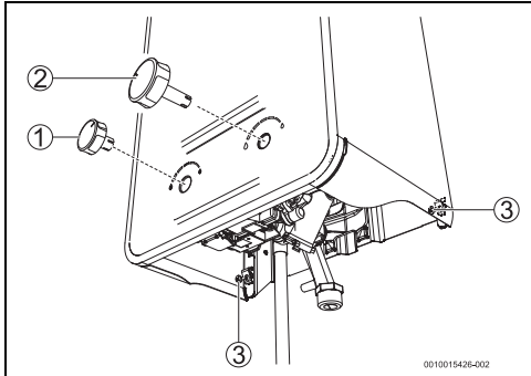
Bild 17 Verkleidung entfernen
