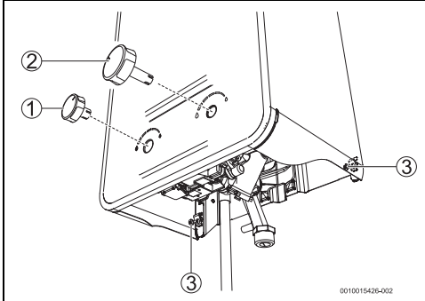
Bild 18 Verkleidung entfernen
