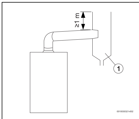
Bild 11 Kondensatsiphon
