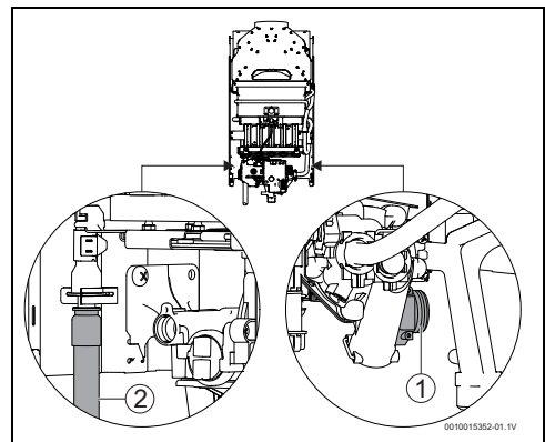
Bild 15 Wasseranschluss
