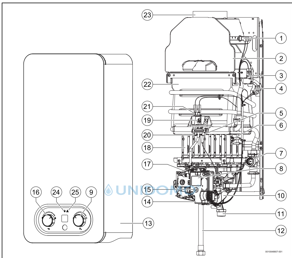
Bild 2 Geräteübersicht
