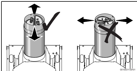
Bild 12 Abgasklappe montieren
