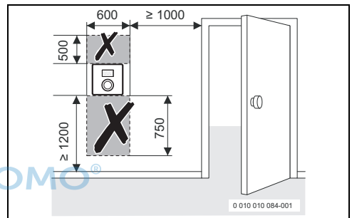
Bild 5 Installationsort Bedieneinheit
