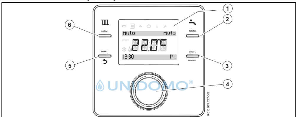
Bild 1 Bedieneinheit
