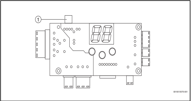
Bild 3 Anschluss D der Heizgerätbedieneinheit
