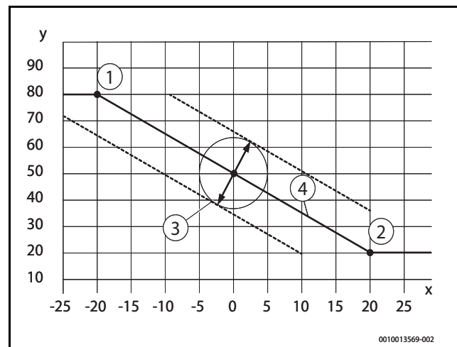
Bild 5 Außentemperaturgeführte Heizkurve
