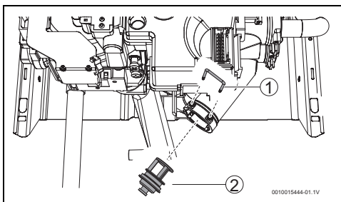
Bild 9 Entleeren
