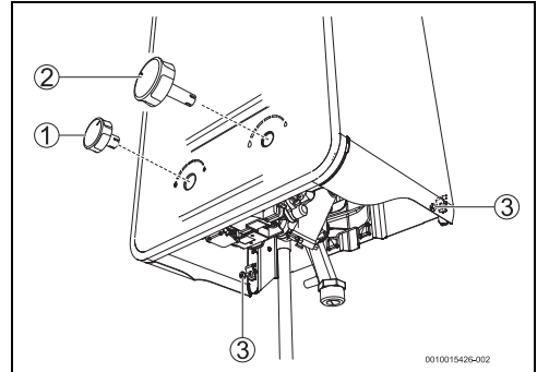
Bild 19 Verkleidung entfernen
