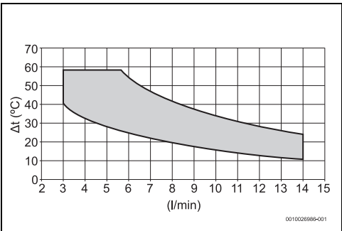
Bild 30 14-Liter-Modell
