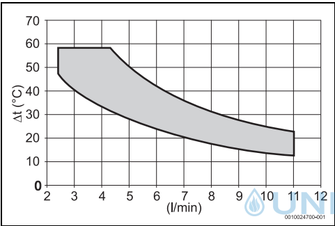
Bild 29 10-Liter-Modell
