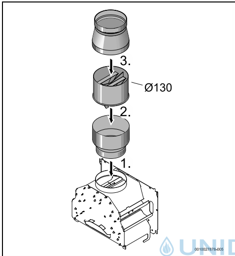
Bild 14 Ø 130 mm montieren
