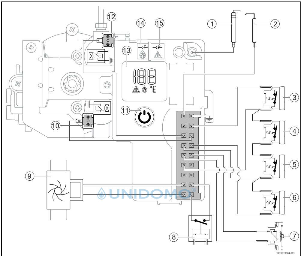
Bild 28 Schaltplan
