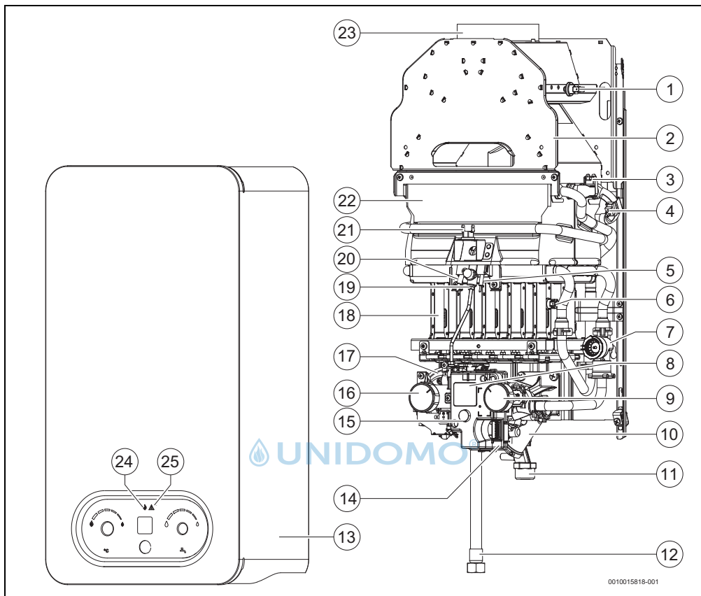
Bild 2 Geräteübersicht
