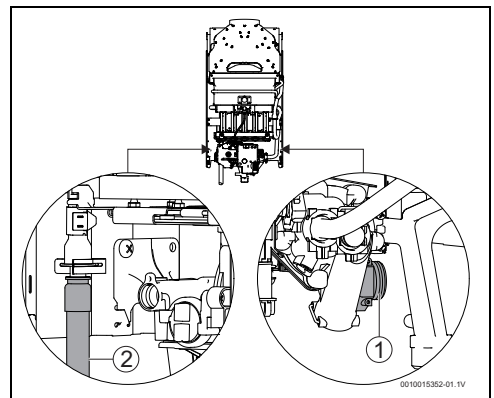
Bild 16 Wasseranschluss
