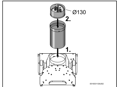
Bild 15 Ø 130 mm montieren
