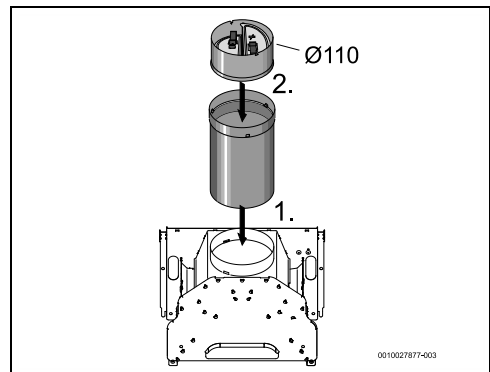
Bild 13 Ø 110 mm montieren
