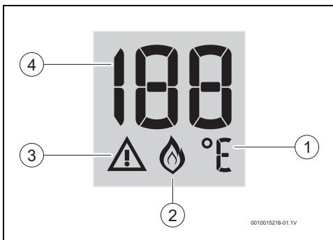
Bild 3 Digitalanzeige
