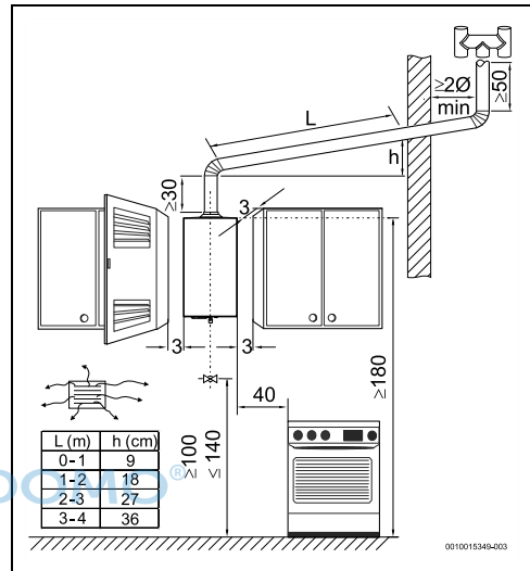
Bild 9 Mindestabstände (cm)
