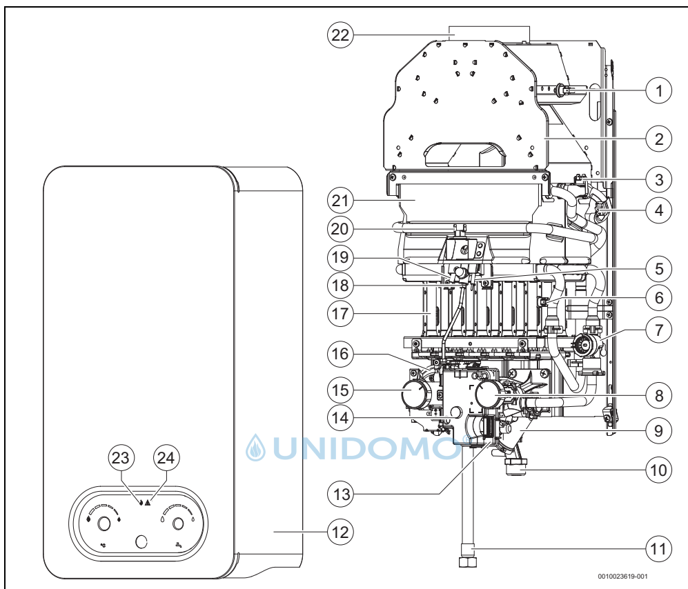
Bild 2 Geräteübersicht
