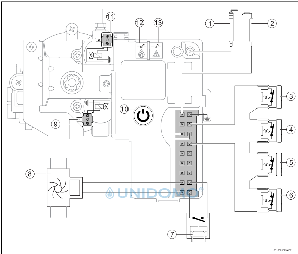
Bild 26 Schaltplan
