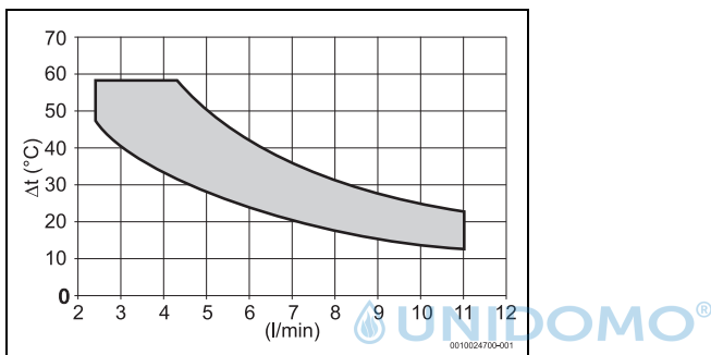
Bild 27 10-Liter-Modell
