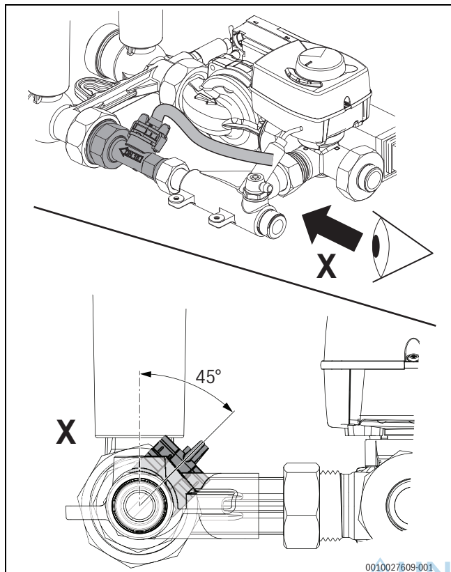
Bild 31 Volumenstromfühler ausrichten
