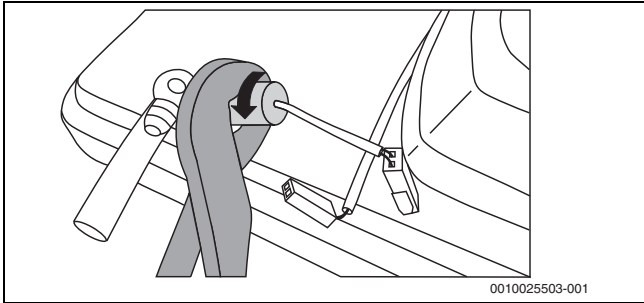
Bild 17 Leitfähigkeitssonde lösen
