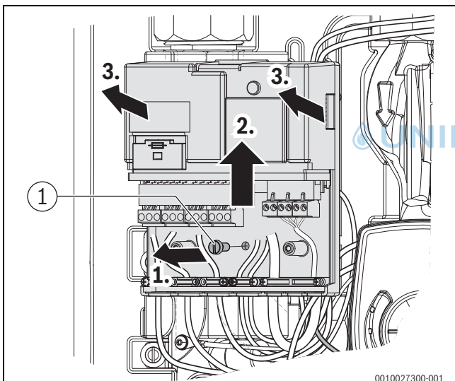
Bild 28 Elektronik-Modul abnehmen
