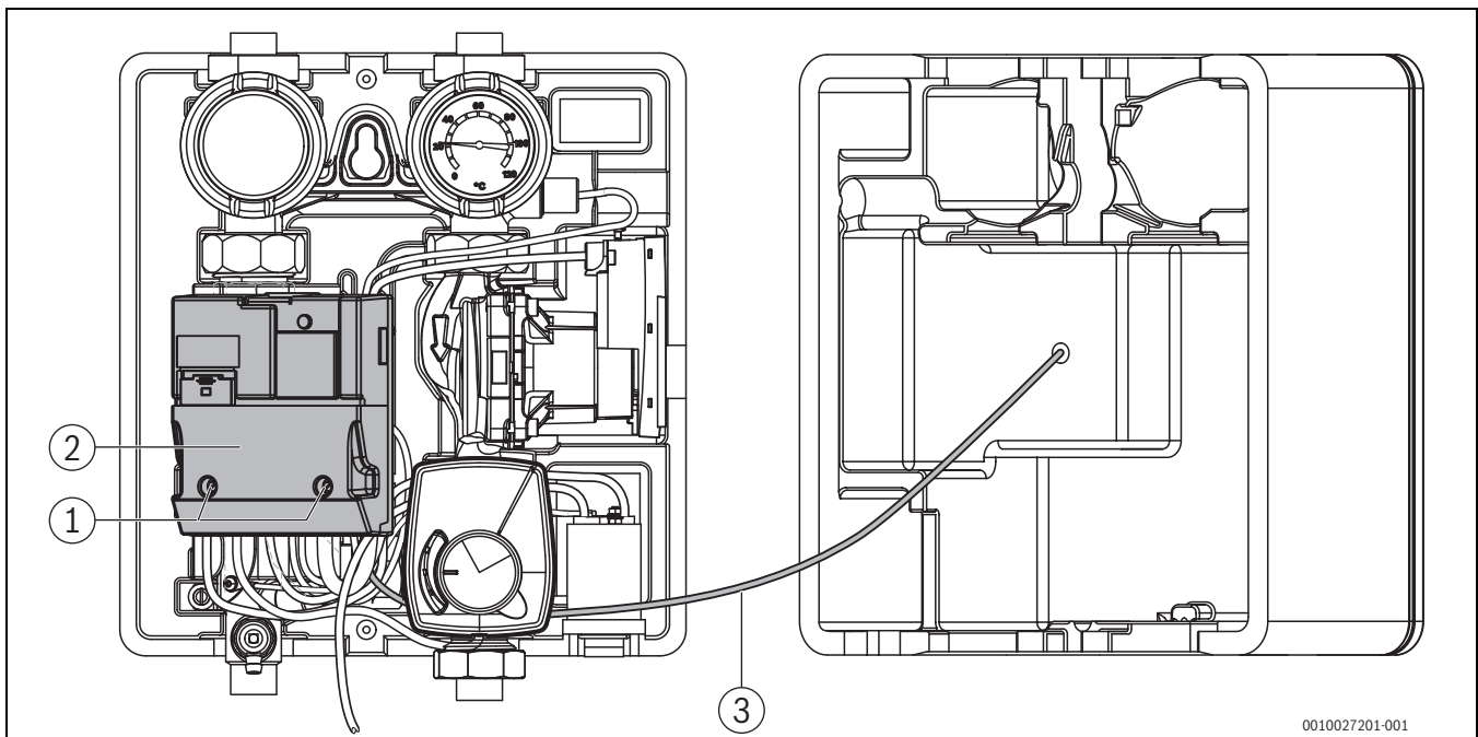
Bild 26 Elektronik-Modul öffnen
