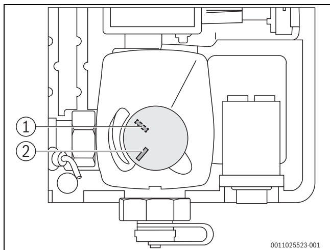
Bild 4 2-Wege-Ventil geschlossen/geöffnet
