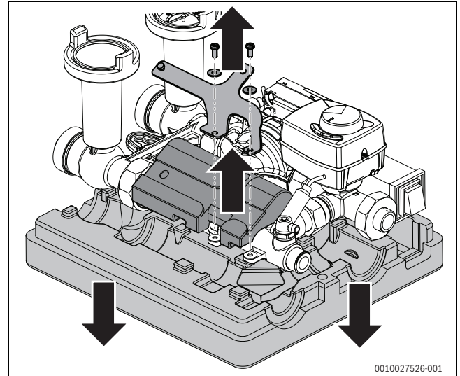
Bild 29 Trägerblech und Wärmeschutz abnehmen
