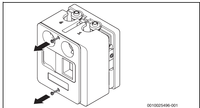
Bild 25 Isolierteil abnehmen
