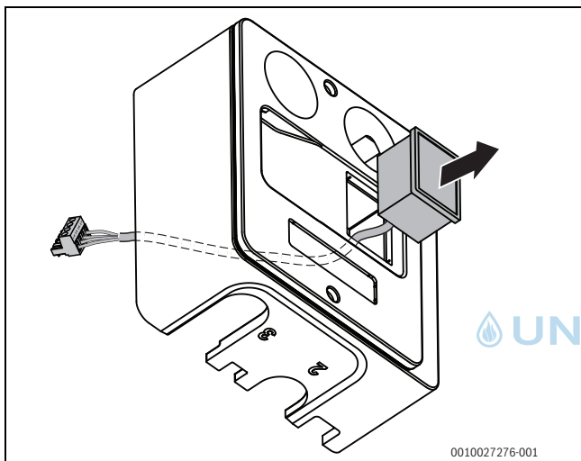
Bild 24 Bedieneinheit entnehmen
