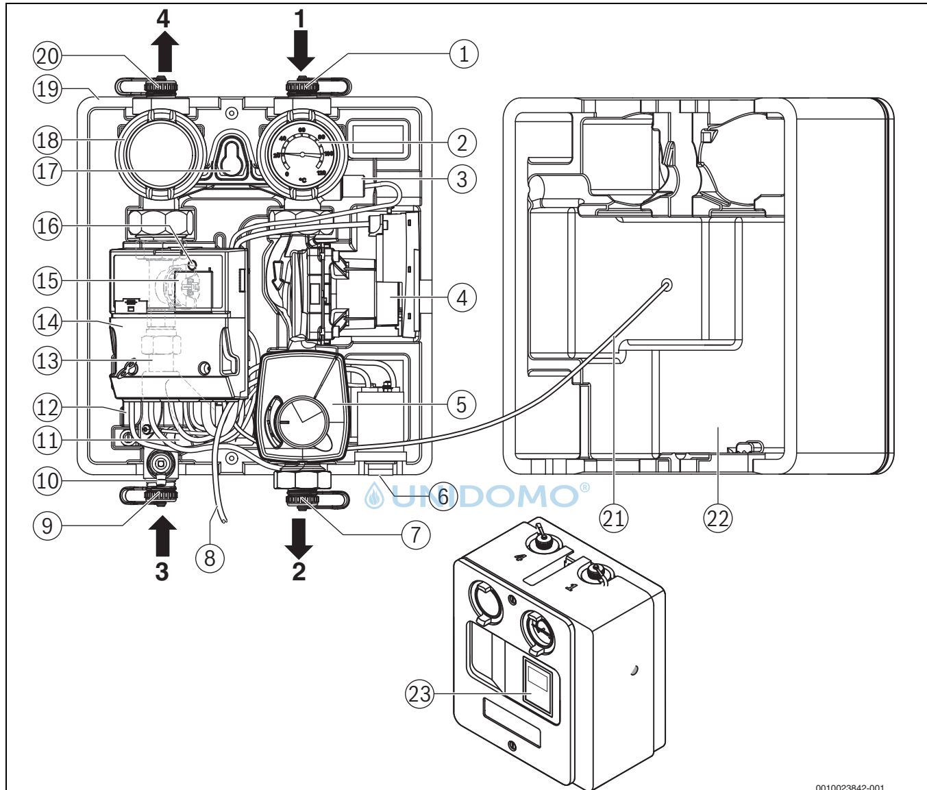
Bild 3 Komponenten Bypassentsalzungsmodul
