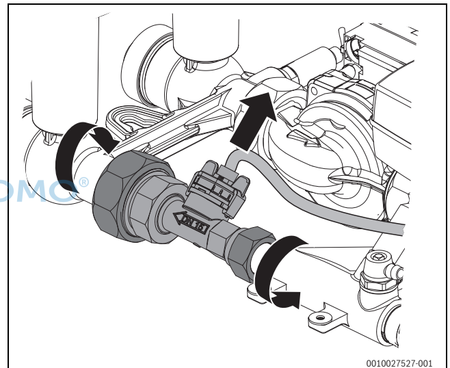
Bild 30 Volumenstromfühler ausbauen
