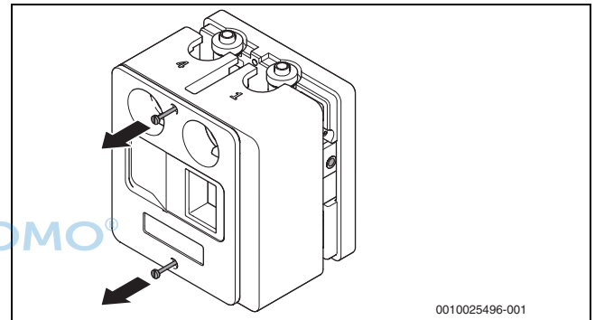
Bild 15 Isolierteil abnehmen
