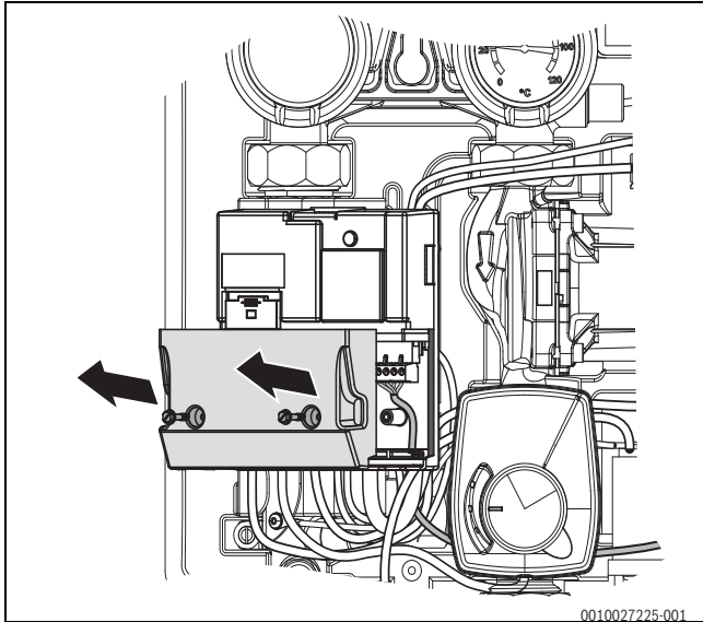
Bild 27 Abdeckung abnehmen
