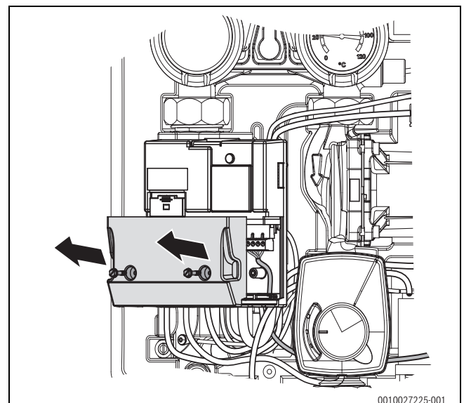
Bild 22 Abdeckung abnehmen
