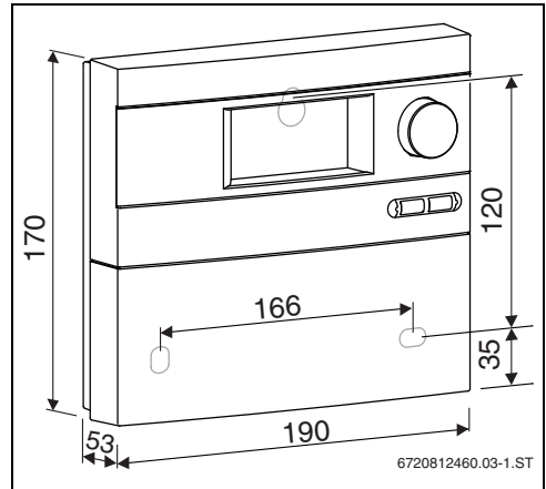
Bild 4 Abmessungen Gehäuse
