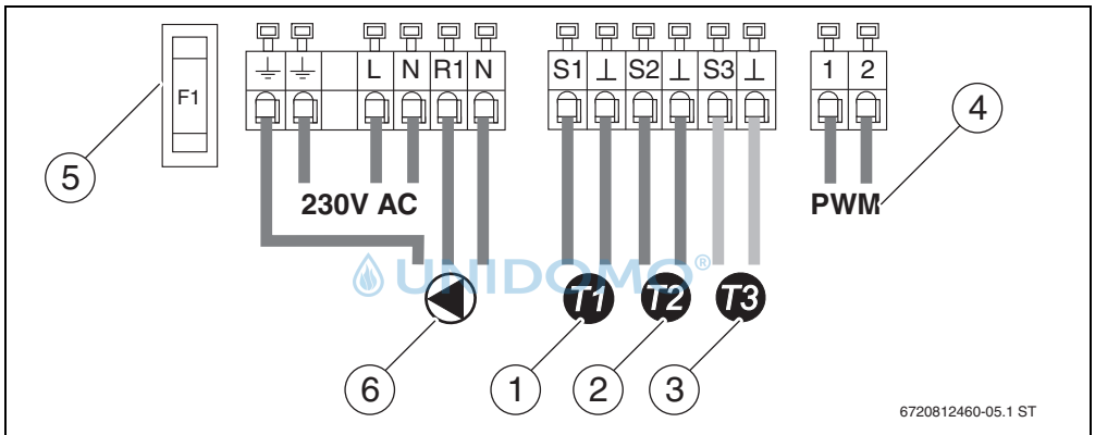
Bild 8 Anschlussplan
