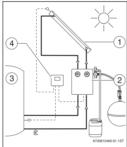
Bild 3 Anlagenschema
