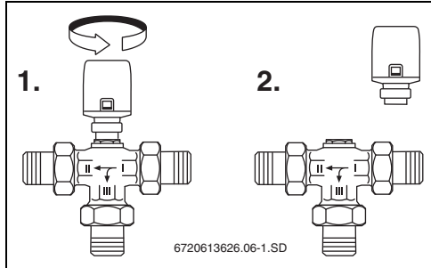
Bild 10 Stellantrieb demontieren
