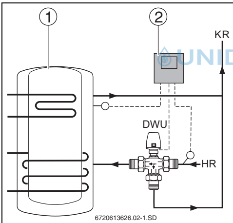
Bild 7 Rücklaufanhebung
