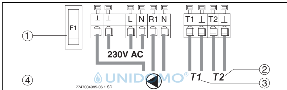
Bild 12 Anschlussplan
