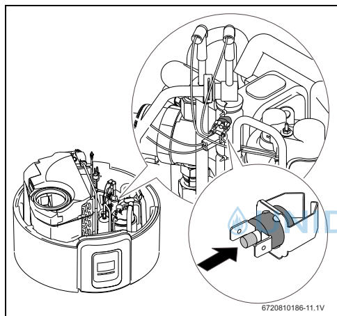
Bild 53 Thermostat
