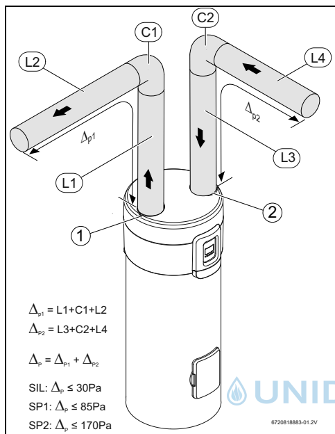
Bild 11 Druckverluste
