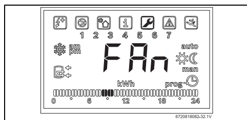
Bild 42 Untermenü "Fan"
