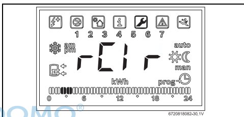
Bild 38 Untermenü "Rcir"
