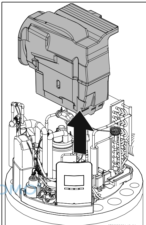
Bild 51 Baugruppe Luftführung und Gebläse entfernen.
