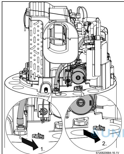
Bild 53 Haltefeder abnehmen
