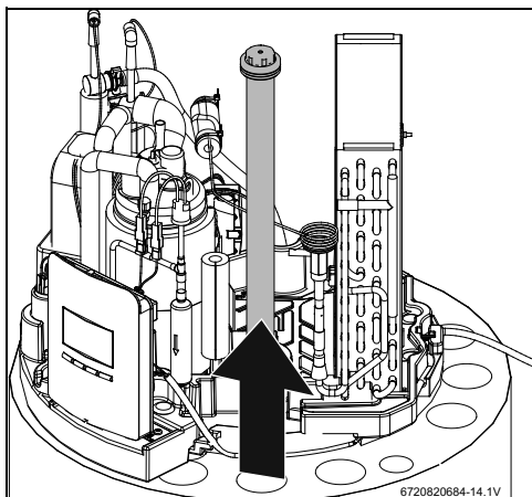
Bild 52 Kontrolle des Zustands der Magnesium-Anode
