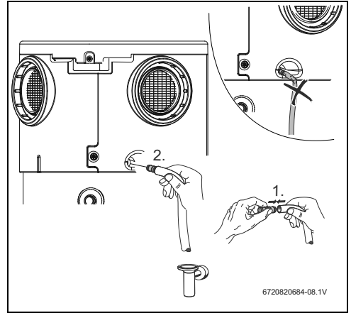
Bild 12 Kondensatabfang
