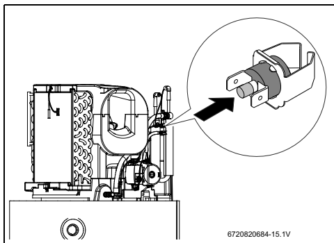
Bild 56 Temperaturbegrenzer
