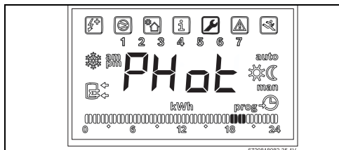
Bild 42 Funktion "Phot"
