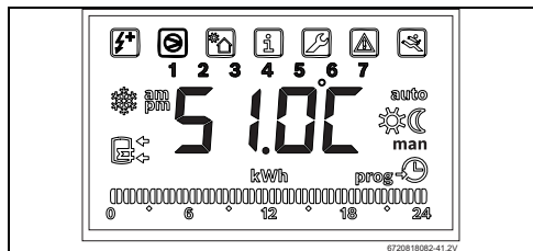
Bild 47 Ausgangsmenü
