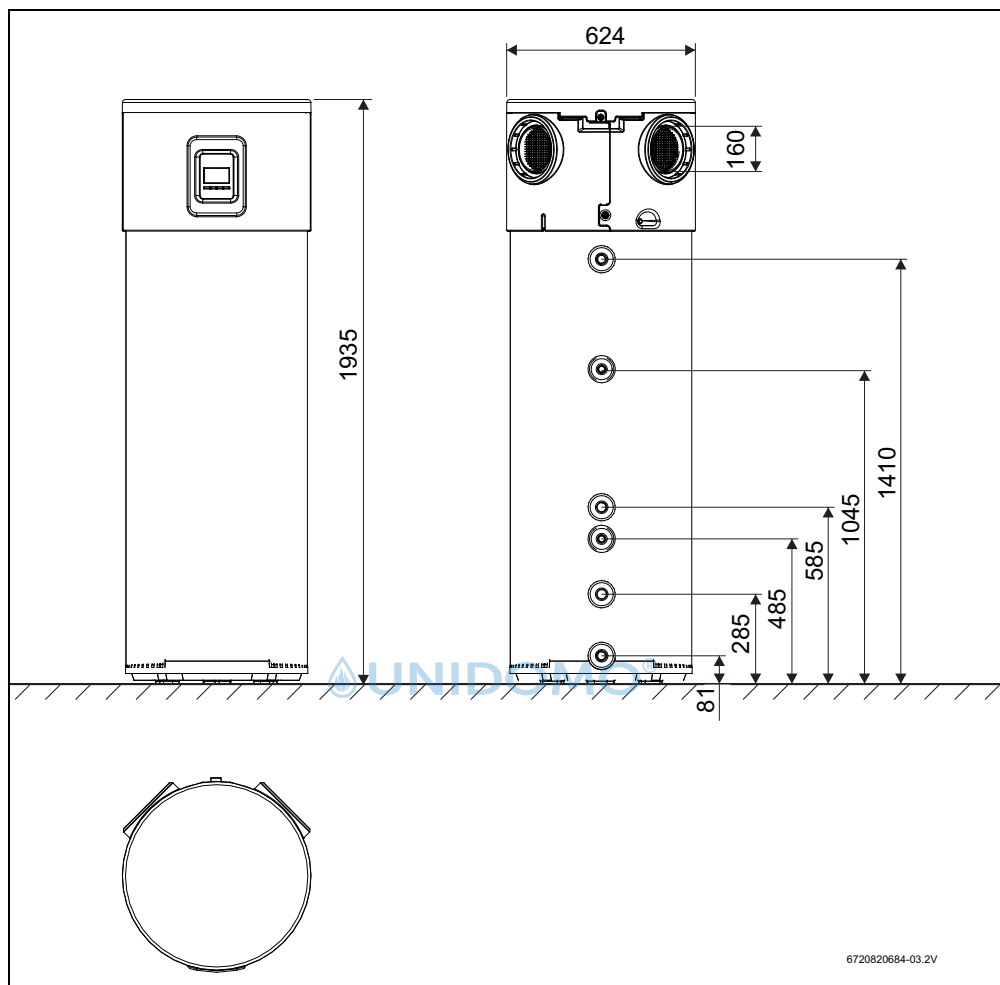
Bild 3 Abmessungen des 250 l-Gerätes (in mm)
