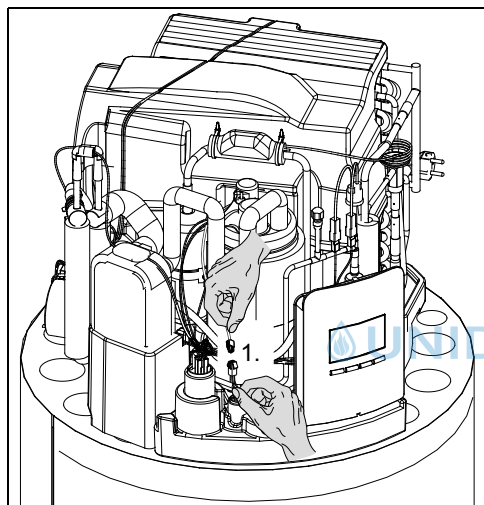
Bild 50 Gebläse-Anschlusskabel
