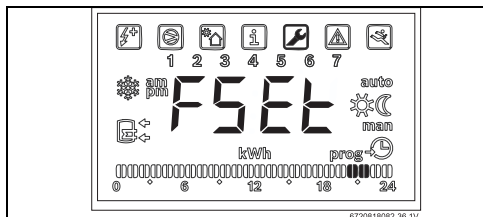
Bild 43 Funktion "Fset"
