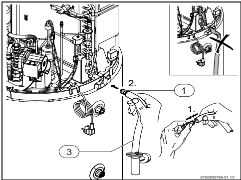
Bild 12 Kondensatauffang
