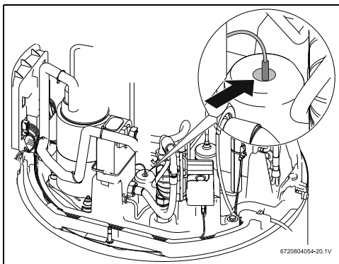
Bild 9 Warmwasser-Temperaturfühler im Speicher
