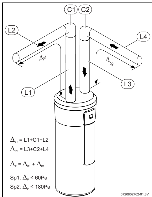
Bild 11 Druckverluste
