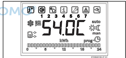
Bild 18 Betriebsart „manuell“
