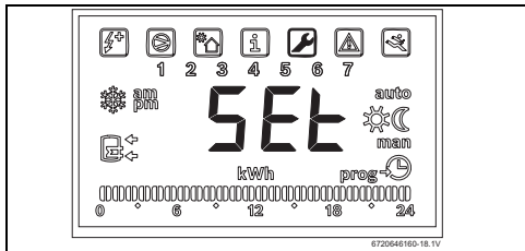
Bild 26 Funktion „Set“
