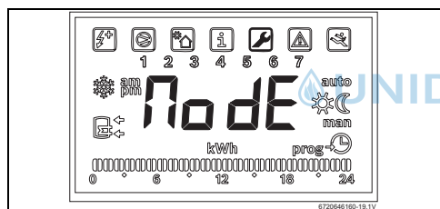
Bild 22 Funktion „Mode“
