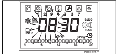
Bild 27 Datum einstellen
