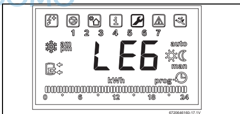
Bild 37 Funktion „Leg“
