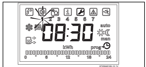
Bild 28 Wochentag einstellen
