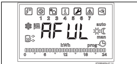
Bild 41 Funktion „Aful“
