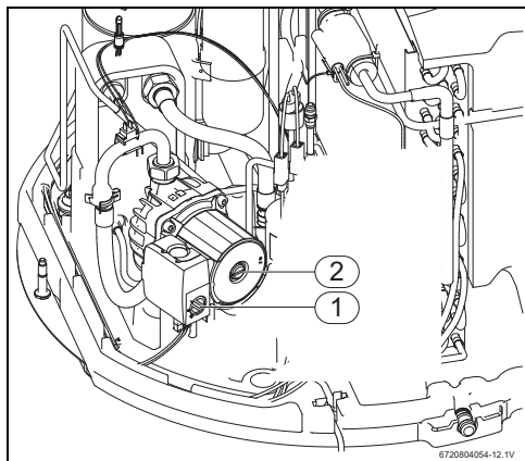
Bild 13 Umwälzpumpe
