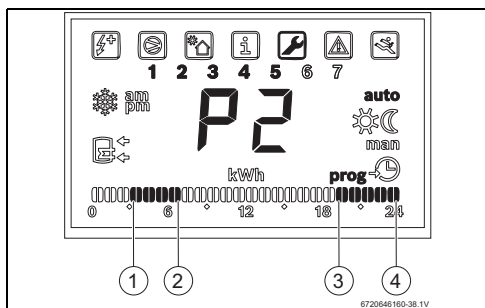
Bild 35 Betriebszeiten einstellen
