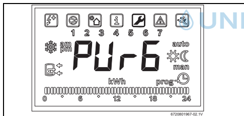
Bild 40 Funktion „Purg“
