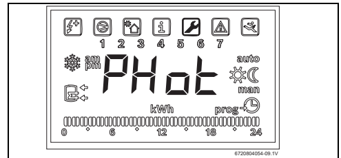
Bild 44 Funktion „Phot“
