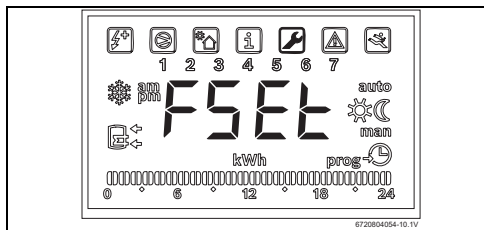
Bild 46 Funktion „Fset“
