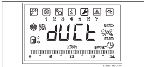
Bild 39 « Duct » funktion
