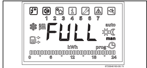
Bild 20 Betriebsart „Full“
