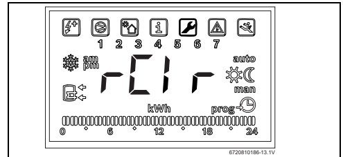
Bild 45 Funktion „Rcir“
