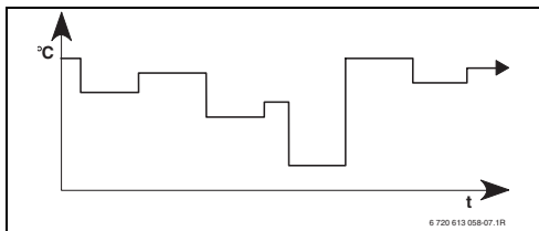
Bild 14 Beispiel Warmwasserprogramm mit Zeit-/Temperaturniveauprofil
