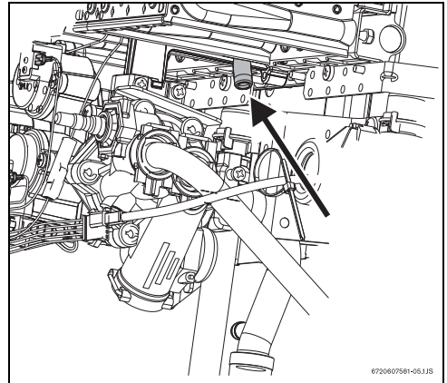
Bild 17 Messpunkt Düsendruck
