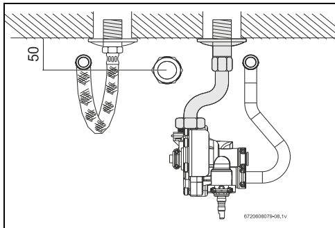
Bild 8 Unterputz-Installation
