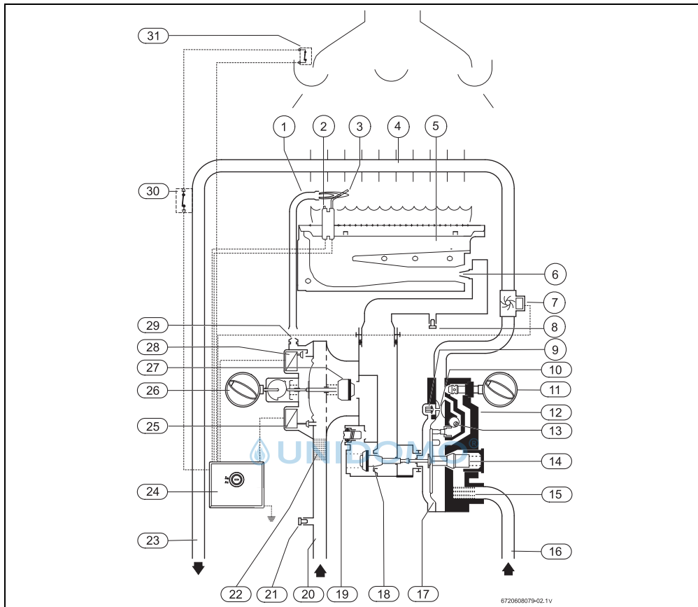
Bild 4 Funktionsschema
