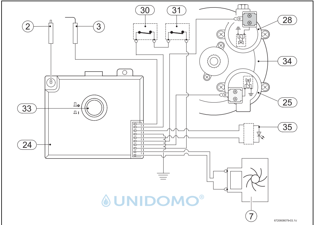
Bild 5 Elektrische Verdrahtung
