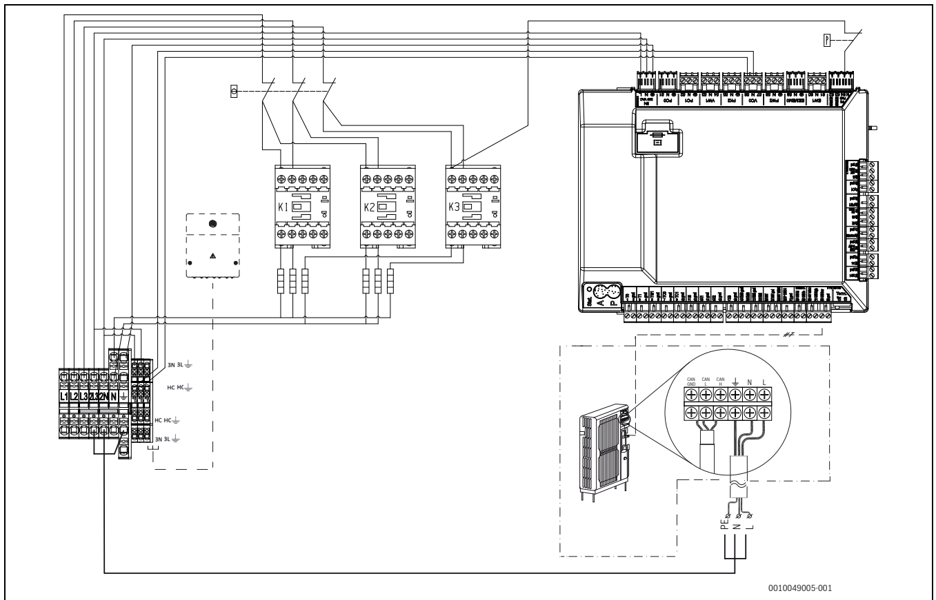
1 400V IDU - 230V ODU
