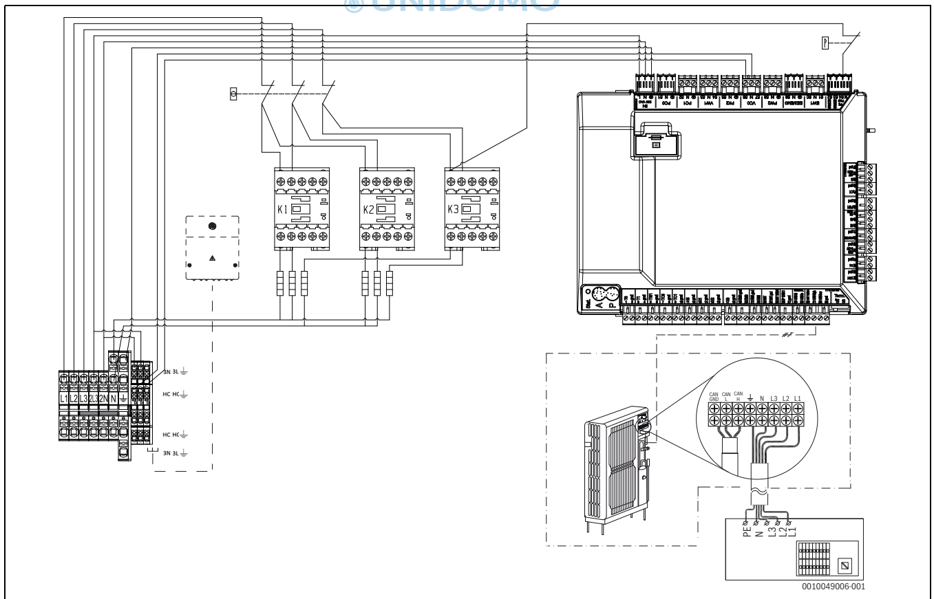
2 400V IDU - 400V ODU
