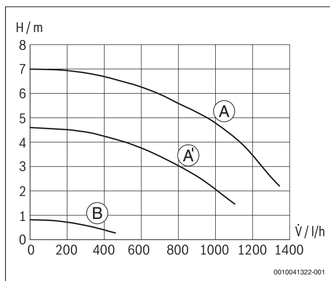
Bild 3 Pumpenkennfeld
