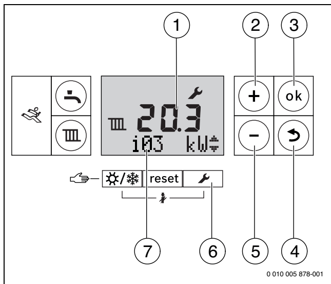
Bild 2 Übersicht der Bedienelemente
