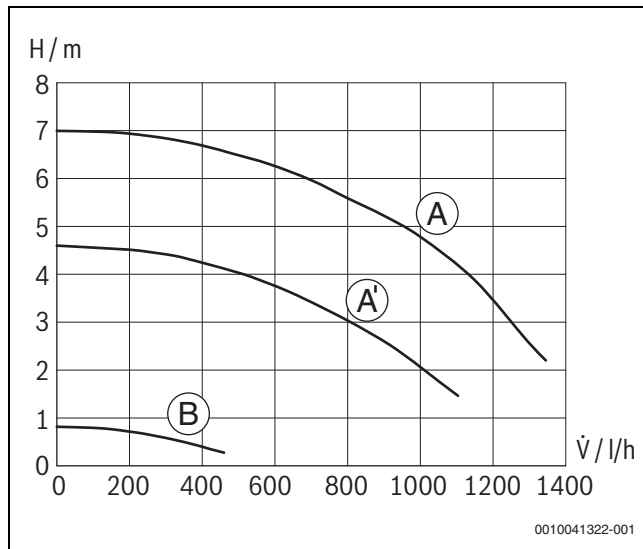
Bild 3 Pumpenkennfeld
