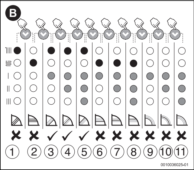
5 de: Pumpenkennlinie verändern (grüne und/oder gelbe LED) / en: changing pump curve (green and/or yellow LED) / nl: opvoer karakteristiek wijzigen
