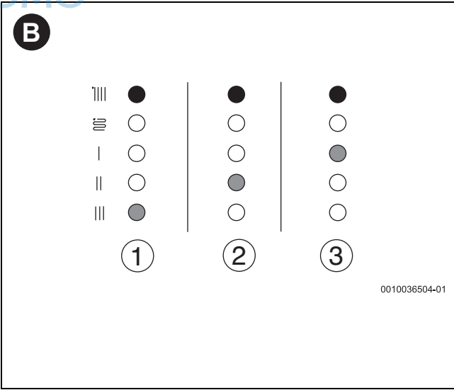
4 de: Störung (rote und gelbe LED) / en: fault (red and yellow LED) / nl: Storing (rote en geel LED) [1] de: Rotor blockiert / en: Rotor is blocked / nl: Rotor geblokkeerd [2] de: Netzspannung zu niedrig / en: supply voltage too low / nl: netspanning te laag [3] de: Störung der Elektronik / en: electrical error / nl: elektronika storing
