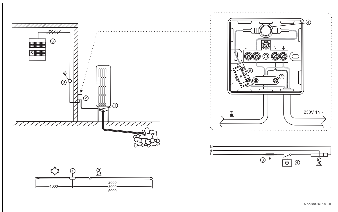
Рис. 73 Інструкції з підключення для теплового насоса з водяним контуром між внутрішнім і зовнішнім блоками
