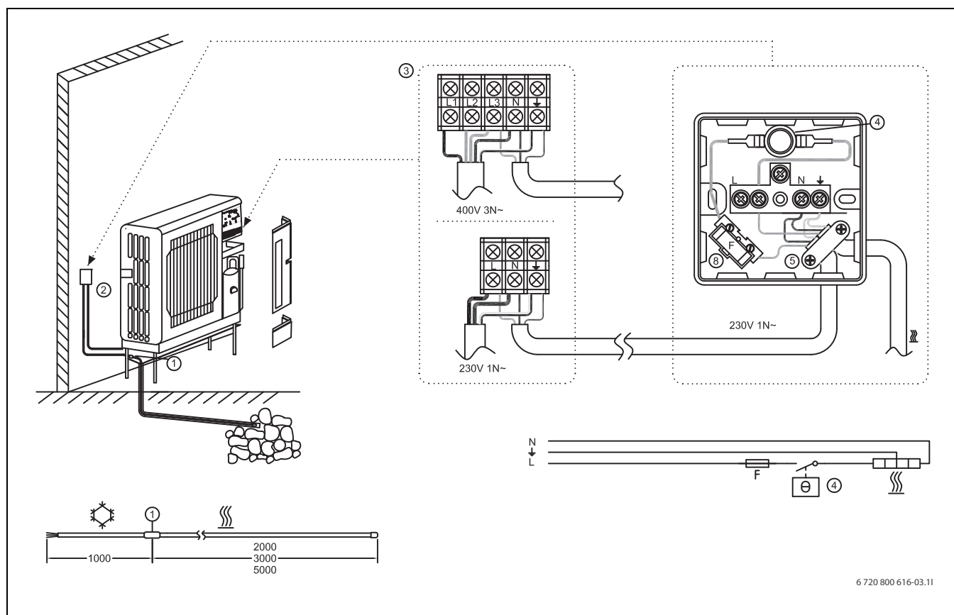
Fig. 45 Innkobleingsveiledning for varmpumpe med vannrør eller kuldemediabærende gjennomgangsrør mellom inne- og utedel
