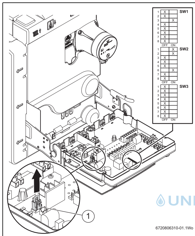
Afb. 1 DIP-schakelposities
