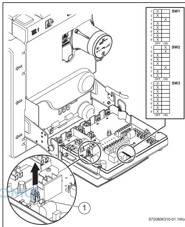
Fig. 1 Posições do interruptor DIP
