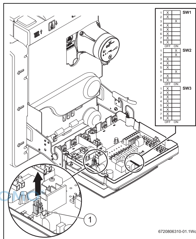
Fig. 1 Posiciones del interruptor DIP
