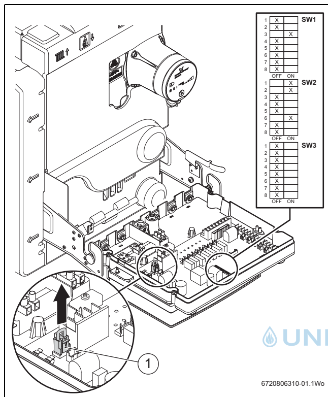
Bild 1 DIP-omkopplarpositioner
