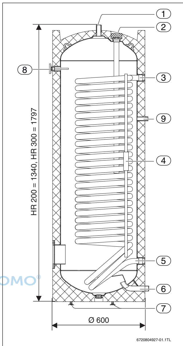
Sl. 14 Boiler za sanitarno vodo (mm)
