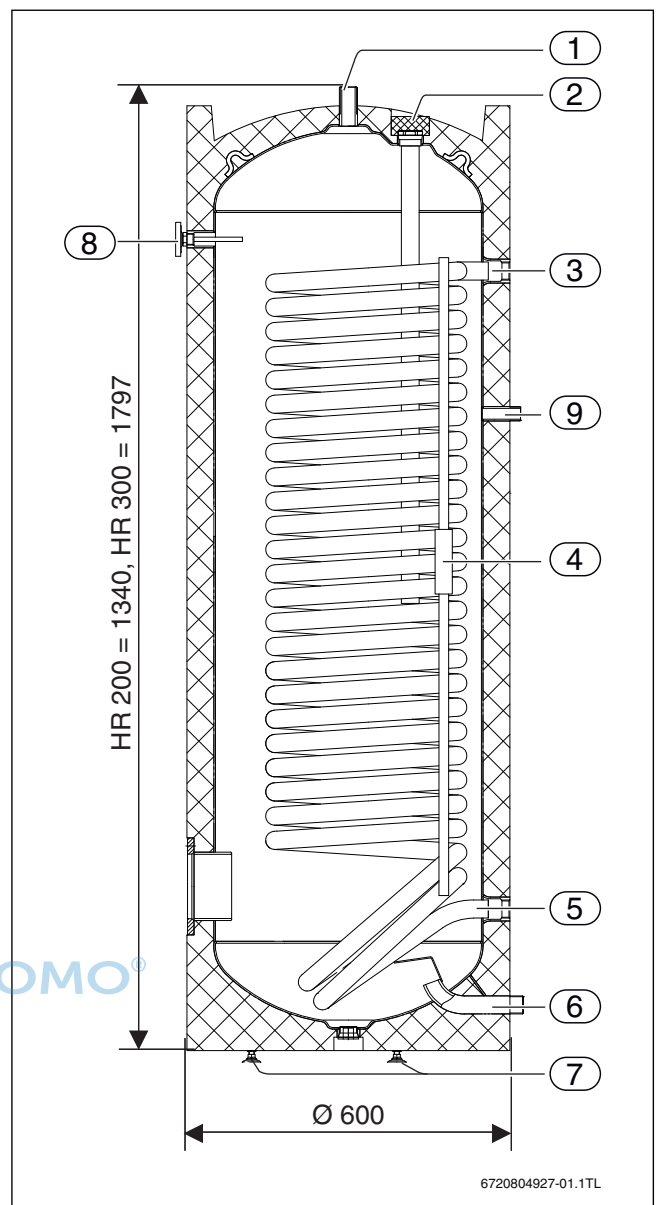
Obr. 15 Ohříváč teplé vody (mm)
