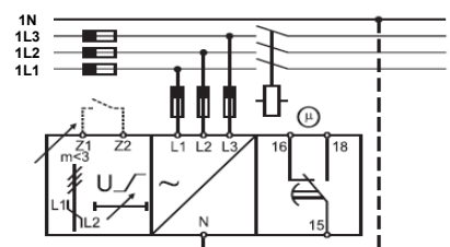
Schaltplan für den neuen Phasenwächter
