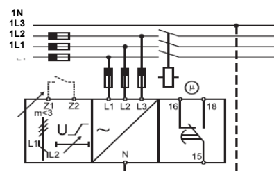
Схема соединений нового реле контроля фаз
