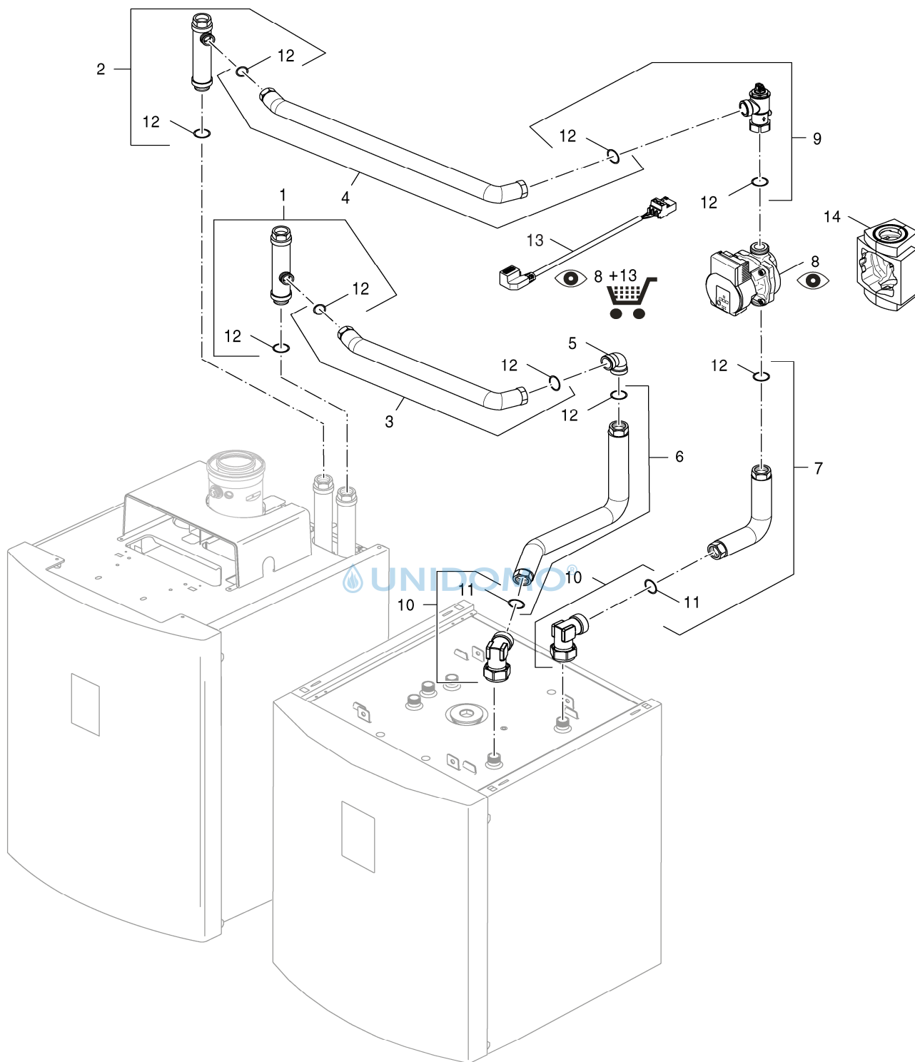
8738890515.ab.RS-Anschluss-Set Speicher nebeneinander
