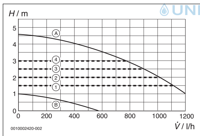
Bild 13 Pumpenkennfelder und Pumpenkennlinien für GC7000iW 14/24/28 (C)
