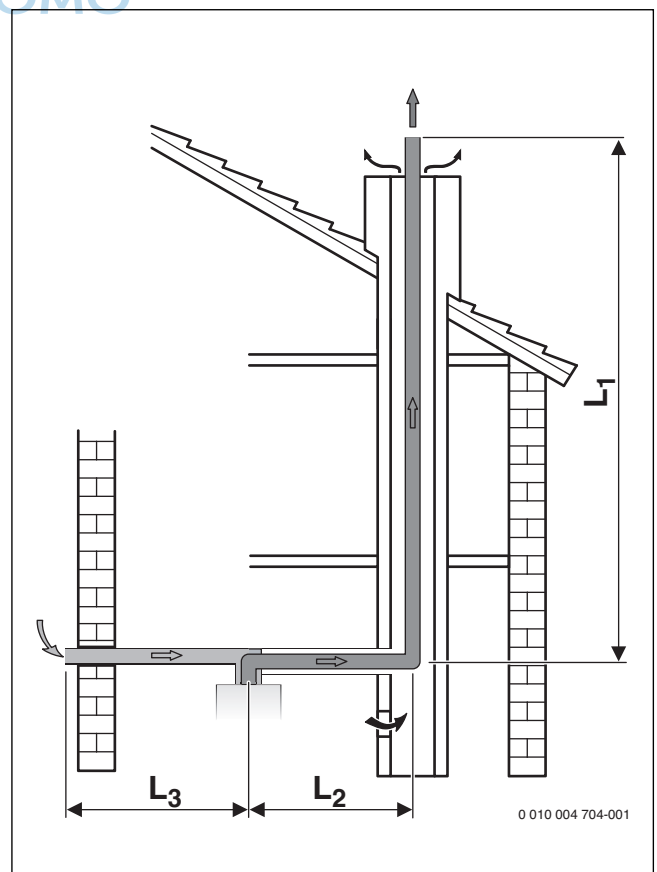
Bild 45 Abgasführung im Schacht nach C 53x
