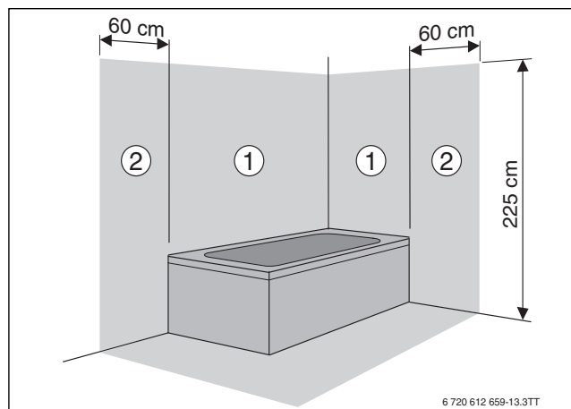
Bild 31 Schutzbereiche
