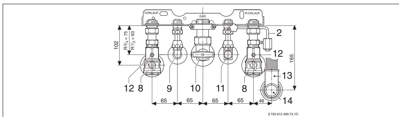
Bild 22 Montageanschlussplatte Zubehör Nr. 258 für Unterputzinstallation, fertig montiert mit Wartungshähnen (Zubehör)
