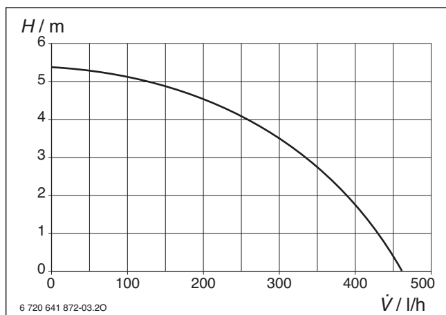
Bild 29 Hebepumpendiagramm
