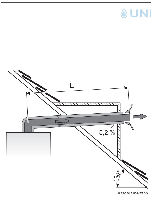
Bild 47 Abgasführung waagrecht nach C 13x
