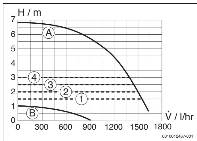
Bild 14 Pumpenkennfelder und Pumpenkennlinien für GC7000iW 35/42 (C)
