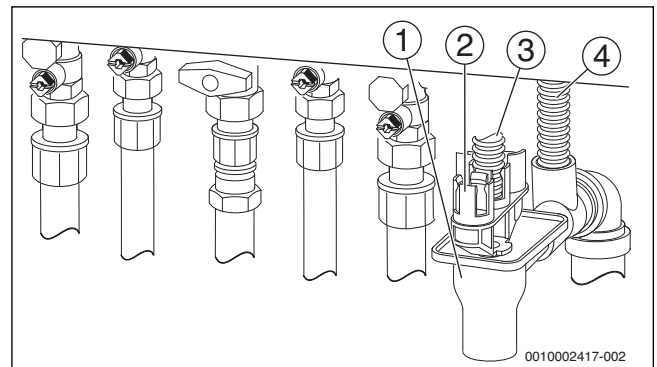
Bild 23 Siphon mit Tropfadapter (Zubehör Nr. 432)
