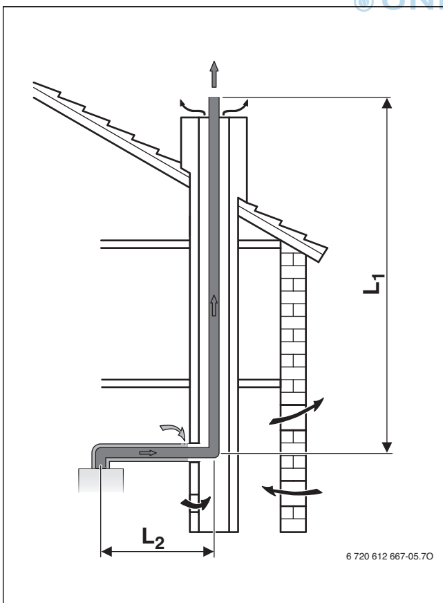
Bild 43 Abgasführung im Schacht nach B 33x
