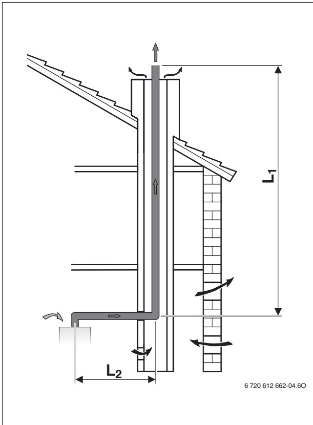
Bild 42 Abgasführung im Schacht nach B 23
