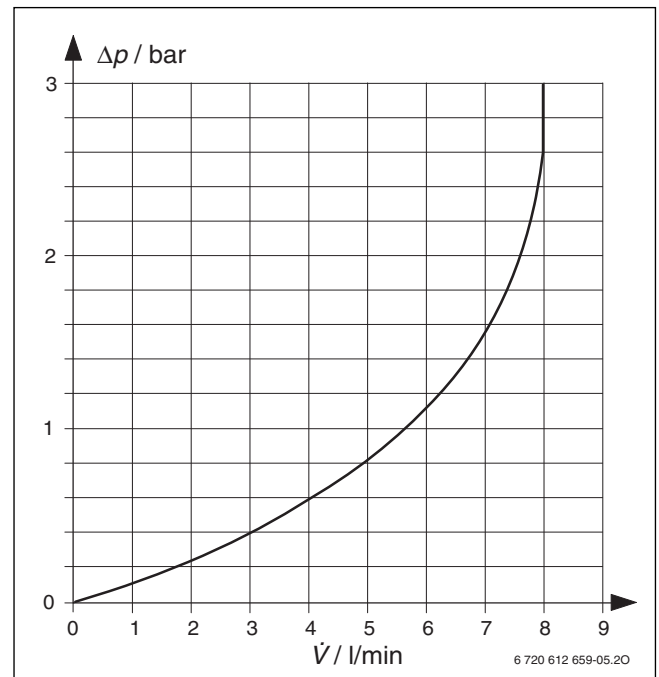
Bild 44 Druckverlustdiagramm Warmwasser
