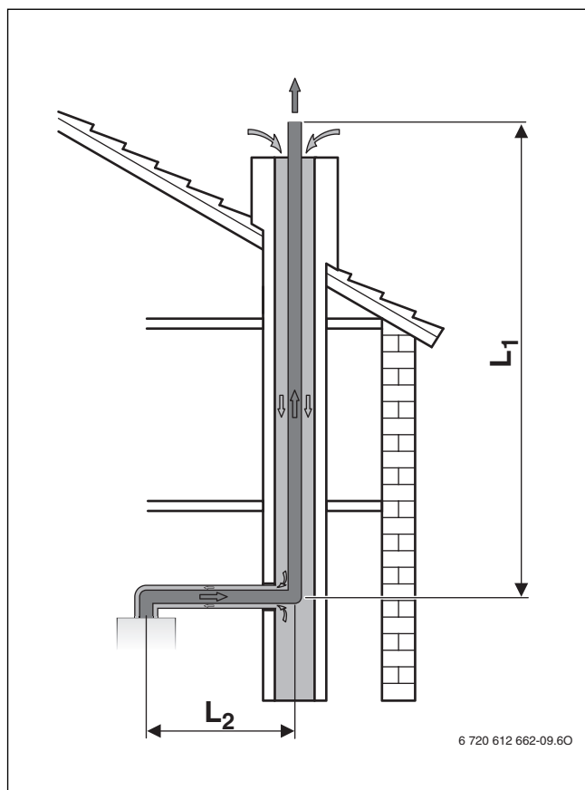
Bild 52 Abgasführung im Schacht nach C 93x
