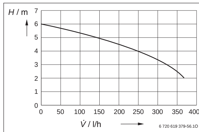
Bild 26 Restförderhöhe Nr. 1620
