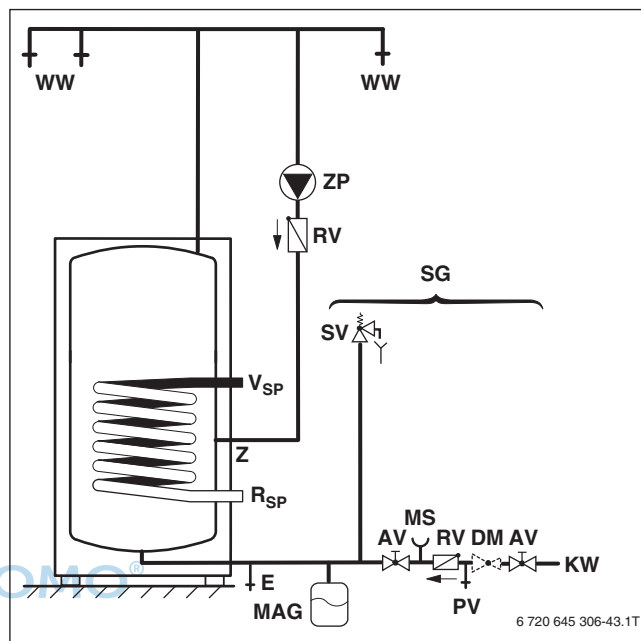
Bild 38 Warmwasserseitiges Anschluss-Schema
