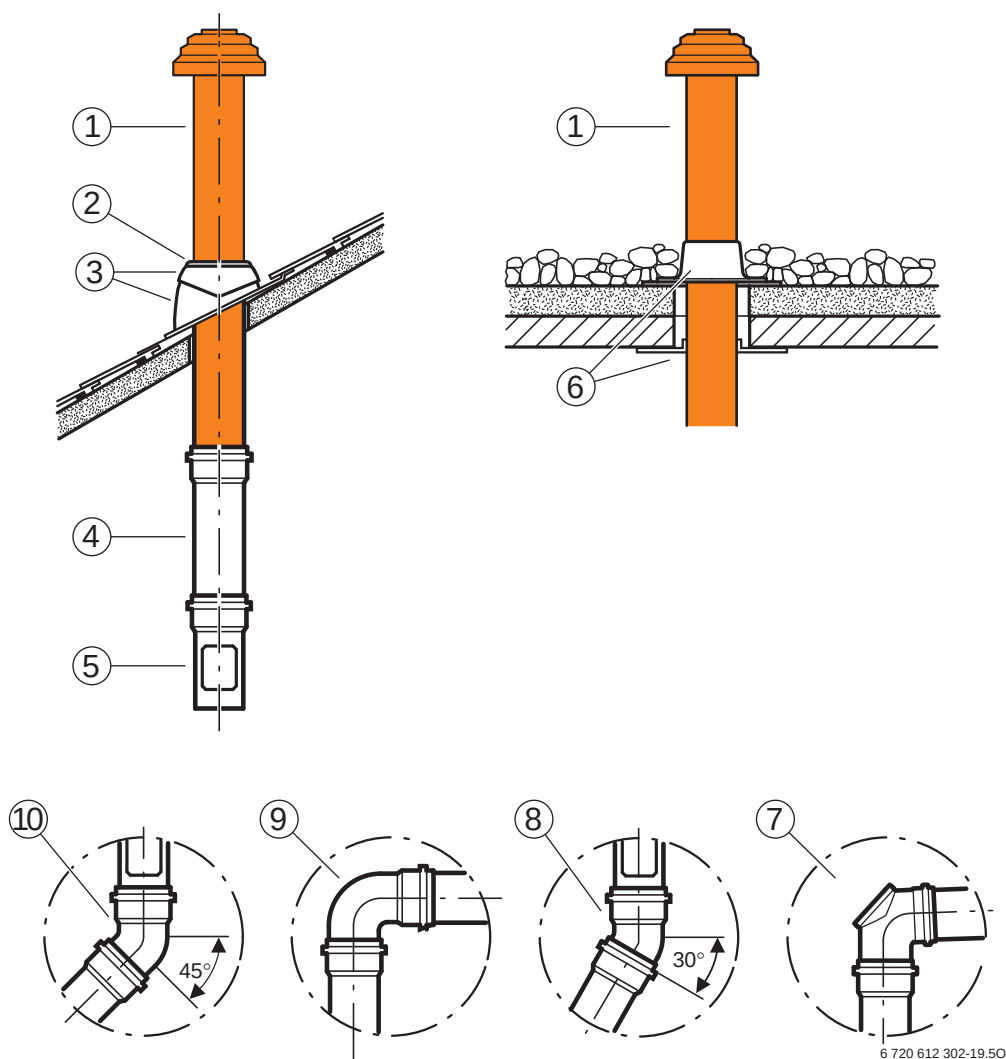
Bild 52 Abgasführung senkrecht Ø 80/125 mm über Dach (C 33x )
