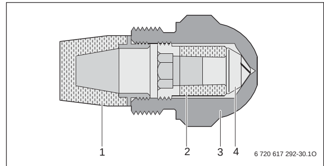
Bild 23 Öl-Druckzerstäuberdüse
