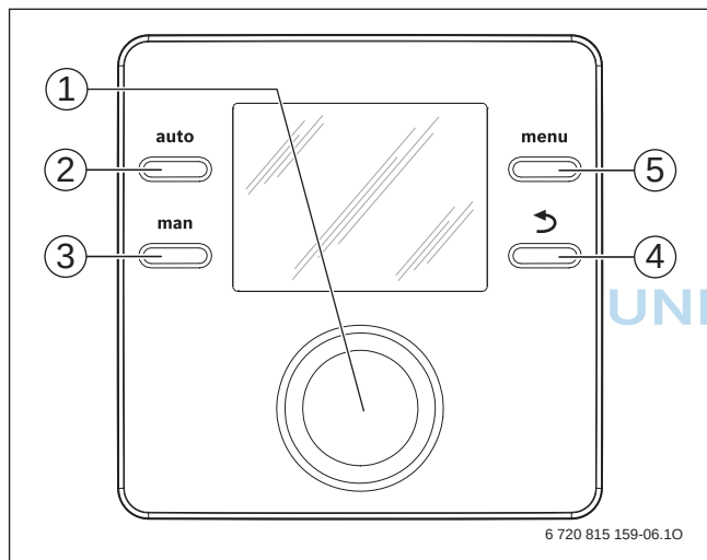
Bild 34 Bedienelemente CR 100
