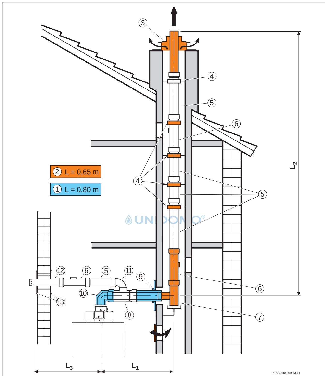
Bild 55 Abgasführung über Abgasleitung Ø 80 mm (C 53x )
