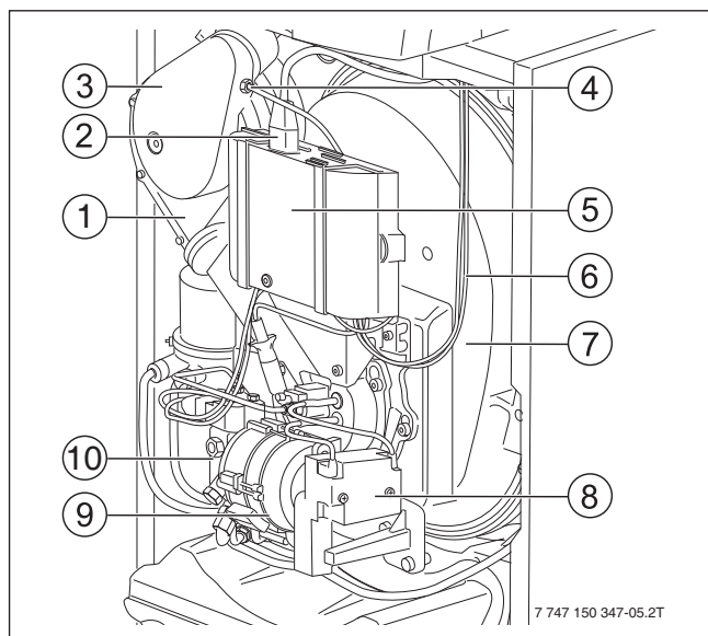
Bild 8 Ölbrenner
