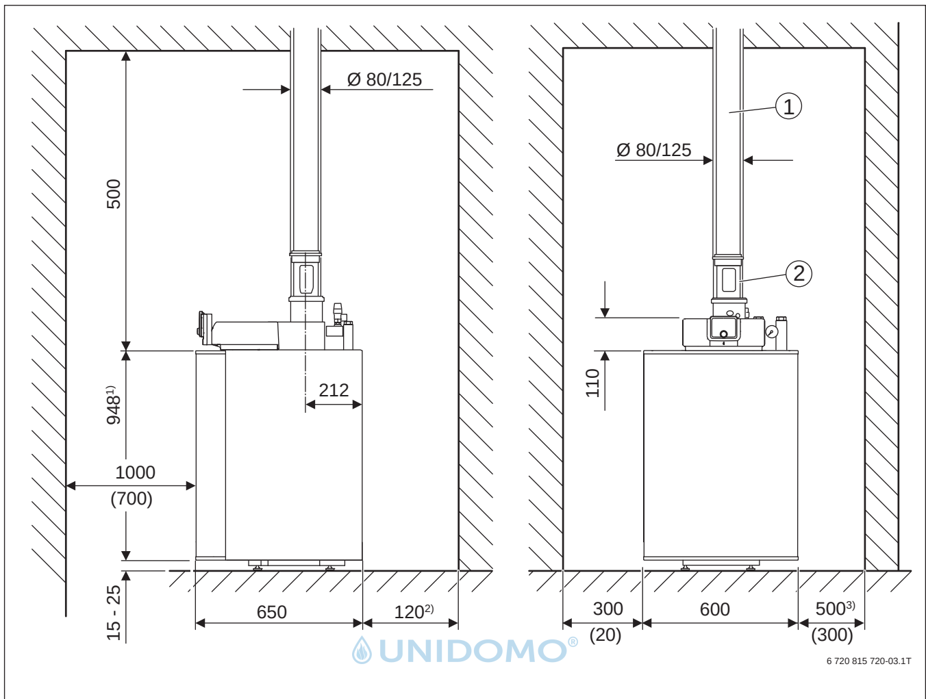
Bild 44 Einbaumaße bei senkrechter Abgasführung (die in Klammern angegebenen Werte sind Mindestmaße)
