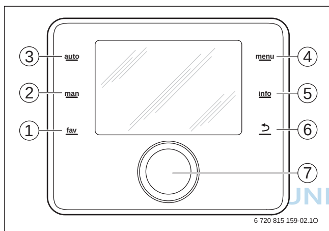
Bild 31 Bedienelemente
