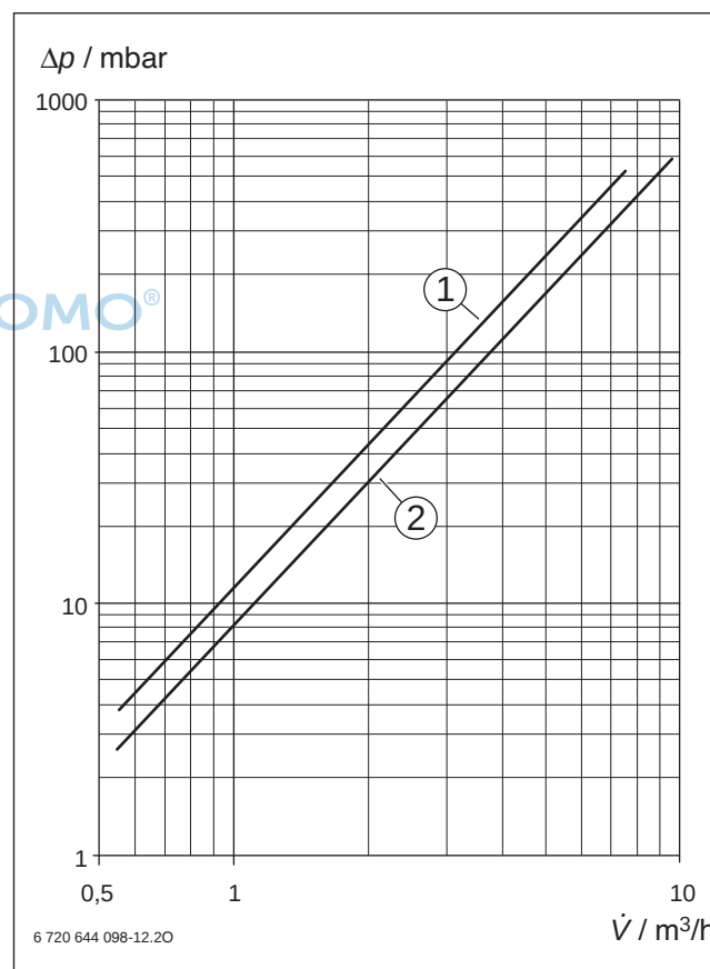
Bild 40 Druckverlust der Heizschlange
