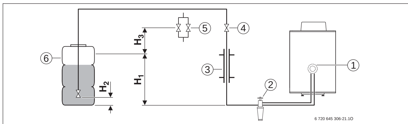
Bild 21 Installationsbeispiel
