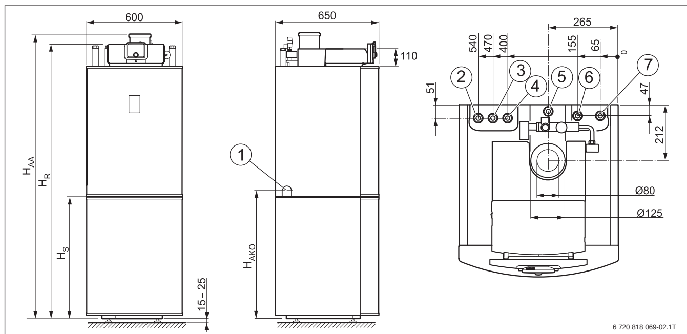
Bild 11 Anschlüsse und Abmessungen des Heizkessels mit optional untergestelltem Warmwasserspeicher (Maße in mm)
