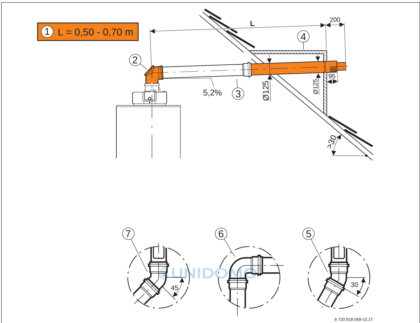
Bild 51 Abgasführung waagrecht Ø 80/125 mm über Dach (C 33x )
