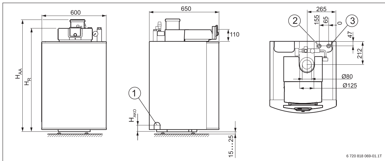
Bild 10 Anschlüsse und Abmessungen des Heizkessels (Maße in mm)
