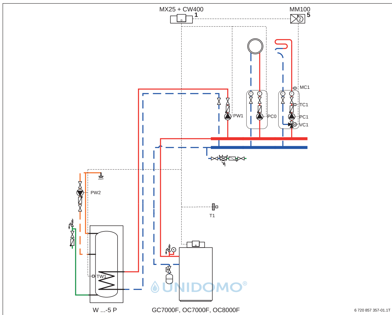
Bild 2 Anlagenschema (Abkürzungsverzeichnis → S. 6)
