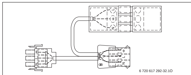
Bild 25 Adapterkabel, Nr. 1637
