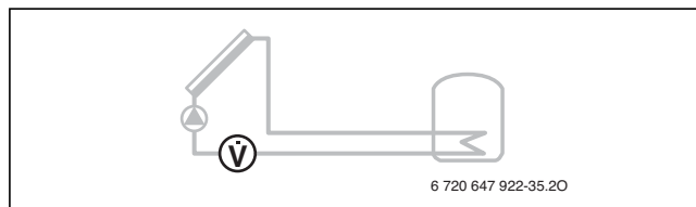
Bild 155 Wärmemengenzählung(L) Durch Auswahl des Wärmemengenzählers kann die Ertragsermittlung eingeschaltet werden.
