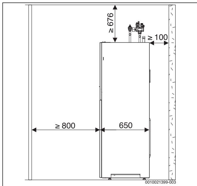
Bild 114 Mindestabstand Inneneinheit
