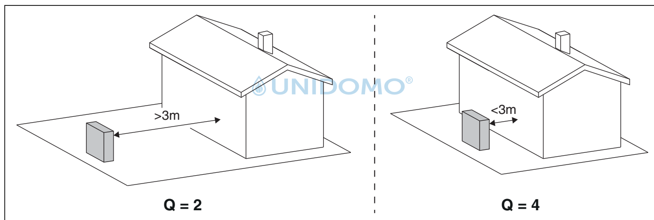
Bild 59 Abstand zu Wänden
