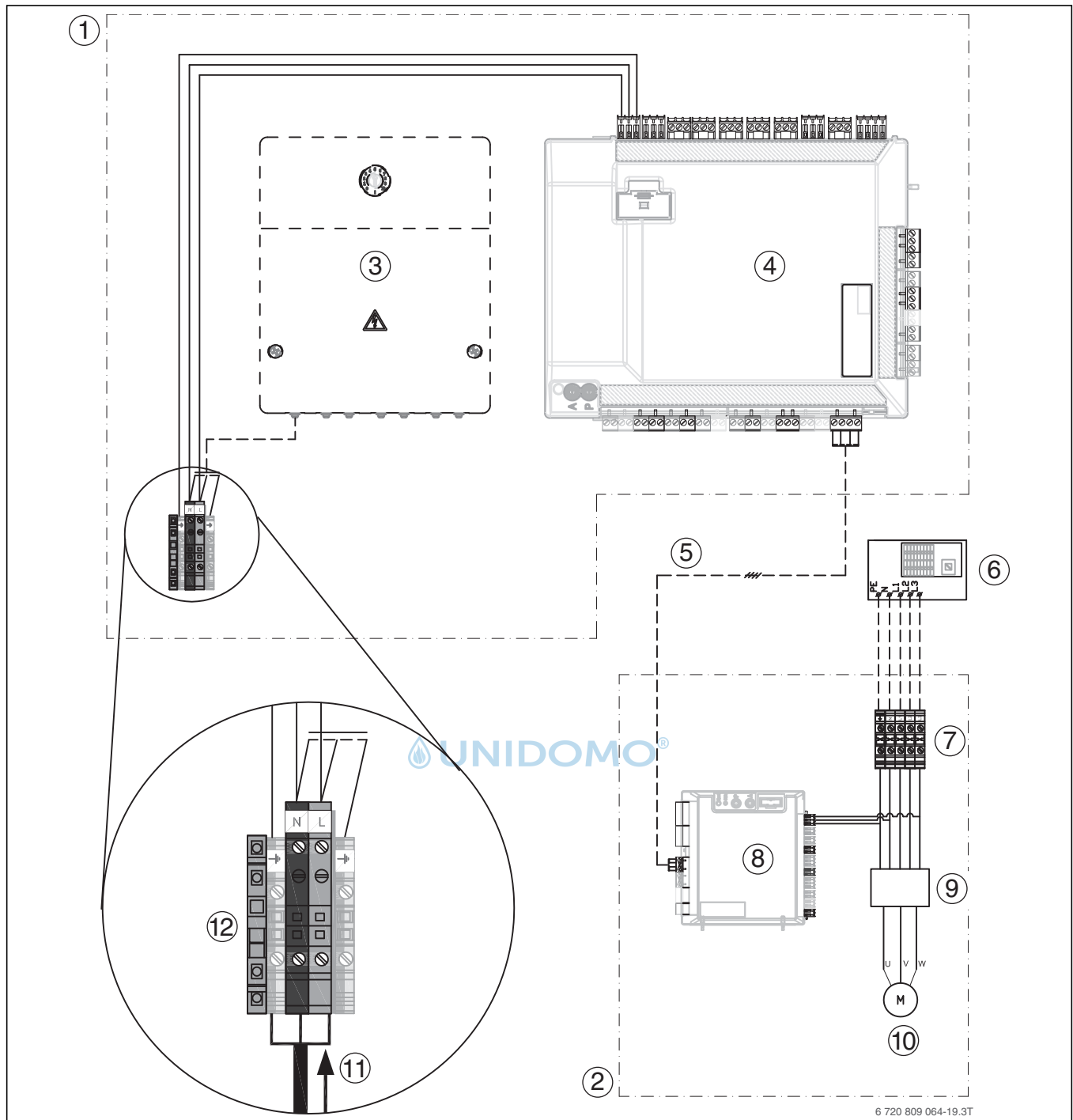
Bild 134 Wärmepumpen-Inneneinheit mit externem Zuheizter – Überblick
