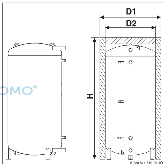
Bild 188 Maße BH ...-6
