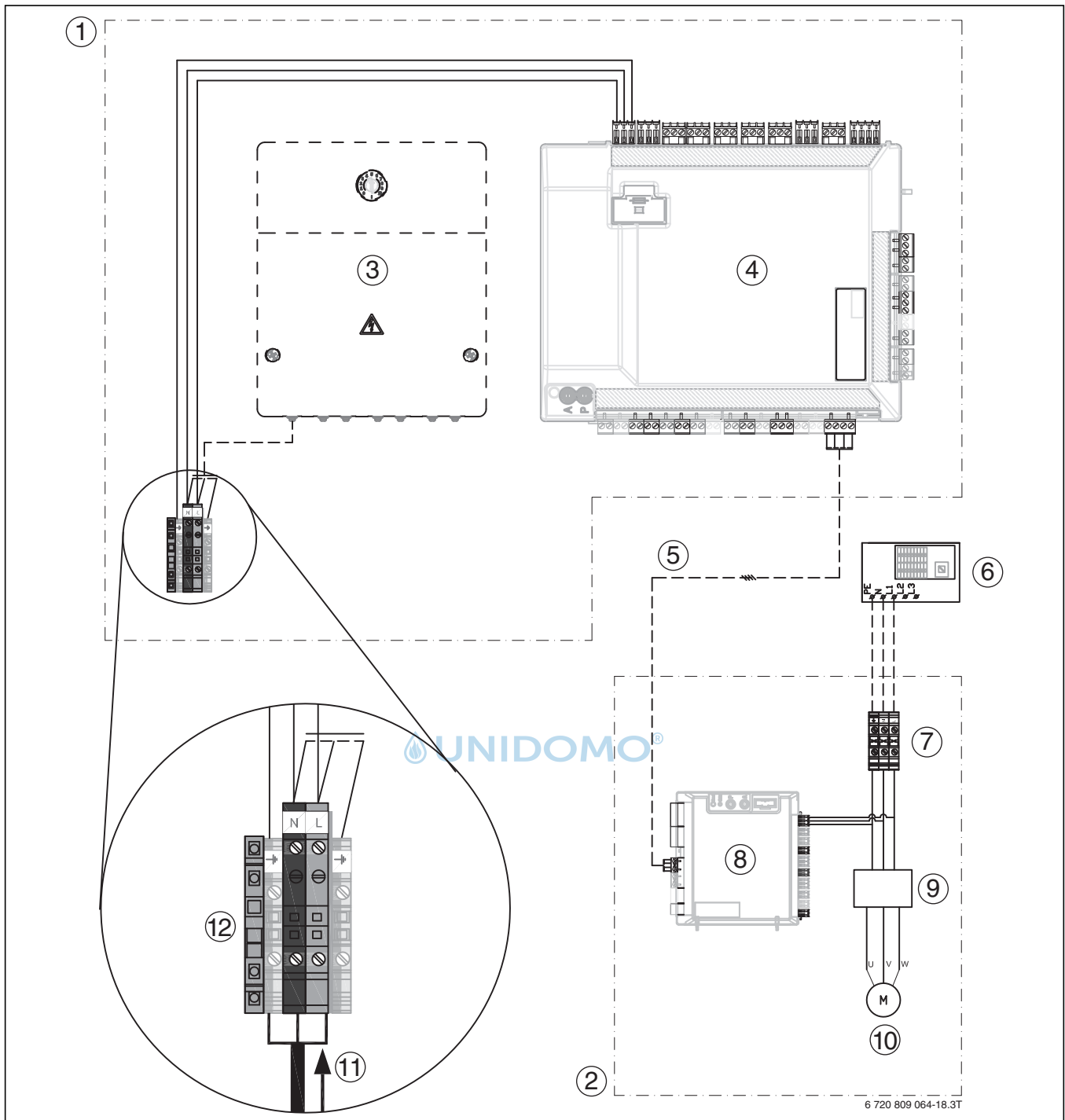
Bild 133 Wärmepumpen-Inneneinheit mit externem Zuheizter – Überblick
