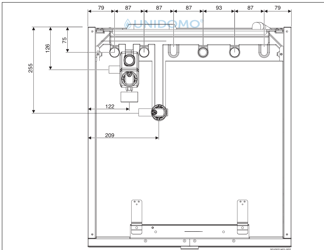
Bild 116 Abmessungen – Draufsicht
