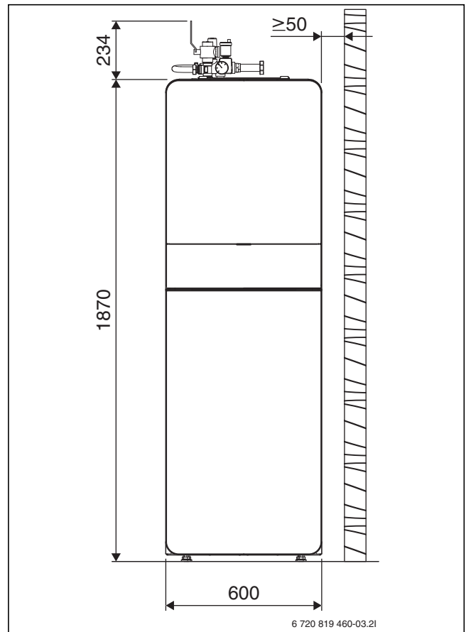
Bild 109 Mindestabstände Inneneinheit AWM 9/17, AWMS 9/17 (Ansicht von vorn)
