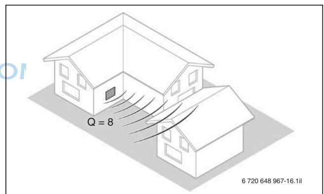
Bild 58 Wärmepumpe oder Lufteinlass/Luftauslass (bei Innenaufstellung) an einer Hauswand bei einspringender Fassadenecke, Abstrahlung in den Achtelraum ( Q = 8 ); Bildquelle: „Leitfaden Schall“ des bwp e.V.
