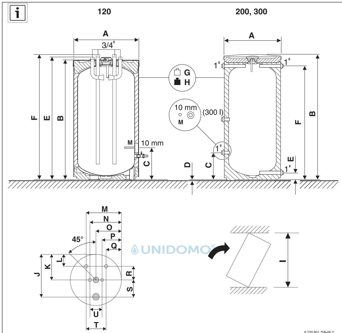
Bild 185 Abmessungen BH ...-5
