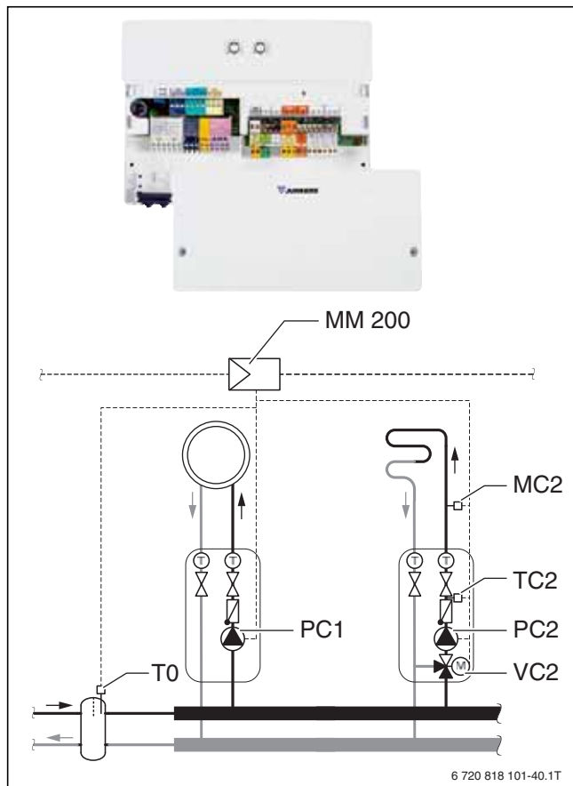
Bild 148 Heizkreismodul MM 200
