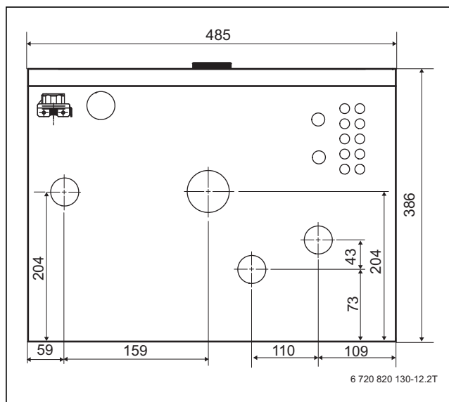
Bild 102 Abmessungen der Rohranschlüsse Inneneinheit AWE (Ansicht von unten)
