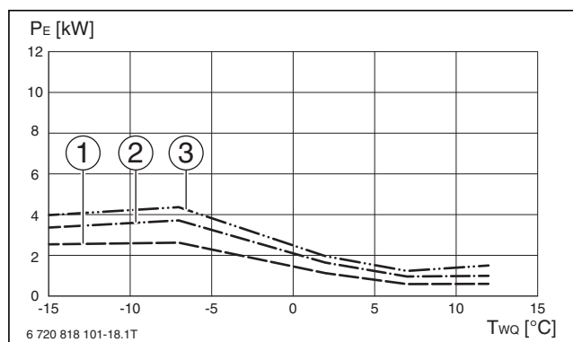
Bild 87 Leistungsaufnahme ( P_E ) CS7000iAW 13 OR-T
