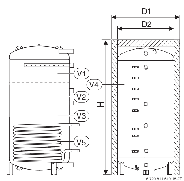
Bild 191 Maße und Volumina BHS 750/1000 ERZ B
