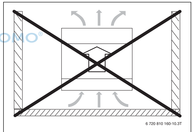
Bild 46 Von Wänden umgebene Aufstellung vermeiden
