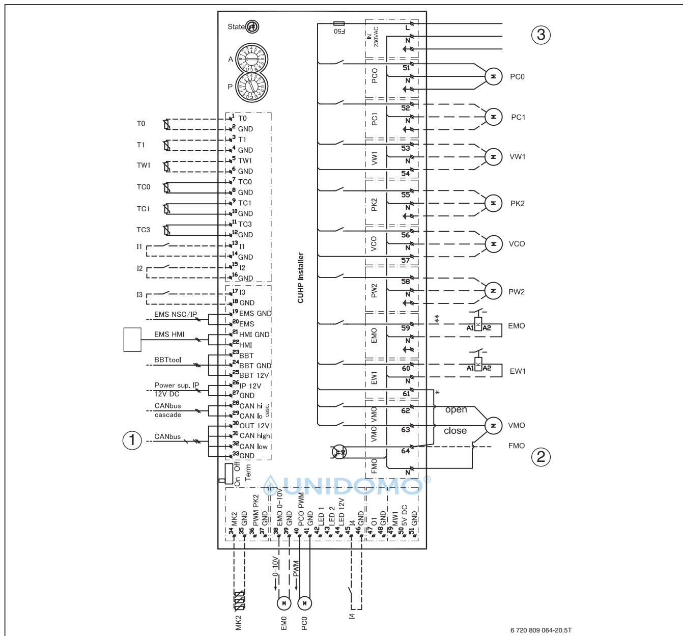
Bild 136 Schaltplan Installationsmodul
