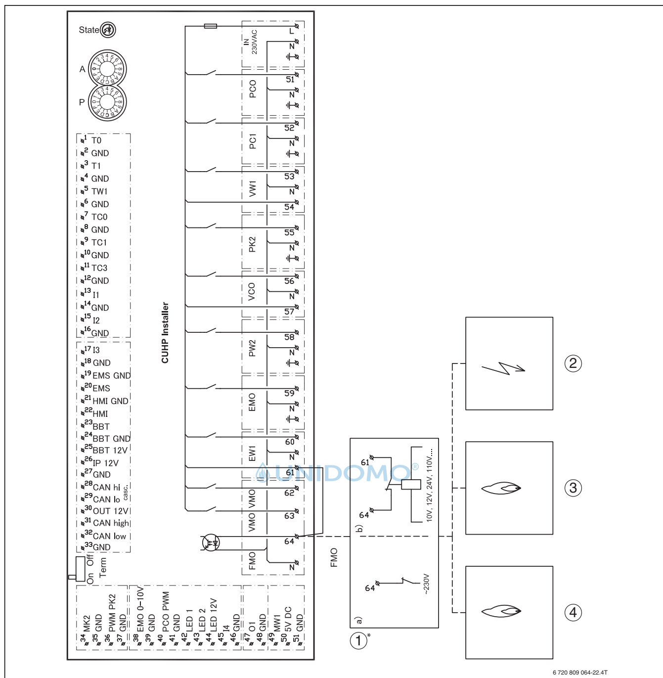
Bild 145 Schaltplan Installationsmodul, Alarm des Heizkessels
