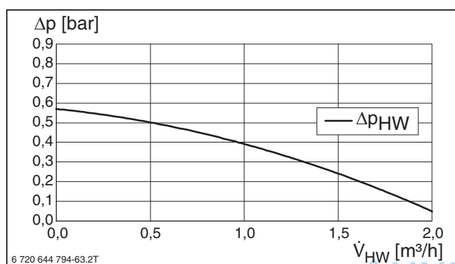
Bild 85 Restförderhöhe CS7001iAW 9 OR-S
