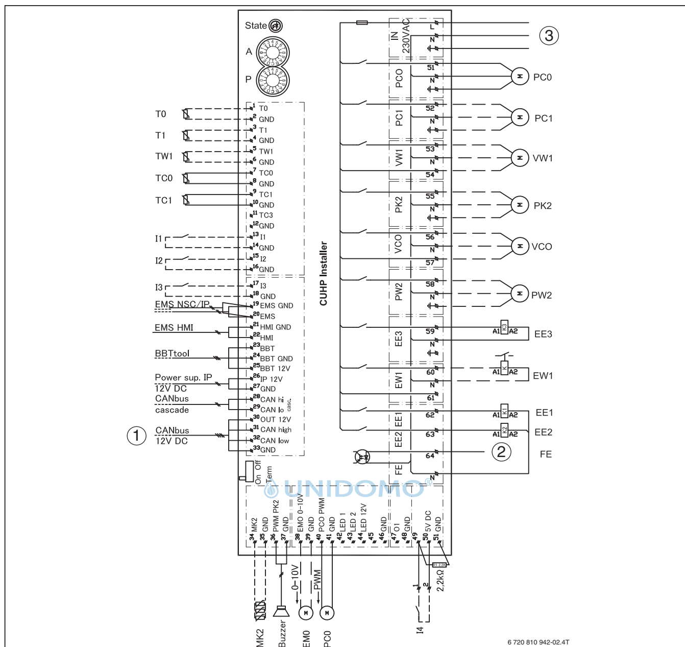
Bild 135 Schaltplan Installationsmodul integrierter elektrischer Zuheiz
