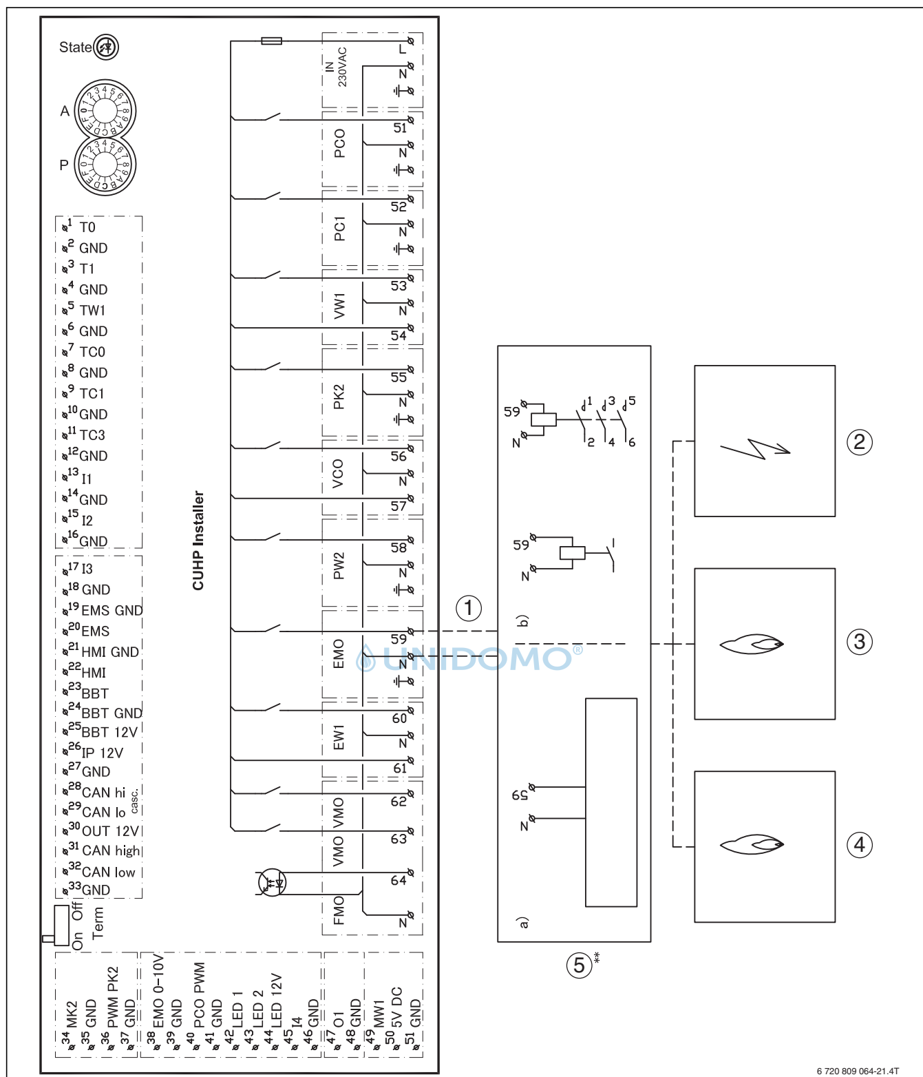
Bild 137 Schaltplan Installationsmodul, Start/Stopp
