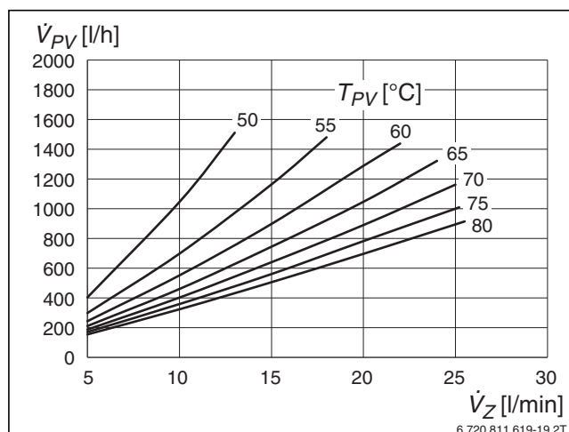
Bild 197 Volumenstrom vom Pufferspeicher (Vorlauf) bei 60 °C Zapftemperatur
