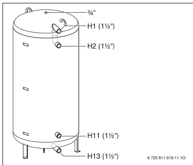
Bild 187 Anschlüsse BH ...-6
