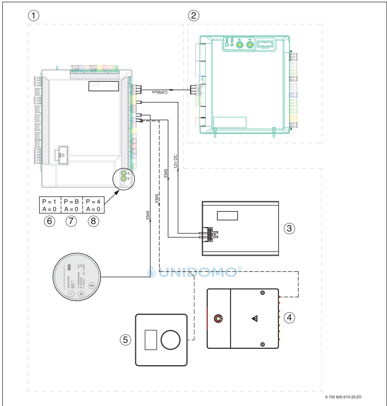
Bild 125 CAN-BUS und EMS – Überblick Inneneinheiten AWE/AWM/AWMS/AWMB mit elektrischem Zuheizer
