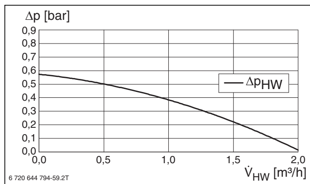
Bild 77 Restförderhöhe CS7001iAW 5 OR-S
