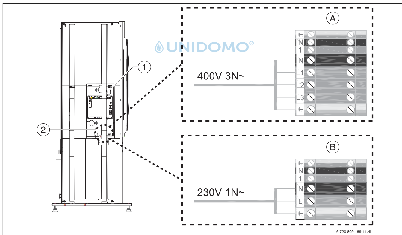
Bild 129 Kabelkanäle am Klemmenkasten der Wärmepumpe CS7000iAW .. OR
