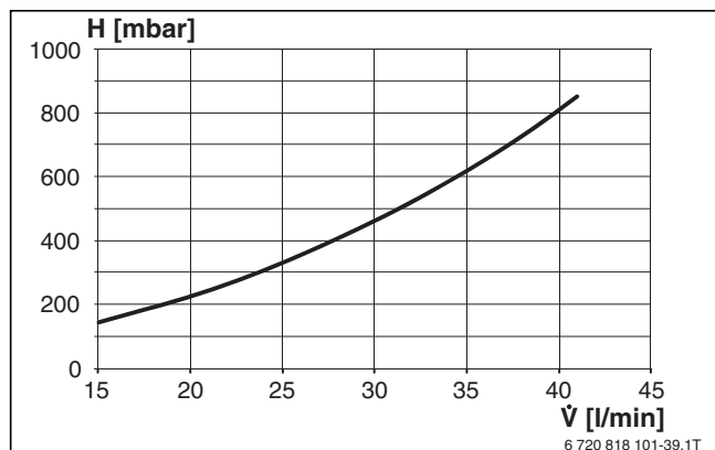
Bild 202 Druckverlust Sekundärseite
