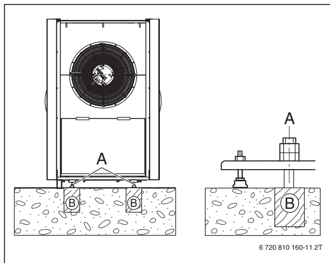
Bild 47 Bedingungen für den Untergrund
