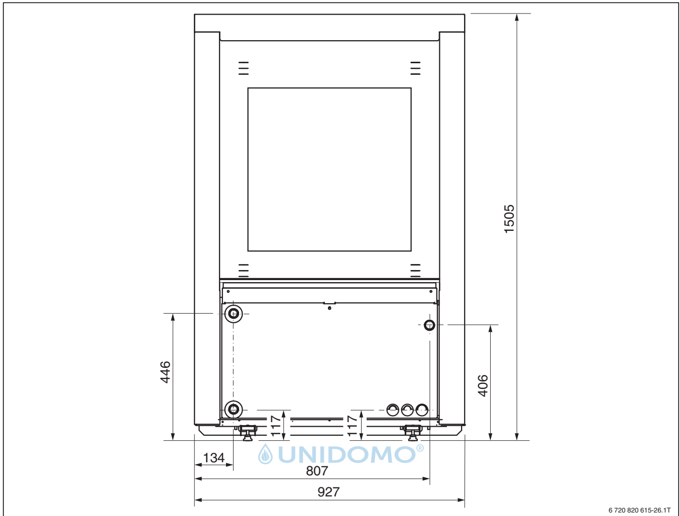
Bild 63 Abmessungen und Anschlüsse CS7000iAW 7/9 IR-S, Rückseite (Maße in mm)
