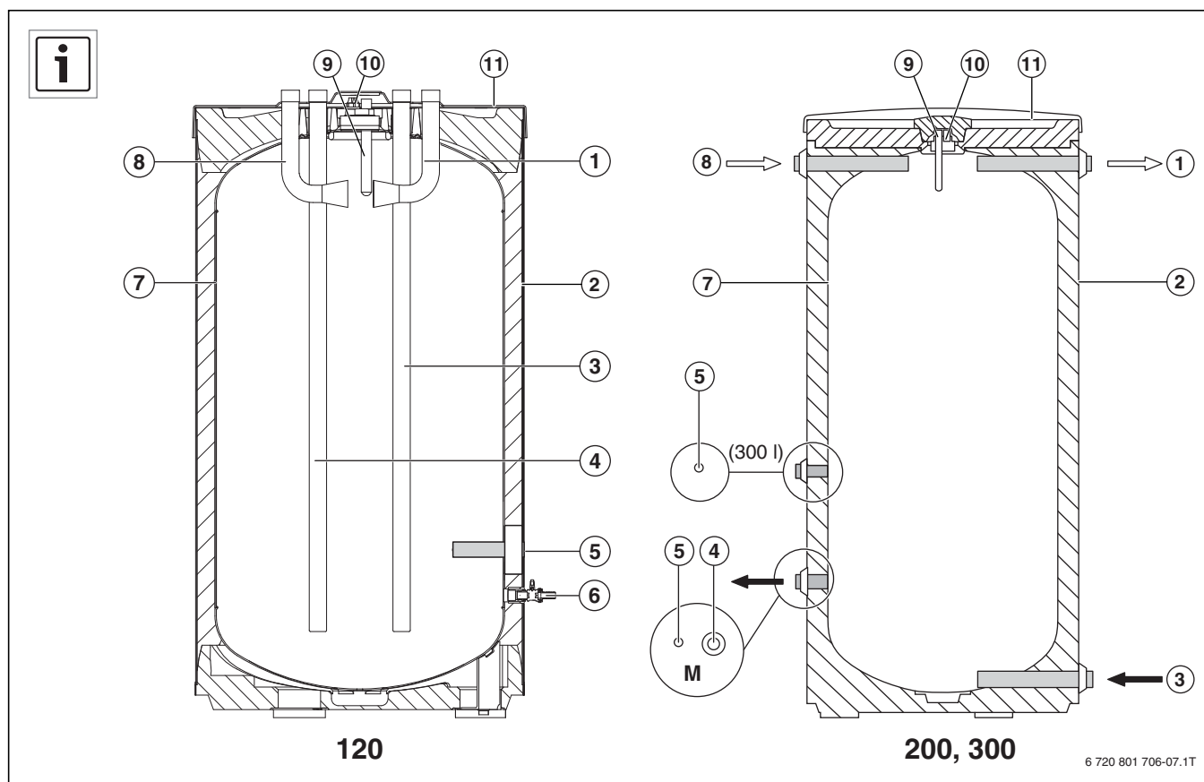
Bild 184 Übersicht BH ...-5
