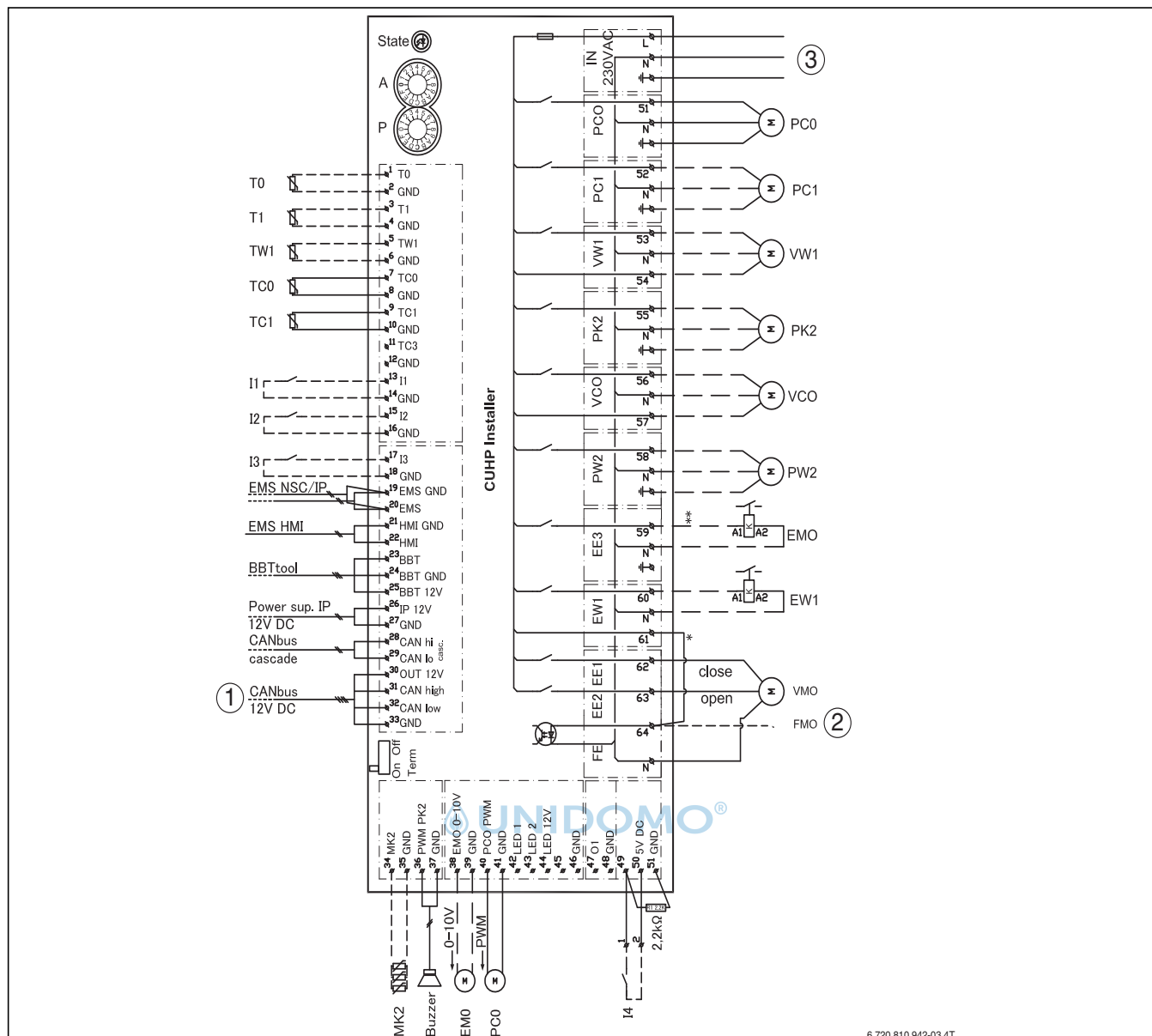
Bild 143 Schaltplan Installationsmodul
