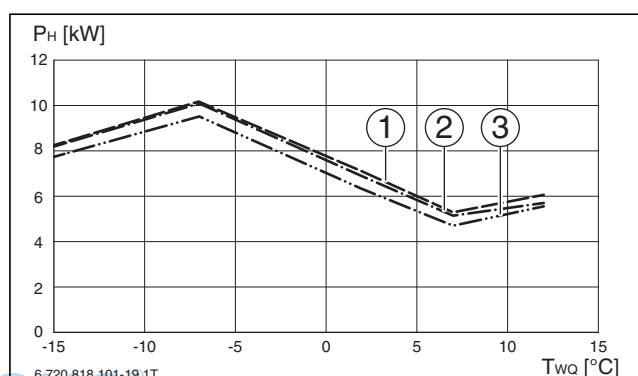
Bild 88 Heizleistung ( P_H ) CS7000iAW 13 OR-T
