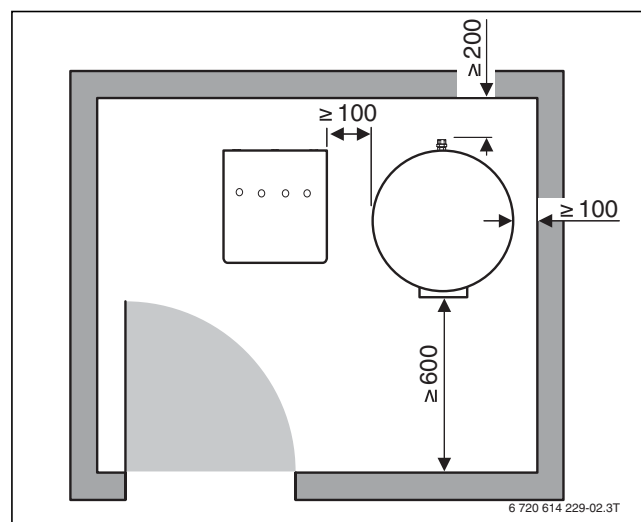
Bild 178 Empfohlene Mindest-Wandabstandsmaße in mm
