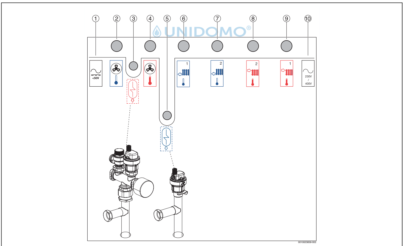
Bild 118 Anschlüsse der Inneneinheit mit zwei Heizkreisen (1 gemischter, 1 ungemischter)
