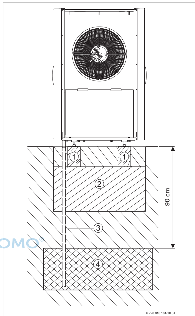
Bild 48 Kondensatablauf in Kiesbett
