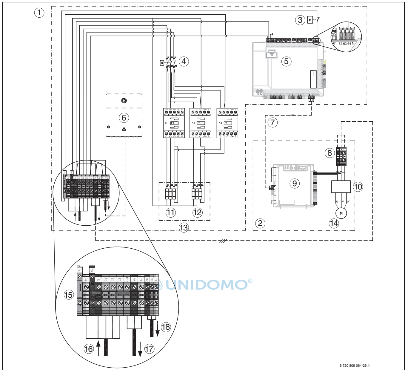
Bild 130 1-phasige Wärmepumpe CS7001iAW 5/7//9 OR-S und 3-phasiger integrierter elektrischer Zuheizer
