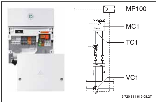
Bild 173 Schwimmbadmodul MP 100
