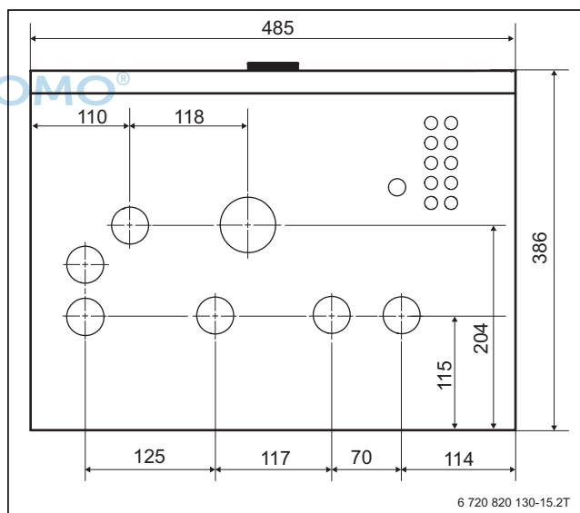
Bild 103 Abmessungen der Rohranschlüsse Inneneinheit AWB (Ansicht von unten)
