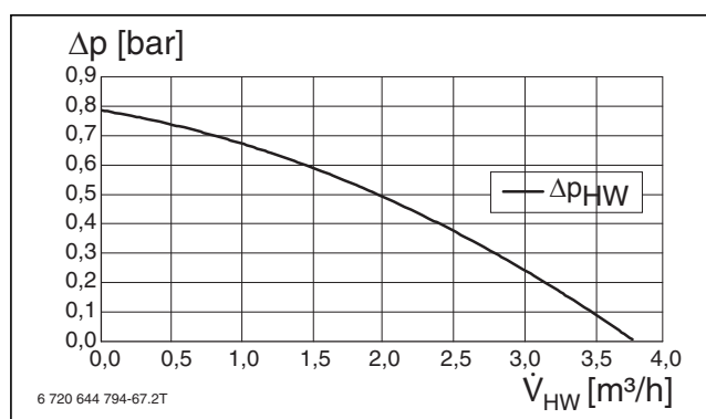
Bild 89 Restförderhöhe CS7000iAW 13 OR-T
