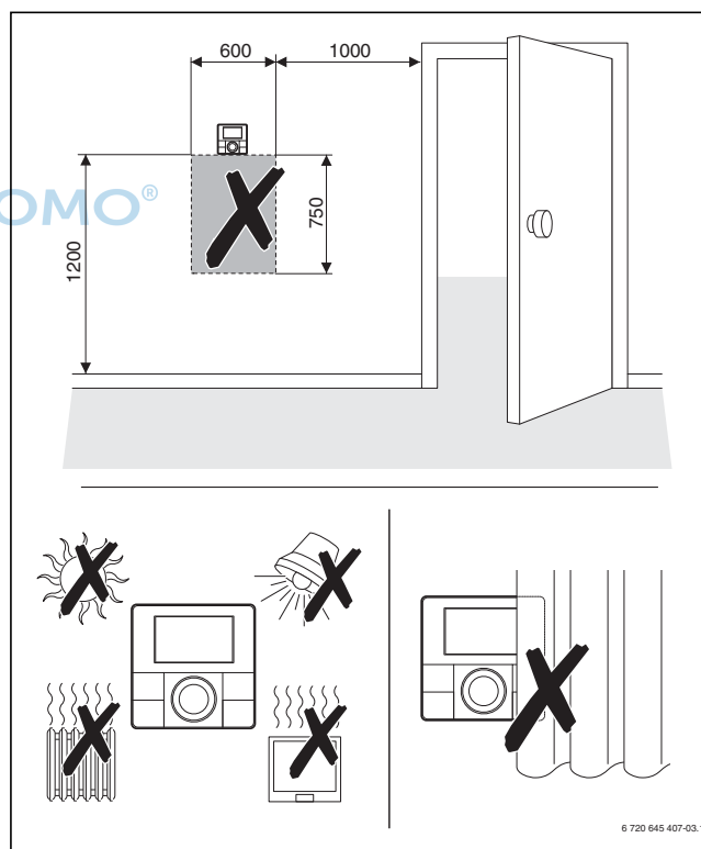
Bild 121 Position der Fernbedienung CR 10/CR 10 H im Referenzraum (Maße in mm)
