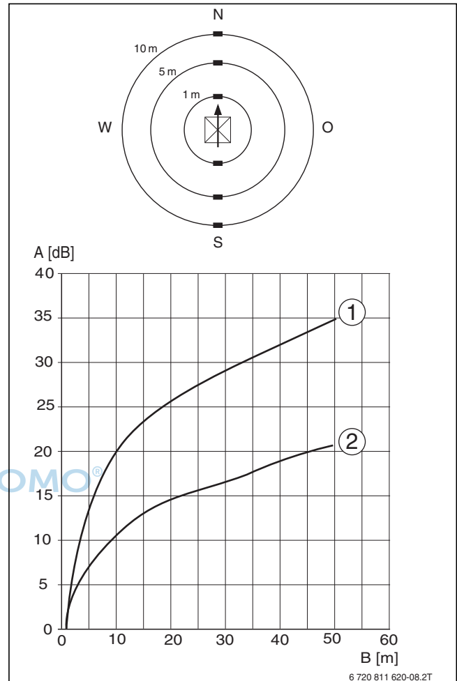
Bild 55 Schalldruckpegel-Abnahme in zunehmendem Abstand zur Wärmepumpe
