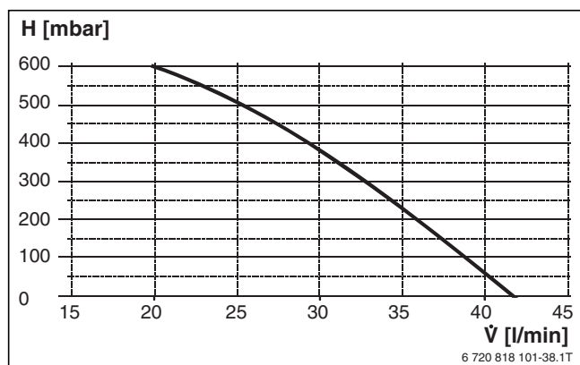
Bild 201 Restförderdruck Primärseite
