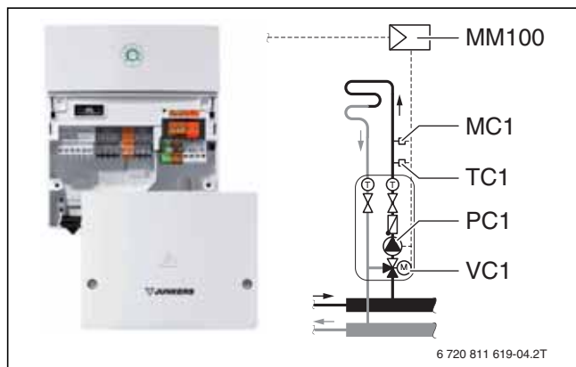
Bild 146 Heizkreismodul MM 100
