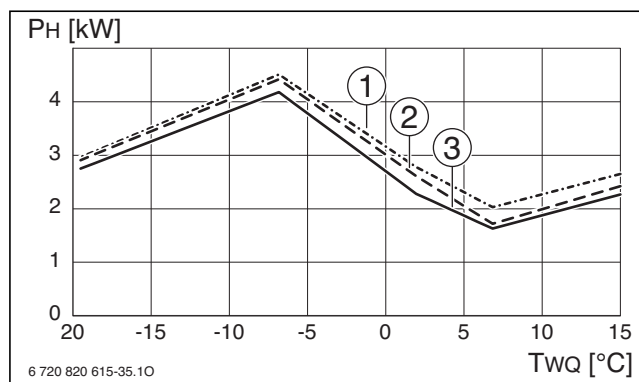
Bild 76 Heizleistung (P H ) CS7001iAW 5 OR-S
