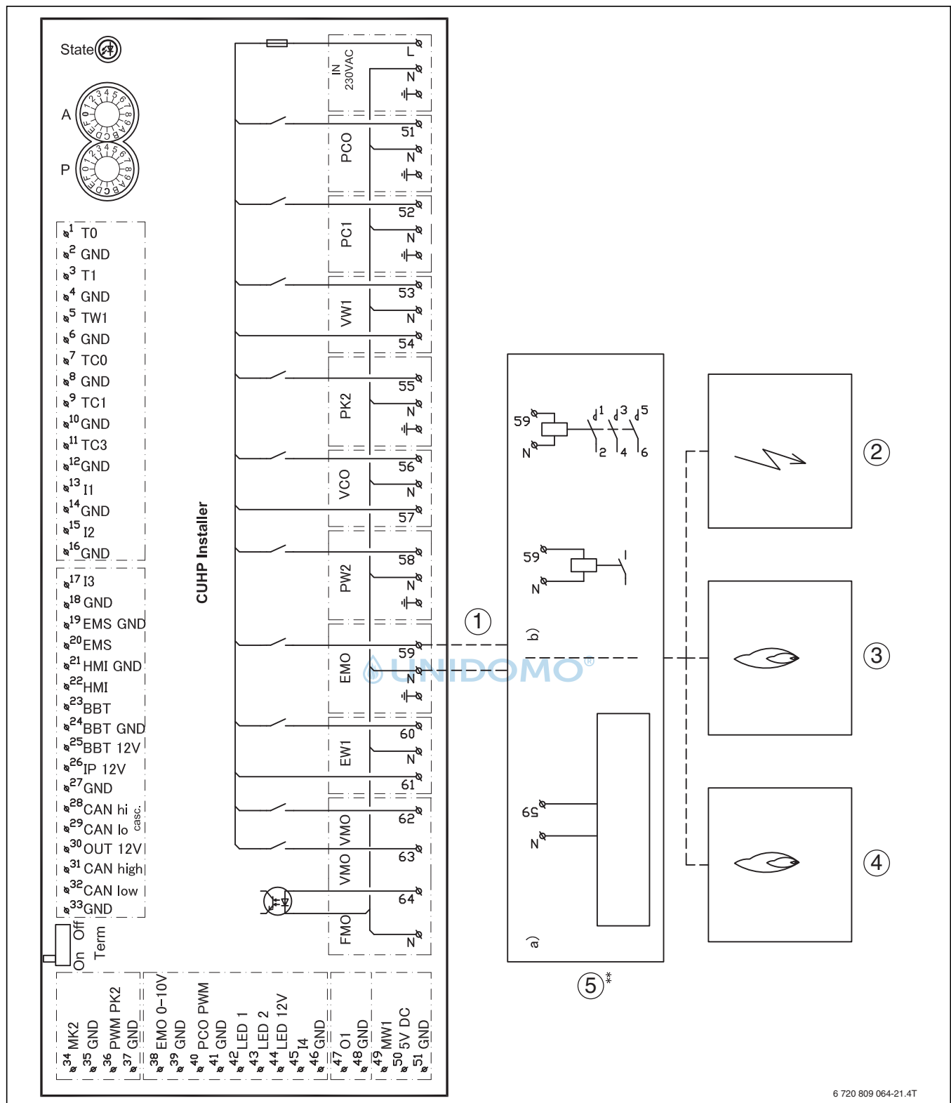
Bild 144 Schaltplan Installationsmodul, Start/Stopp
