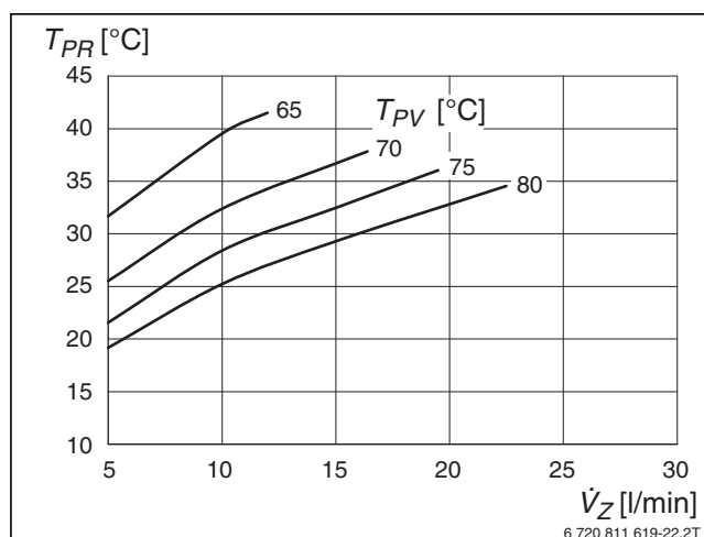
Bild 199 Volumenstrom vom Pufferspeicher (Rücklauf) bei 60 °C Zapftemperatur
