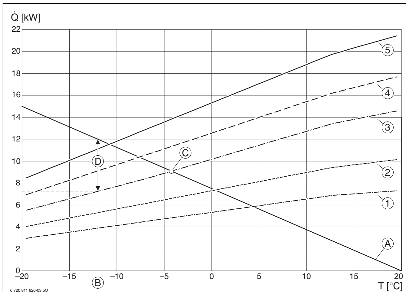
Bild 30 Bivalenztemperatur, Heizleistungskurven der Wärmepumpen Compress 7000i AW bei 35 °C Vorlauftemperatur (schematische Darstellung)
