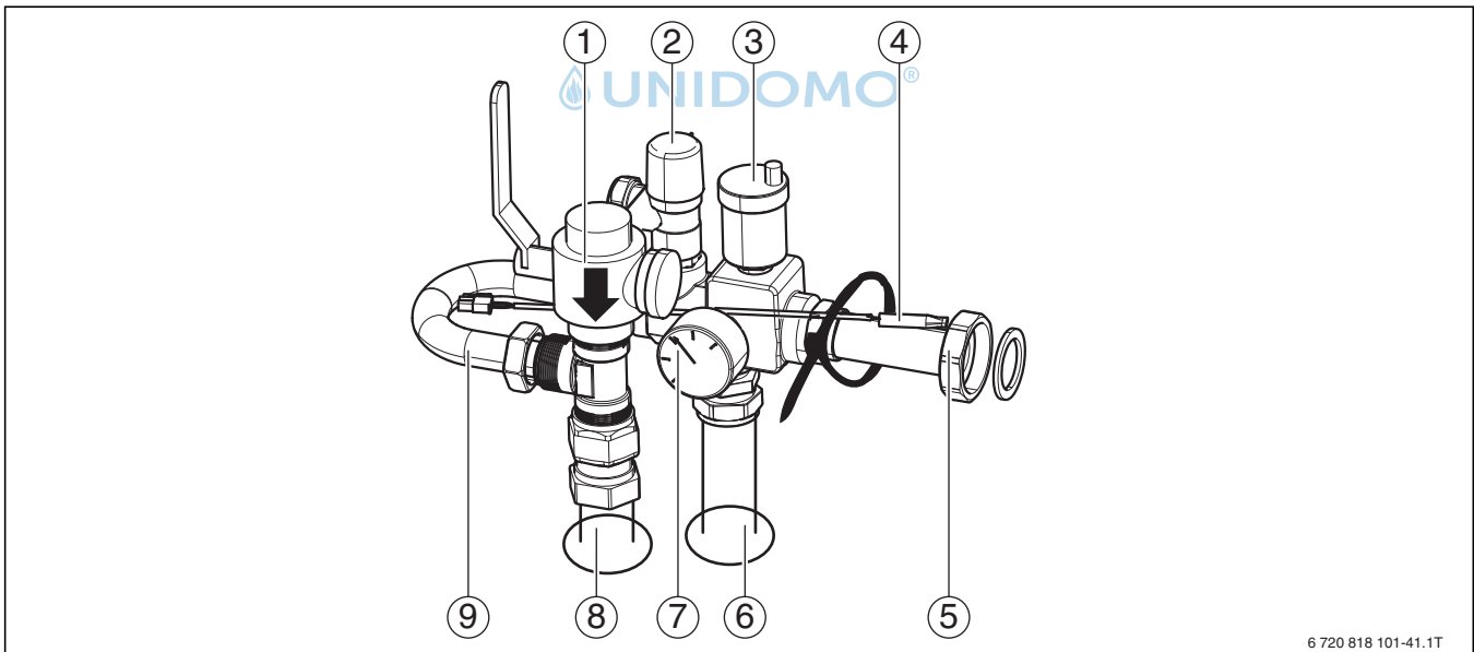
Bild 106 Montierte Sicherheitsgruppe
