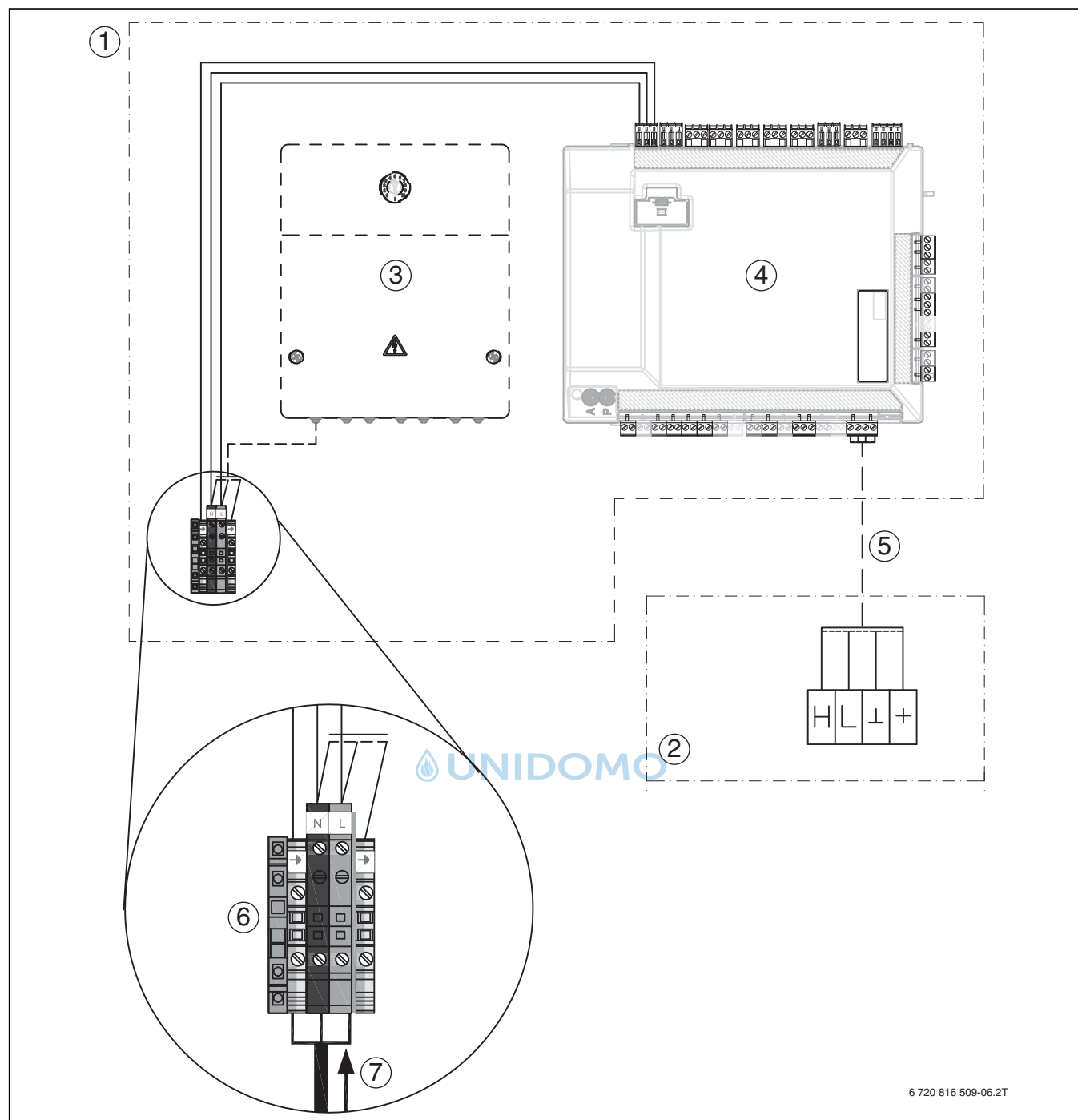
Bild 142 Inneneinheit mit externem Zuheizer – Überblick
