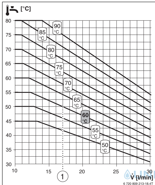
Bild 195 Temperaturverhalten Frischwasserstation FF 20
