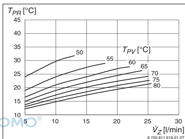
Bild 198 Volumenstrom zum Pufferspeicher (Rücklauf) bei 45 °C Zapftemperatur
