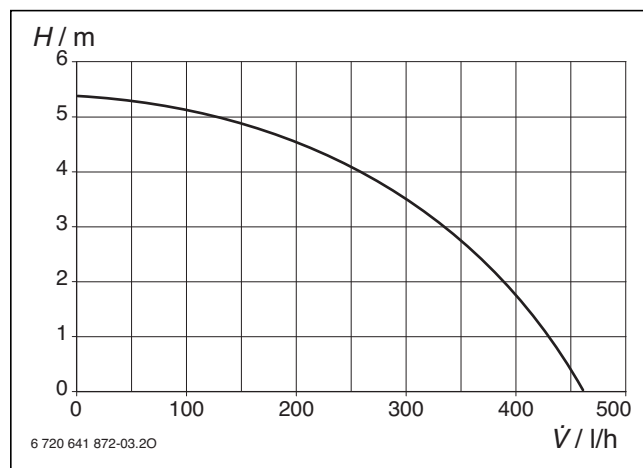
Bild 48 Kondensatpumpendiagramm: Förderhöhe über Volumenstrom
