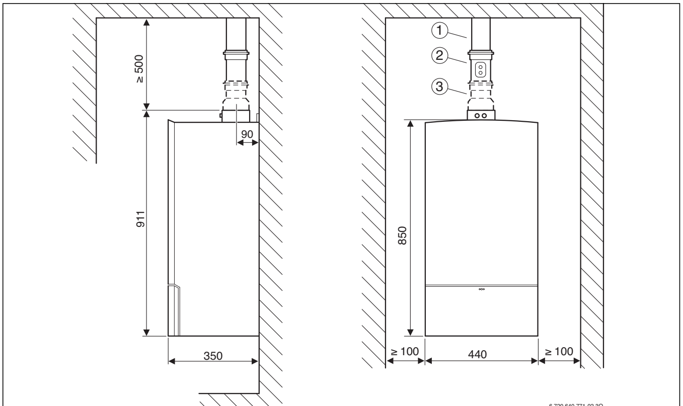
Bild 63 Flachdach
