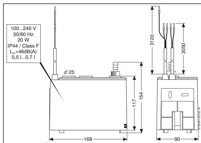
Bild 47 Kondensatpumpe
