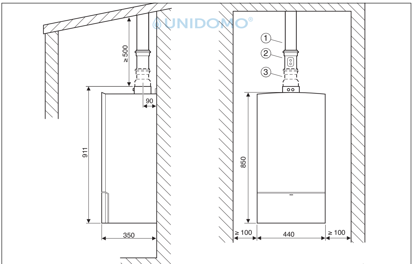
Bild 64 Schrägdach
