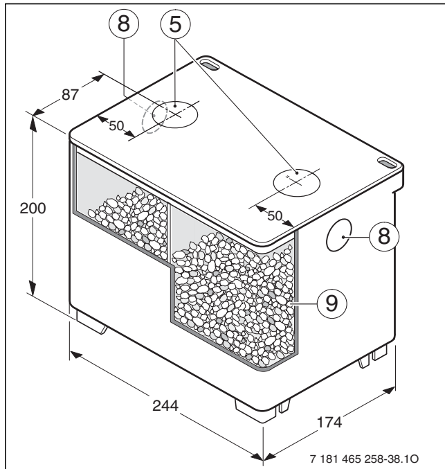
Bild 49 Neutralisationseinrichtung
