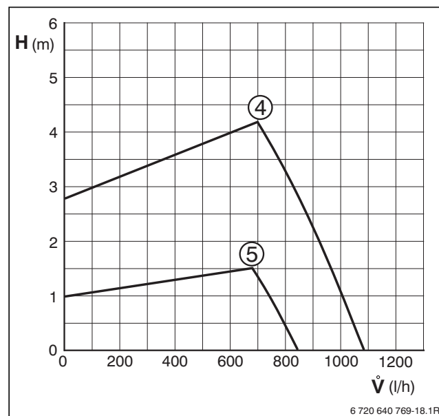
Bild 43 Proportionaldruck - Gerät mit Pufferspeicher SP 400 SHU-2 und Anschluss-Set Zubehör Nr. 1463
