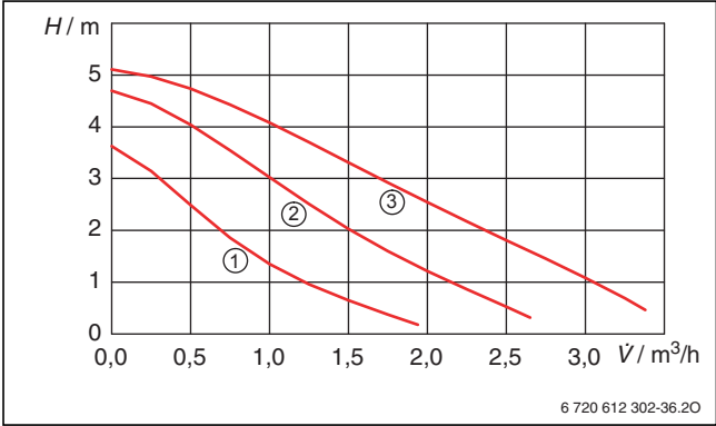
Bild 52 Pumpenkennliniendiagramm
