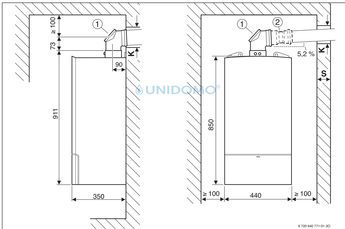
Bild 62 Abgasführung Ø 80/125 mm, Ø 80 mm oder Ø 60/100 mm
