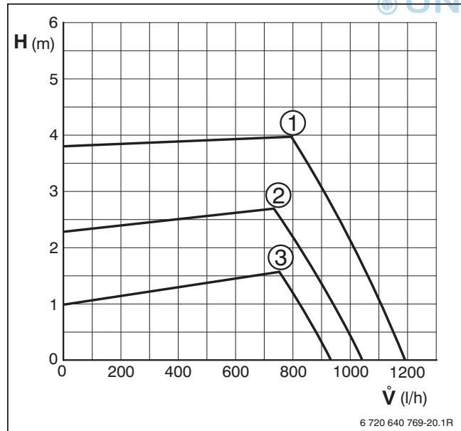
Bild 42 Konstantdruck - Gerät ohne Pufferspeicher und Verrohrung
