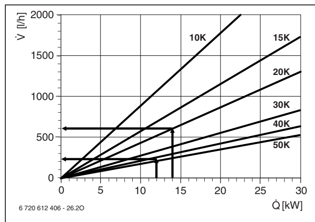
Bild 89 Volumenstrom Primärkreis
