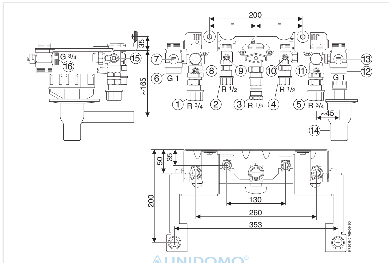
Bild 32 Montageanschlussplatte Nr. 1469
