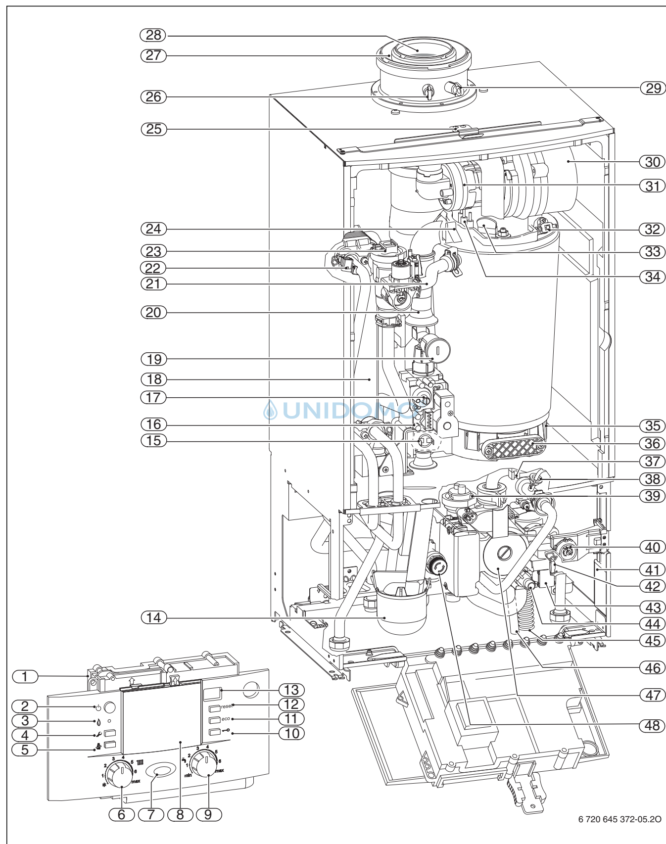
Bild 34 Gas-Brennwertgerät
