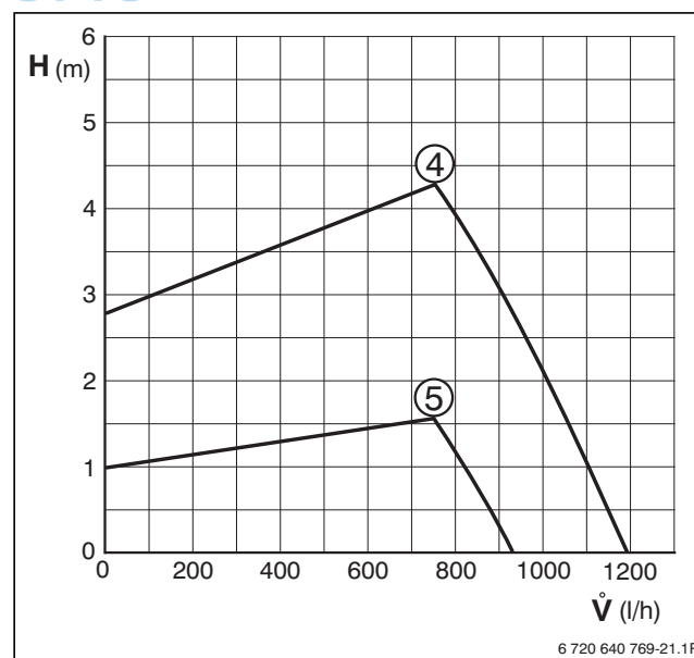
Bild 44 Proportionaldruck - Gerät ohne Pufferspeicher und Verrohrung
