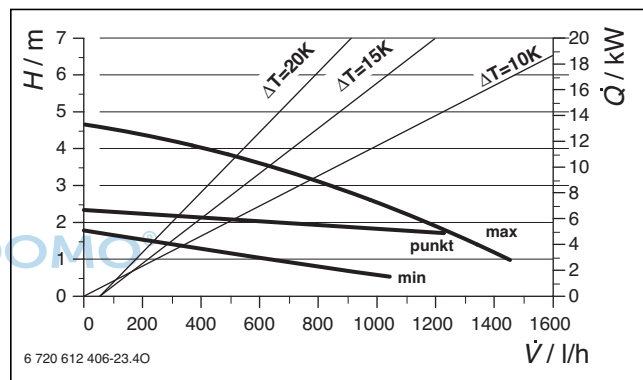
Bild 90 Leistungsfelder gemischter Heizkreis
