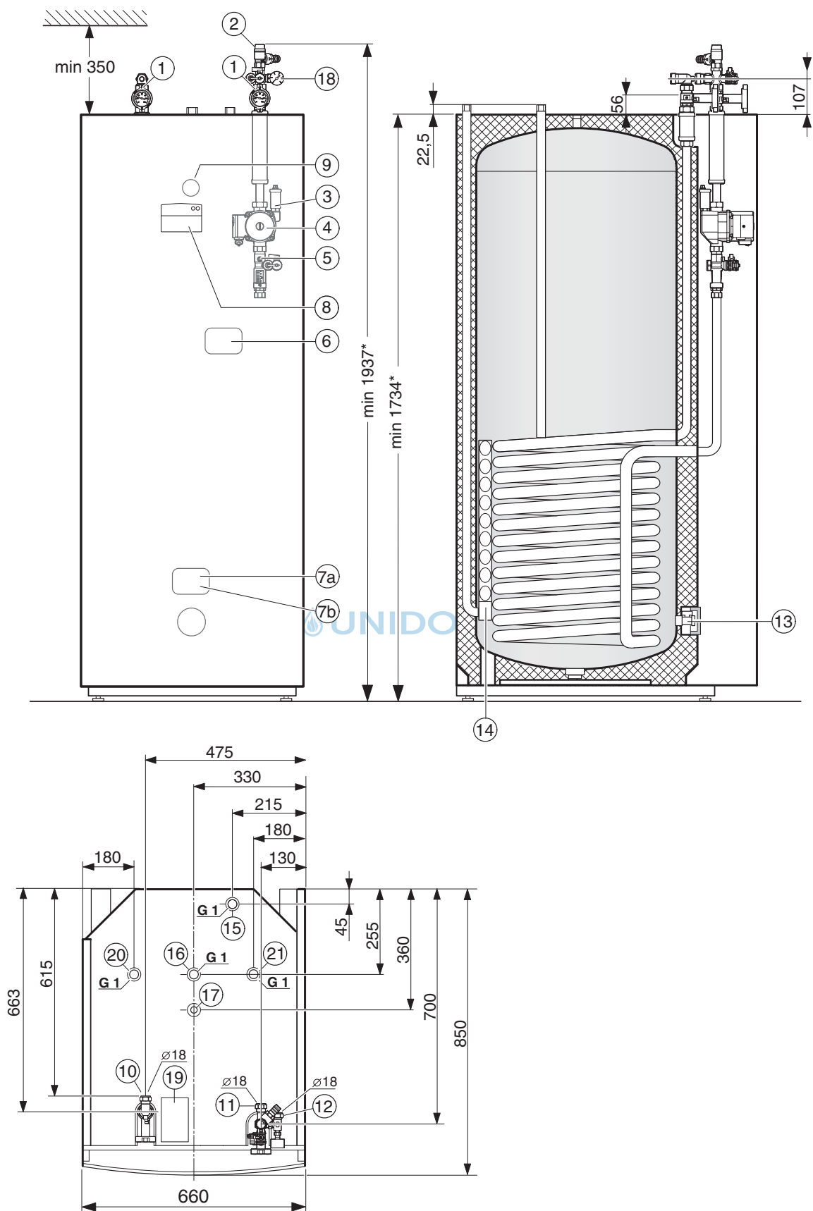
Bild 37 Bau- und Anschlussmaße SP 400 SHU-2
