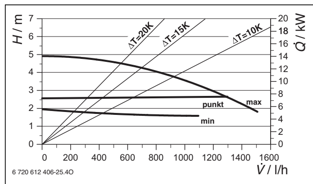
Bild 91 Leistungsfelder ungemischter Heizkreis
