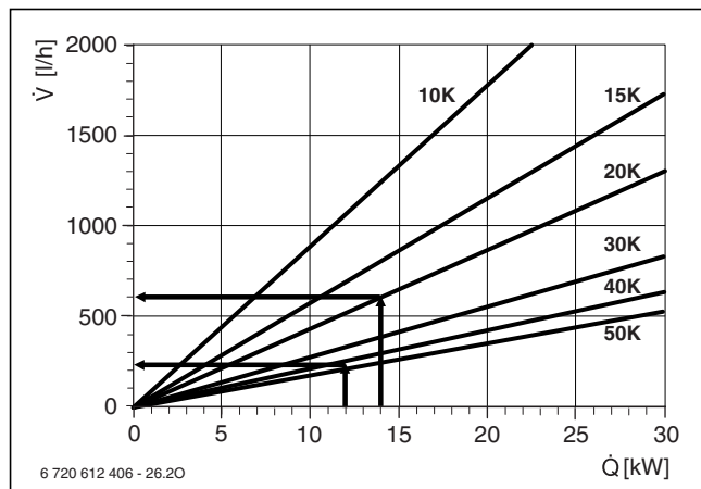
Bild 108 Volumenstrom Primärkreis
