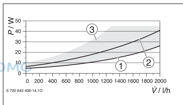
Bild 112 Leistungsaufnahme
