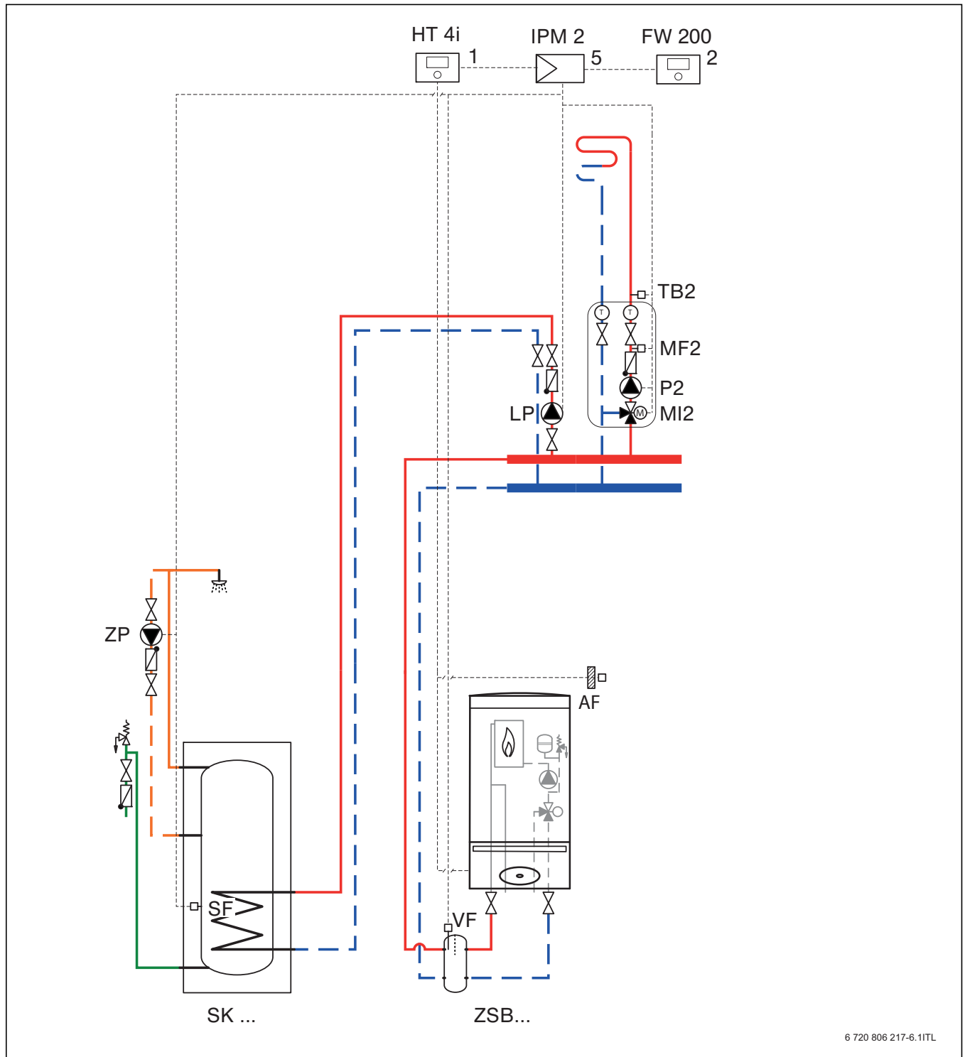
Bild 6 Beispiel hydraulische Weiche mit Warmwasserspeicher und einem gemischten Heizkreis
