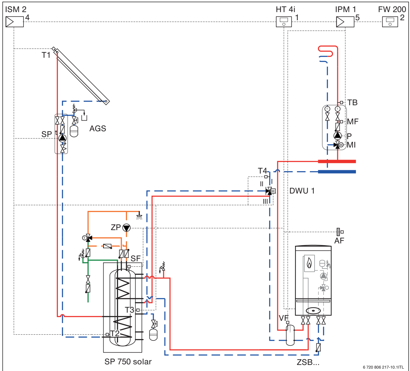
Bild 10 Beispiel solare Heizungsunterstützung mit gemischtem Heizkreis (Solarsystem 2)
