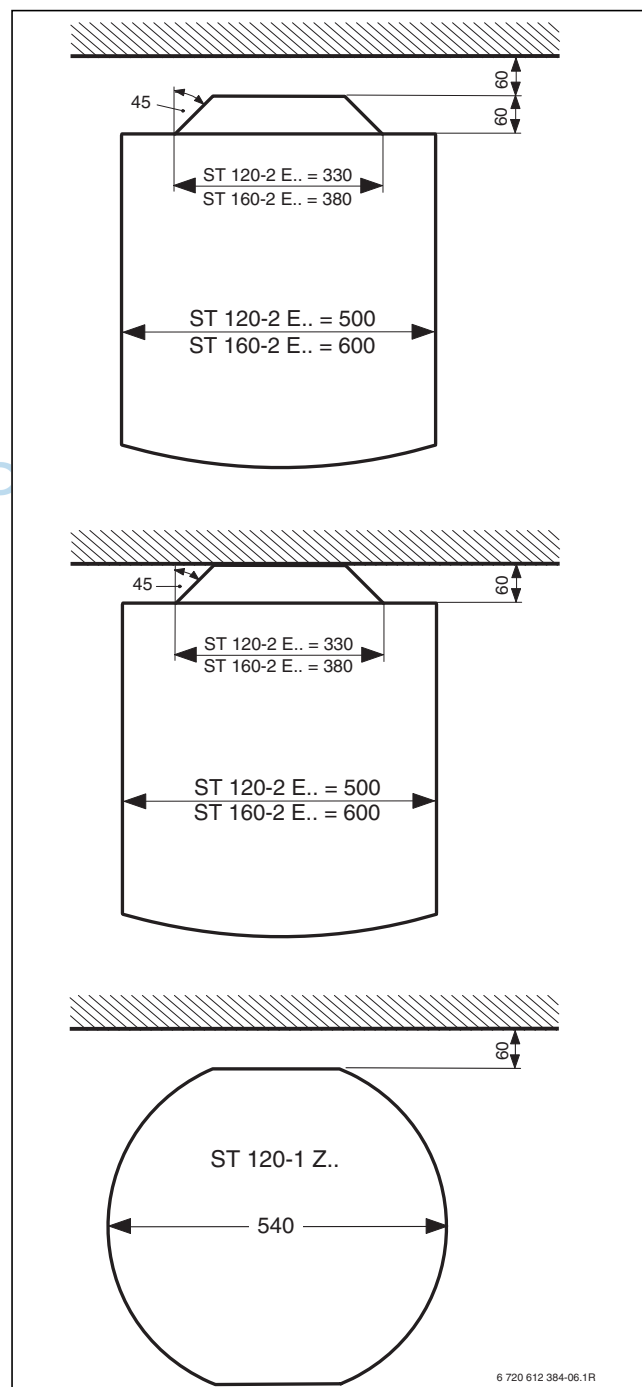
Bild 63 Wandabstandsmaße
