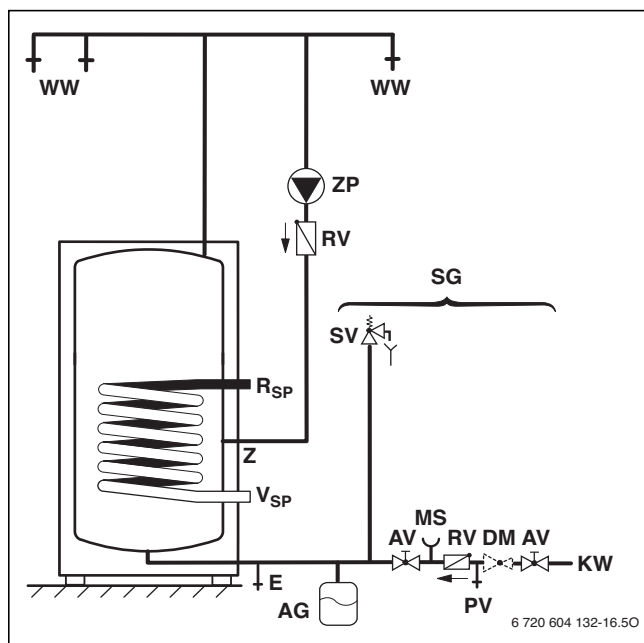
Bild 51 Warmwasserseitiges Anschluss-Schema
