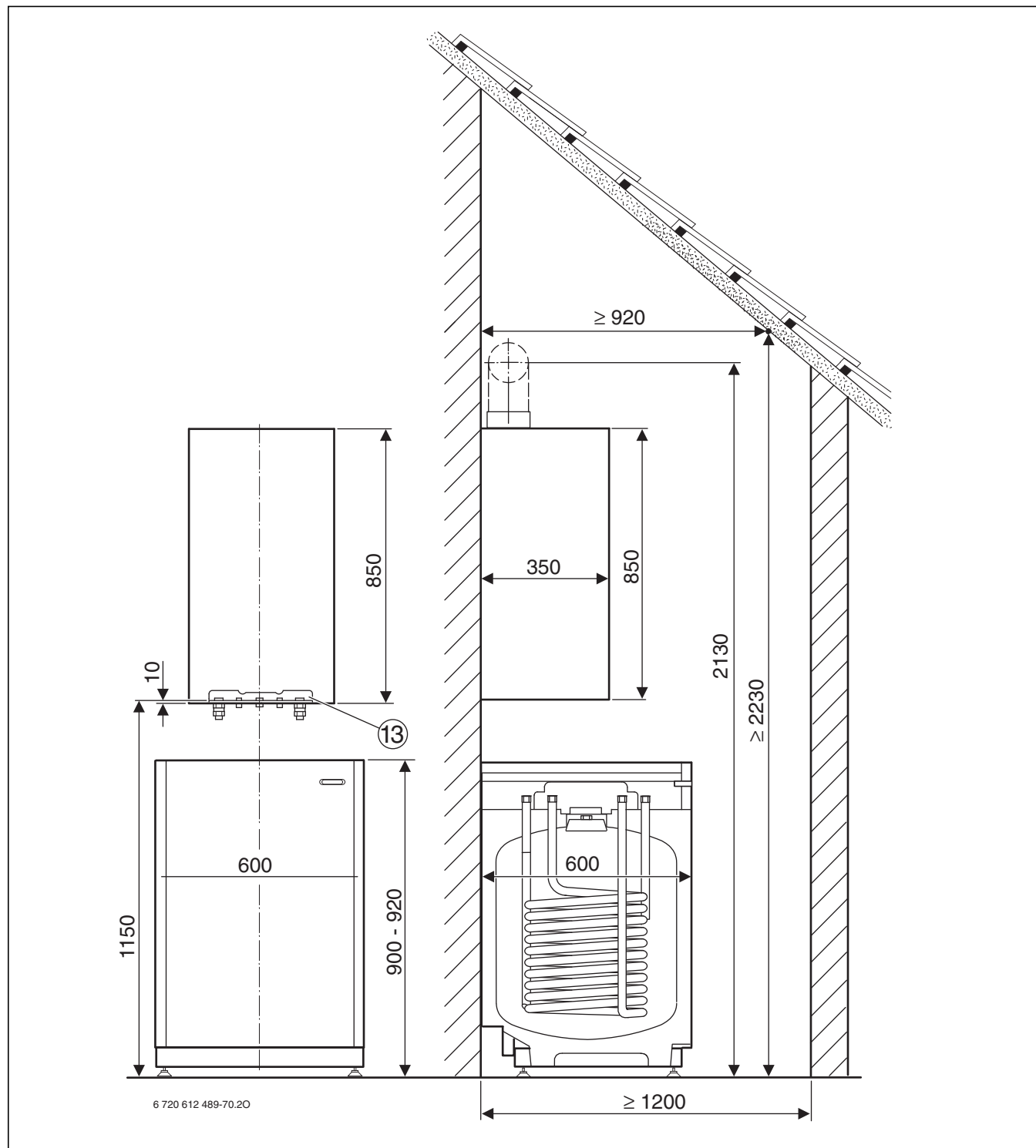
Bild 78 Einbaumaße SE 120-1
