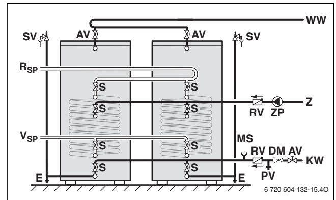
Bild 52 Parallelschaltung
