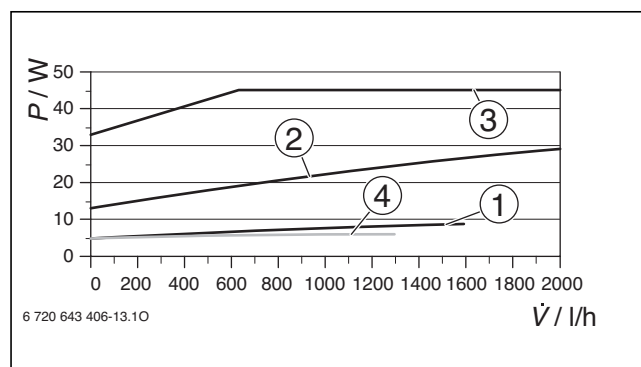
Bild 110 Leistungsaufnahme
