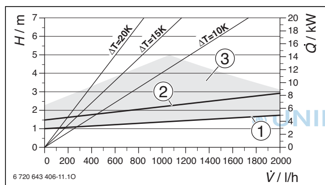
Bild 111 Pumpenkennlinien
