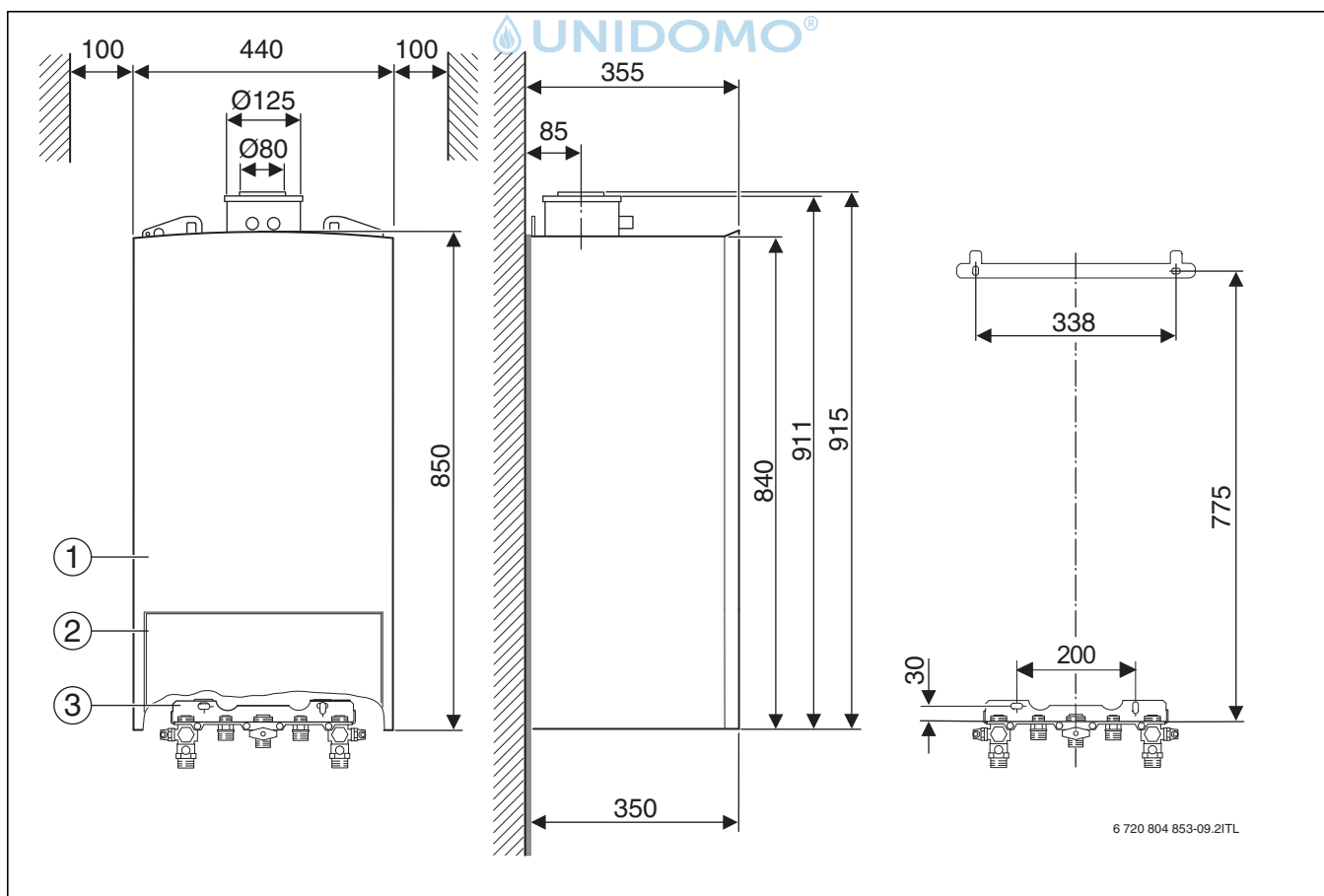
Bild 18 Abmessungen Cerapur
