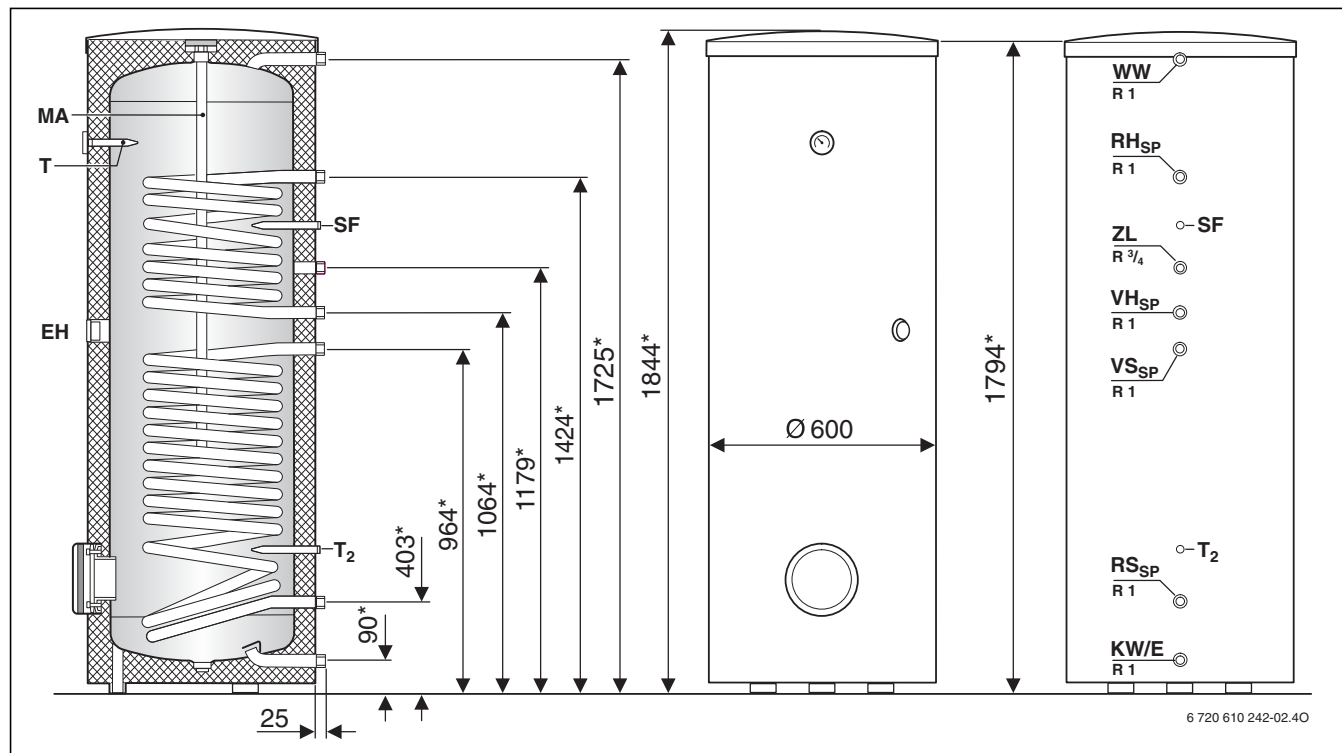
Bild 91 Bau- und Anschlussmaße SKE 290-5 solar
