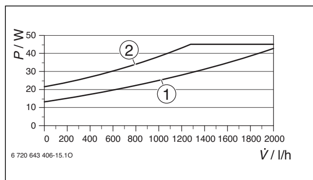
Bild 114 Leistungsaufnahme
