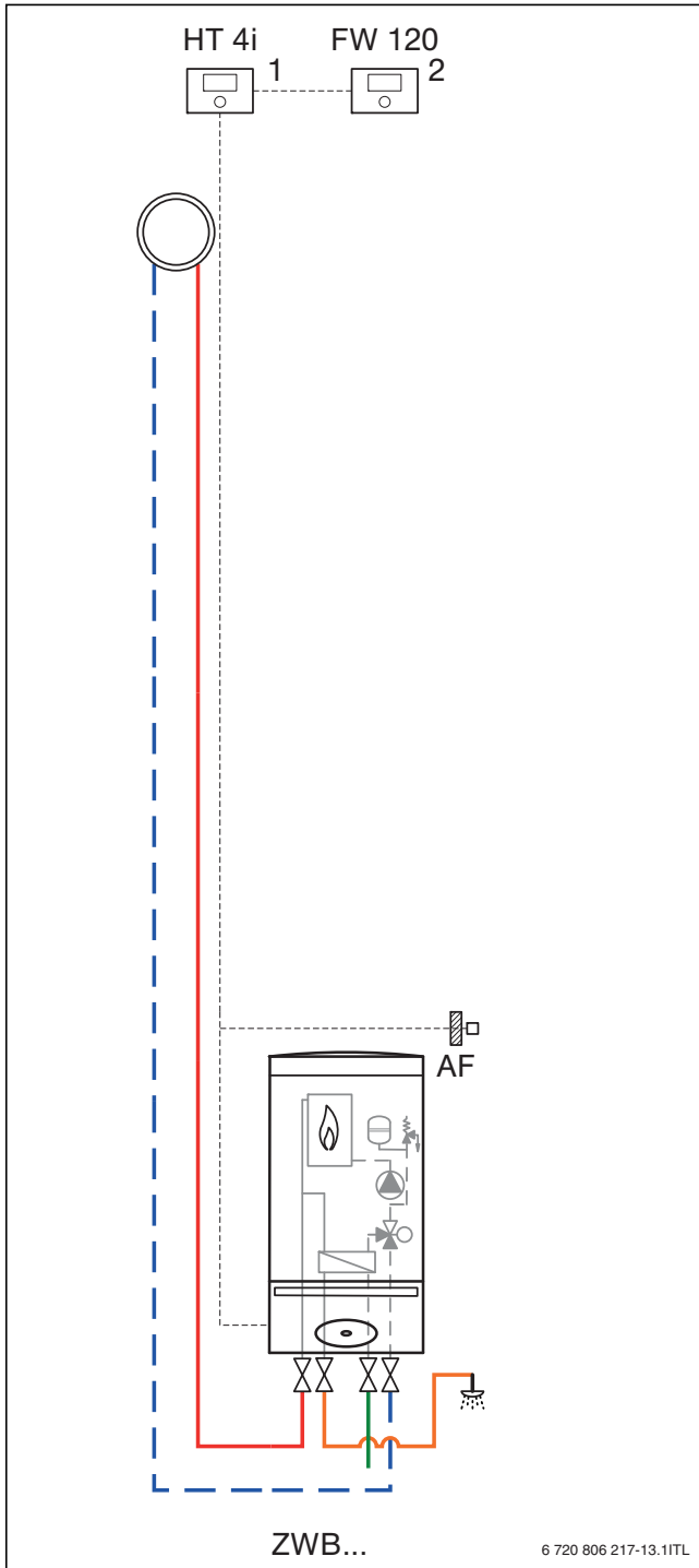
Bild 13 Beispiel mit außertemperaturgeführtem Regler FW 120
