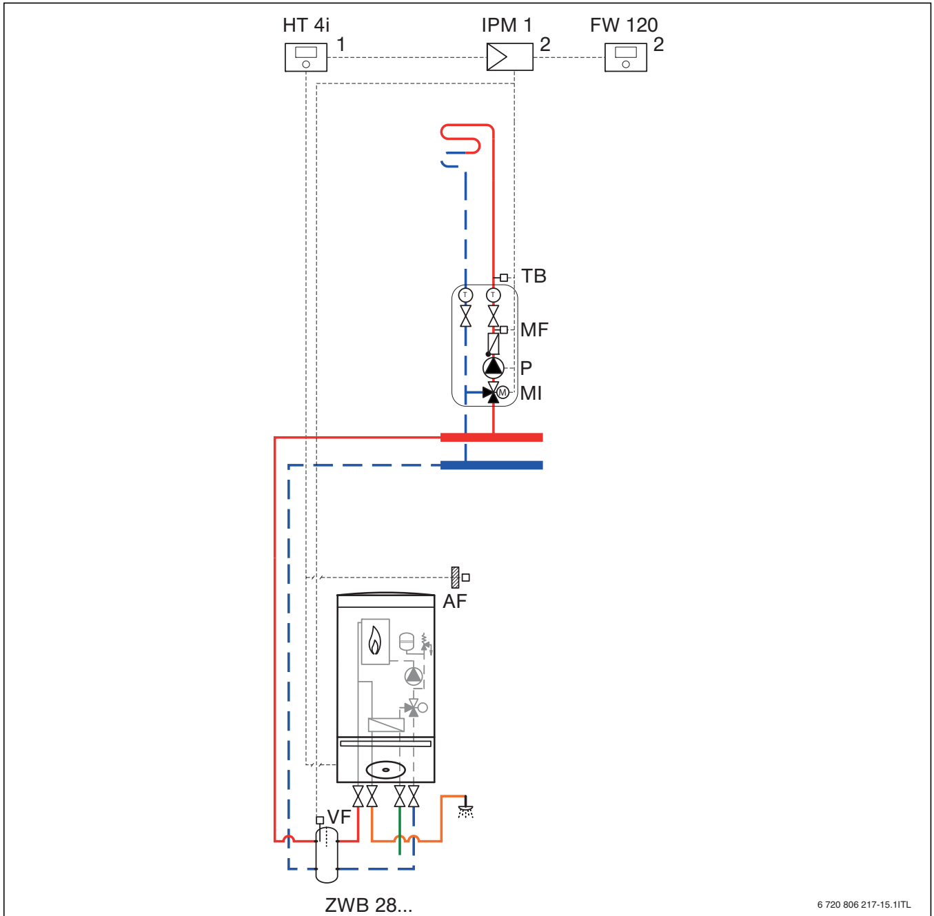
Bild 15 Beispiel Fußbodenheizung über 900 l/h
