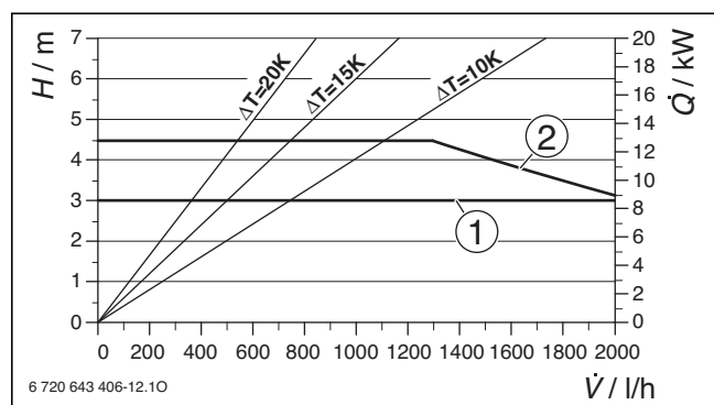
Bild 113 Pumpenkennlinien
