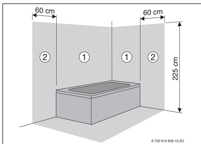
Bild 36 Schutzbereiche
