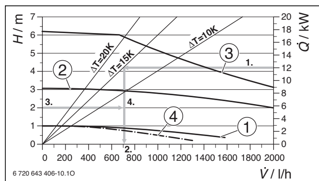
Bild 109 Pumpenkennlinien
