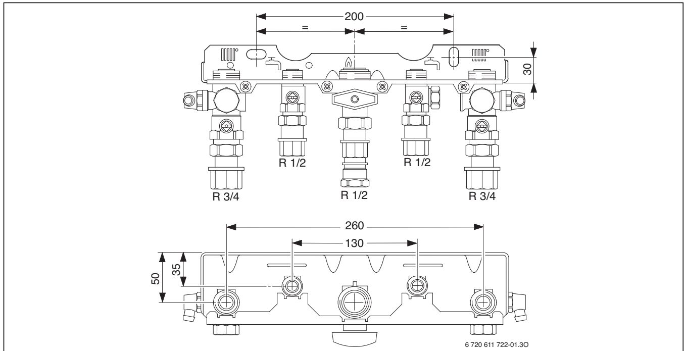
Bild 22 Anschlussmaße Montageanschlussplatte Zubehör Nr. 991
