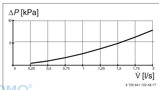
Bild 33 Druckverlust
