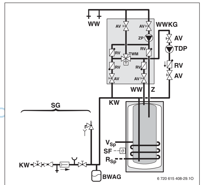
Bild 61 Trinkwasserseitiges Anschlusschema bei solarer Heizungsunterstützung
