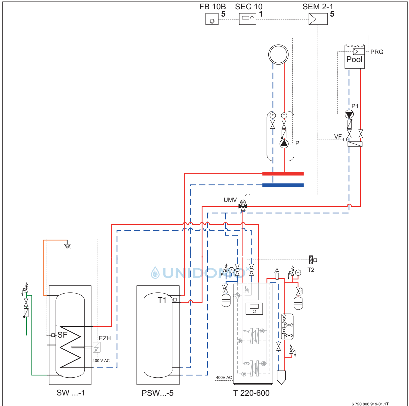
Bild 4 Anlagenschema 4
