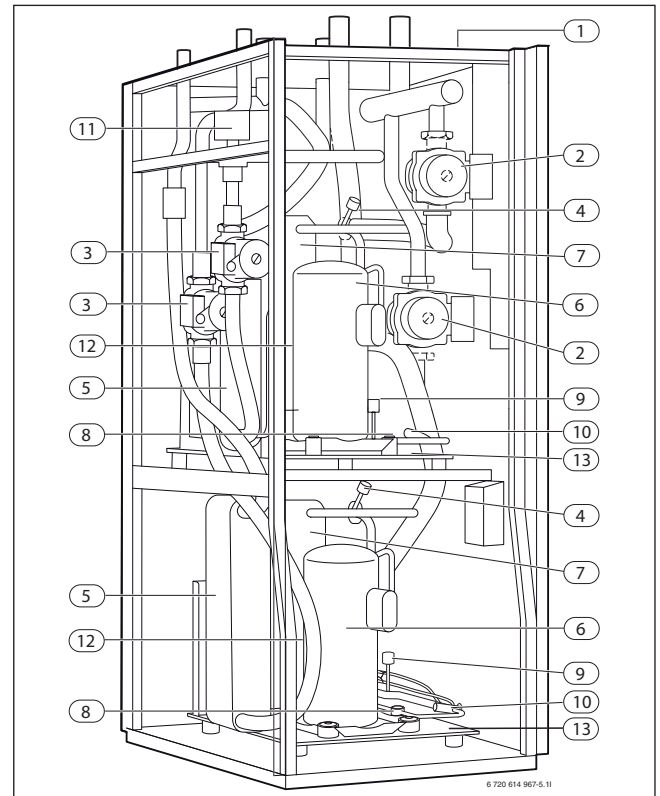
Bild 6 Ausgewählte Bauteile und Baugruppen der Wärmepumpe T 330-2
