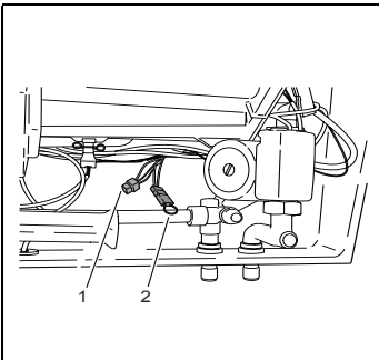
Fig. 7 Fiche Fig. 7 Clavija Fig. 7 Connettore flottante
