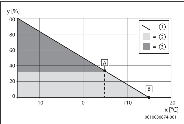
Bild 1 Außentemperatur parallel
