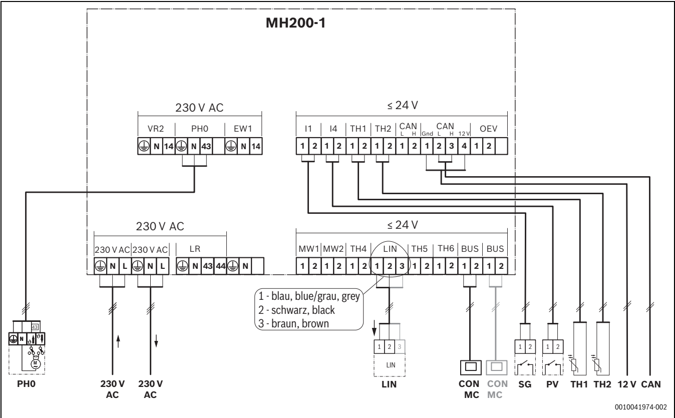
Bild 3 Überblick Anschlussklemmenbelegung
