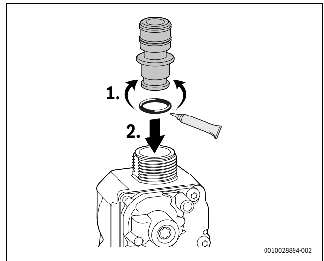
Bild 86 Gasdrossel einsetzen
