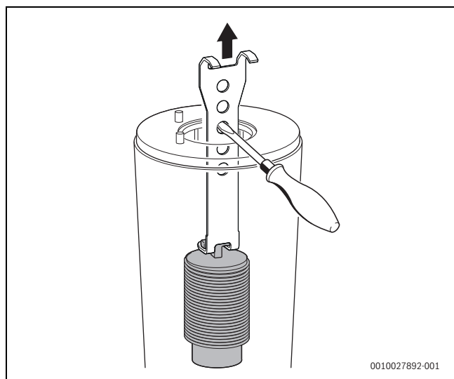
Bild 66 Unteren Verdrängungskörper herausnehmen
