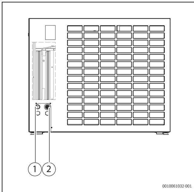
Bild 31 Kabeldurchführungen
