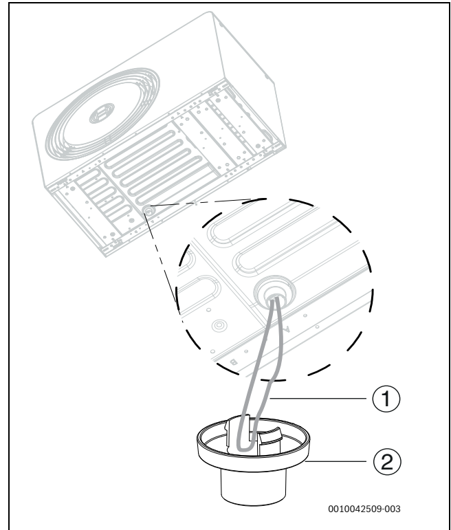
Bild 24 Installation des Ablaufstutzens
