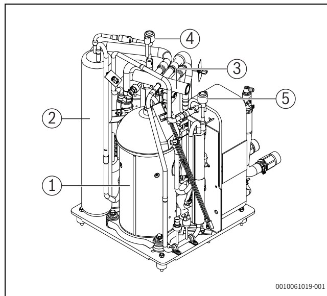
Bild 2 Produktübersicht – Vorderansicht
