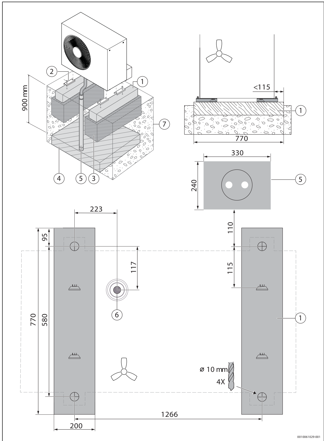
Bild 22 Fundamentplan, Alternative 1
