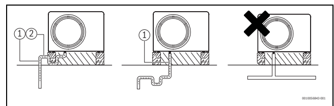
Bild 25 Kondensatableitung in den Abwasser-/Regenwasserabfluss
