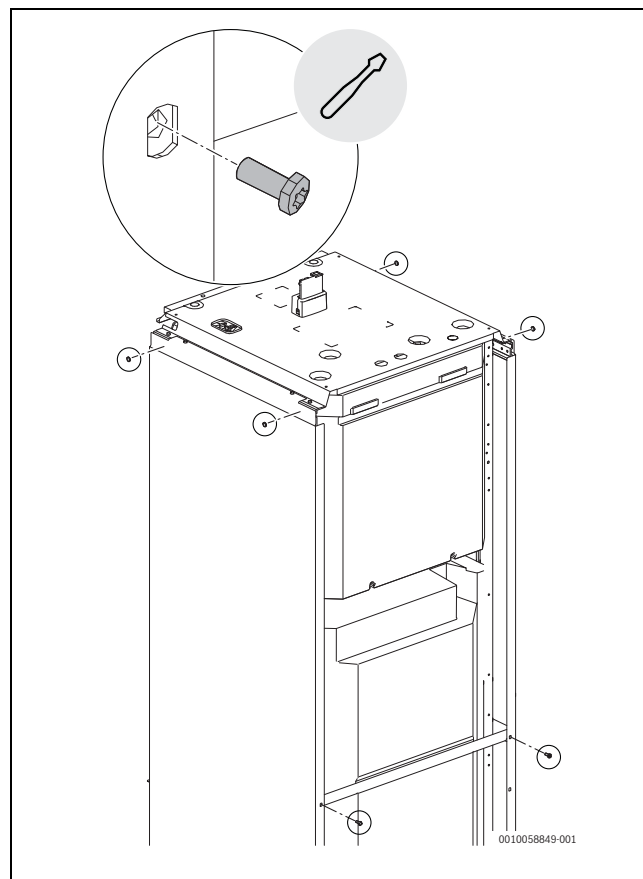
Bild 16 Schrauben für die Seitenwände
