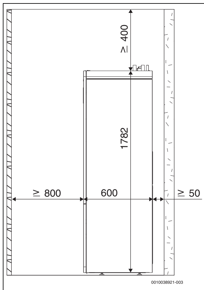
Bild 2 Mindestabstand (mm)
