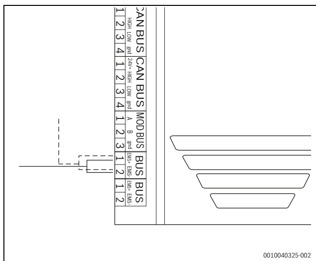
Bild 34 EMS-Anschluss
