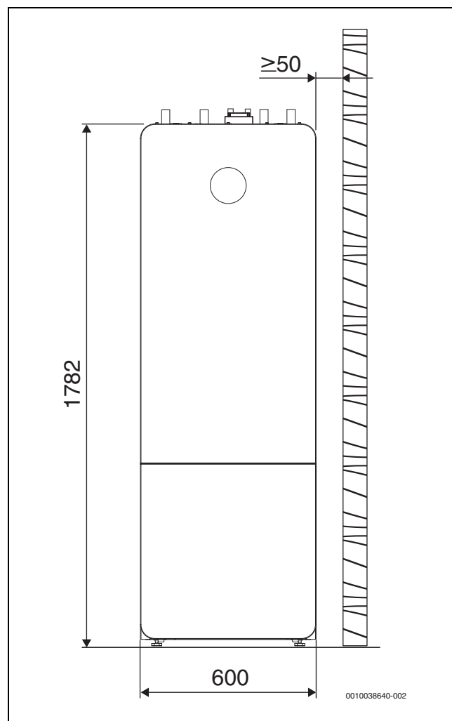
Bild 3 Abmessungen (mm)
