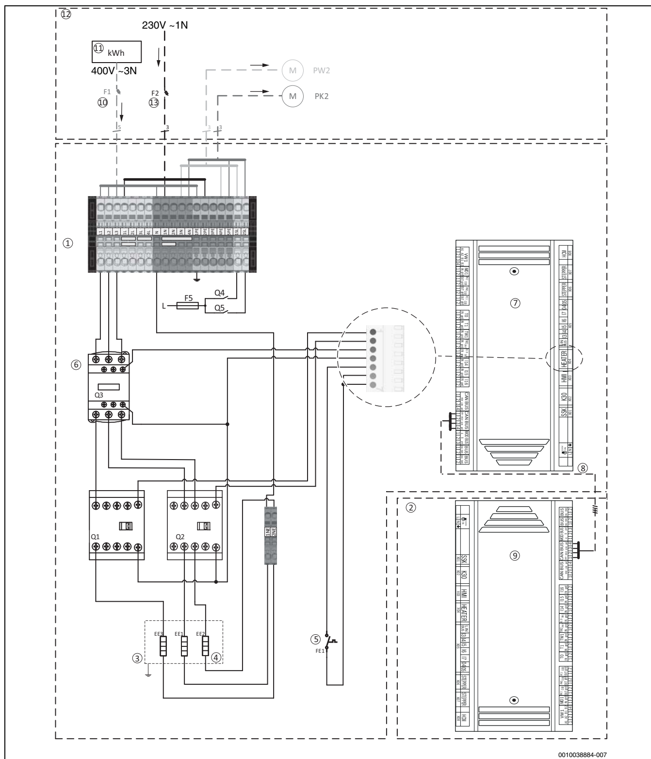
Bild 56 Spannungsversorgung Inneneinheit
