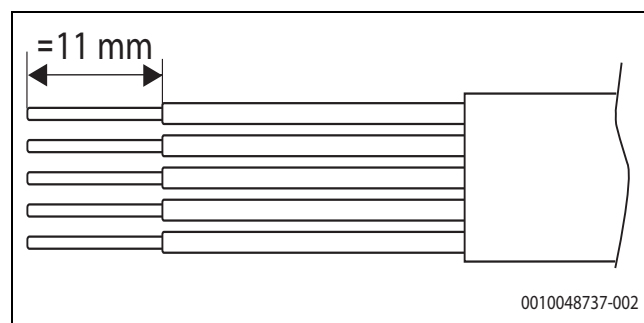
Bild 36 Abisolieren der Adern für den Netzanschluss
