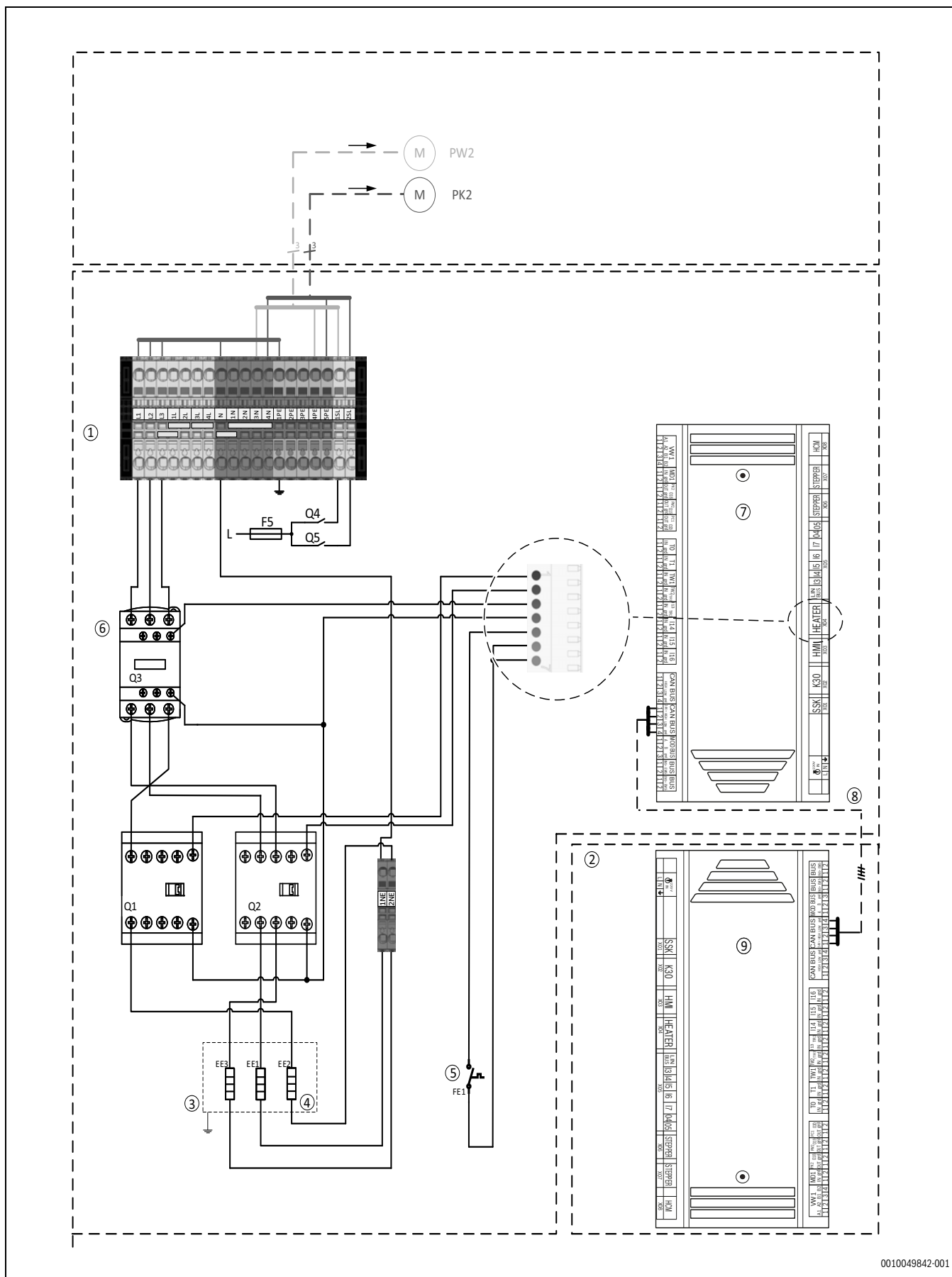
Bild 57 Spannungsversorgung Inneneinheit
