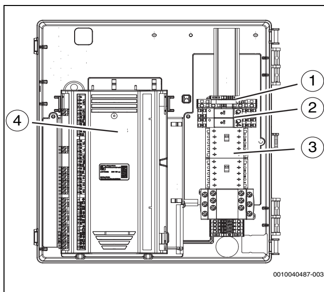
Bild 39 Anordnung der Komponenten im Klemmenkasten
