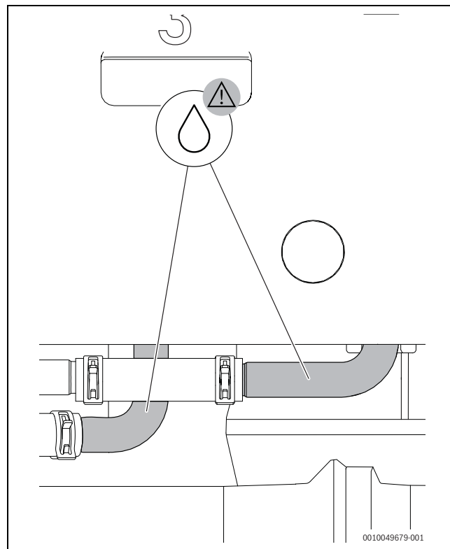
Bild 24 Röhren, die isoliert werden müssen, wenn der Kühlbetrieb bei Temperaturen unter dem Taupunkt verwendet wird.
