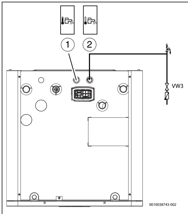
Bild 29 Wärmepumpenanschlüsse Trinkwasser
