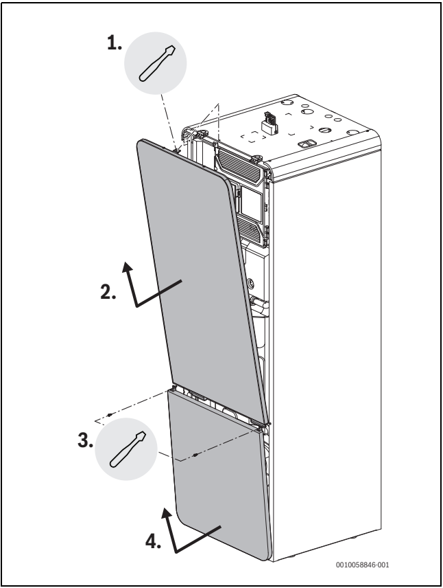
Bild 13 Frontplatte
