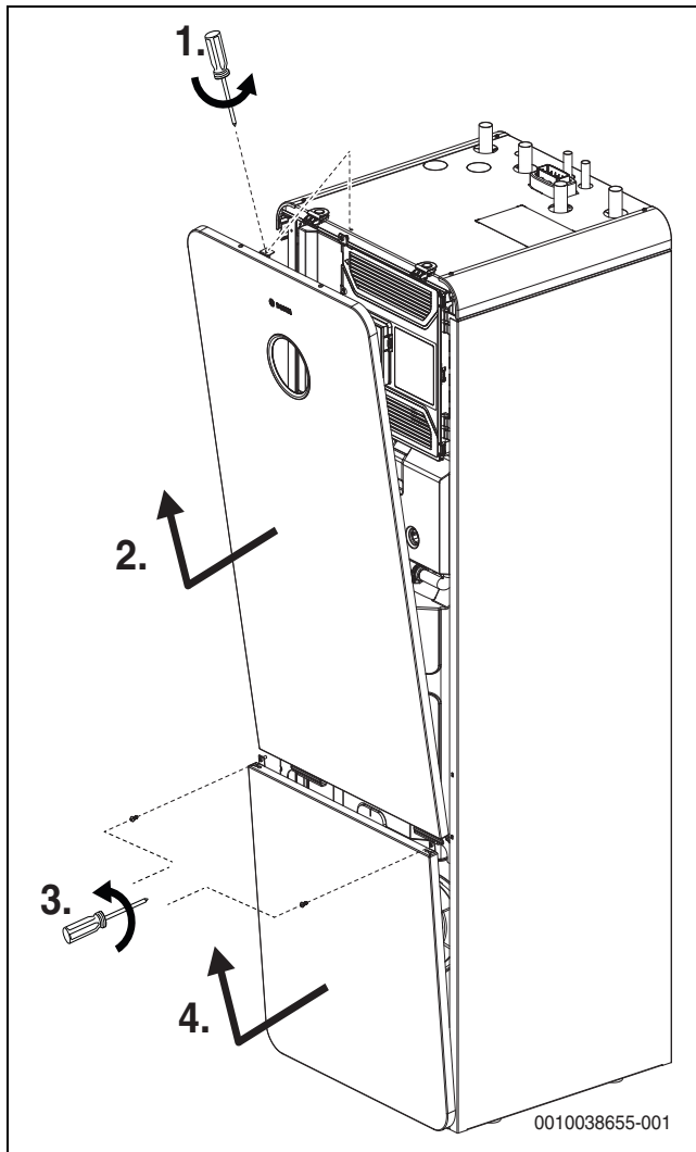
Bild 20 Front abnehmen
