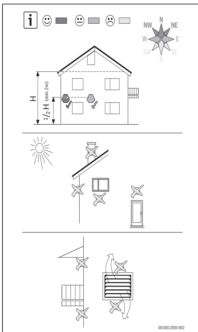
Bild 35 Position des Außentemperaturfühlers
