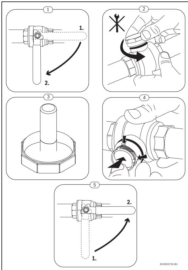
Bild 50 Siebreinigung
