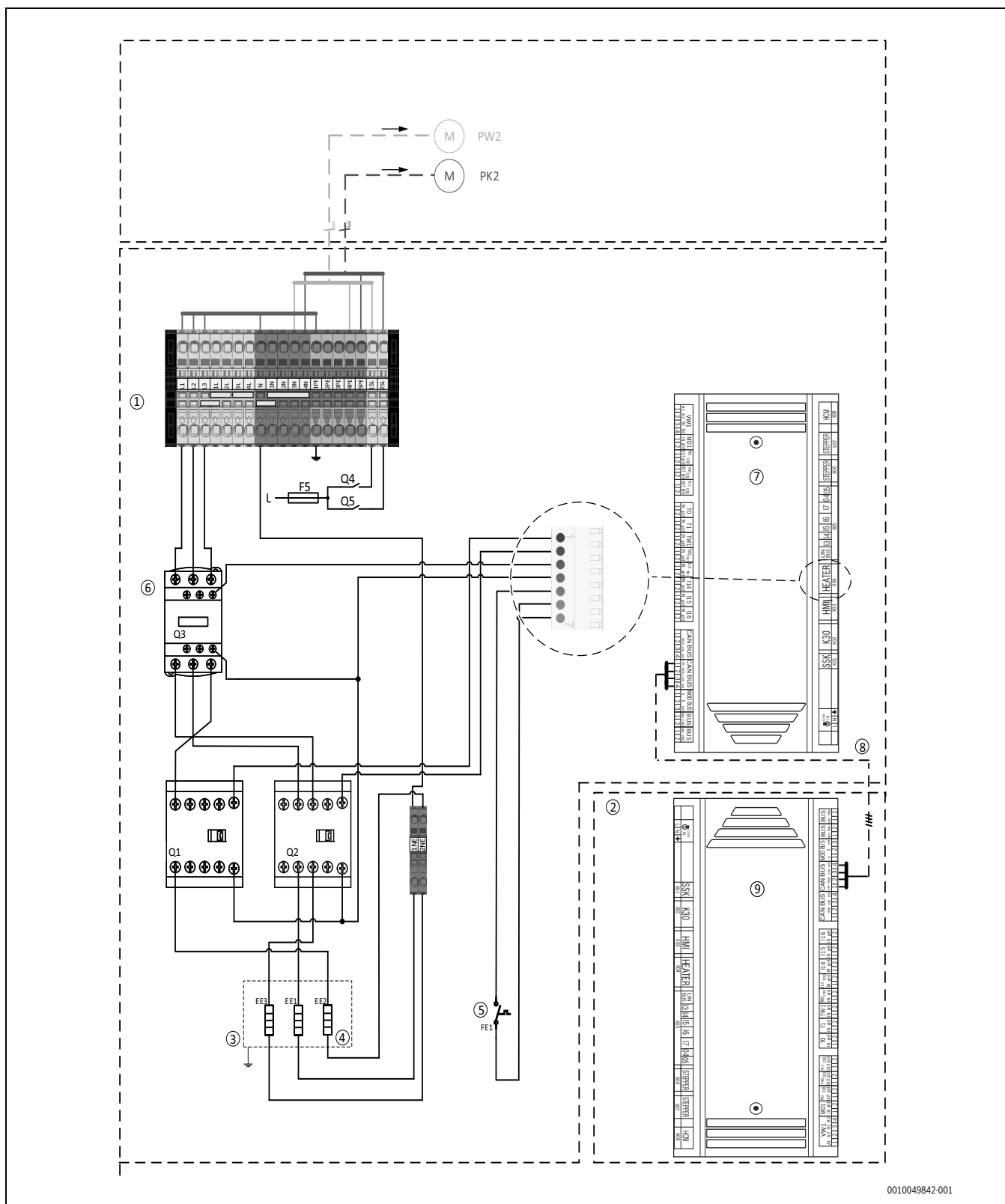
Bild 57 Spannungsversorgung Inneneinheit
