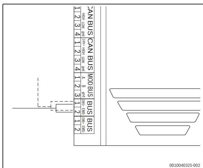
Bild 34 EMS-Anschluss
