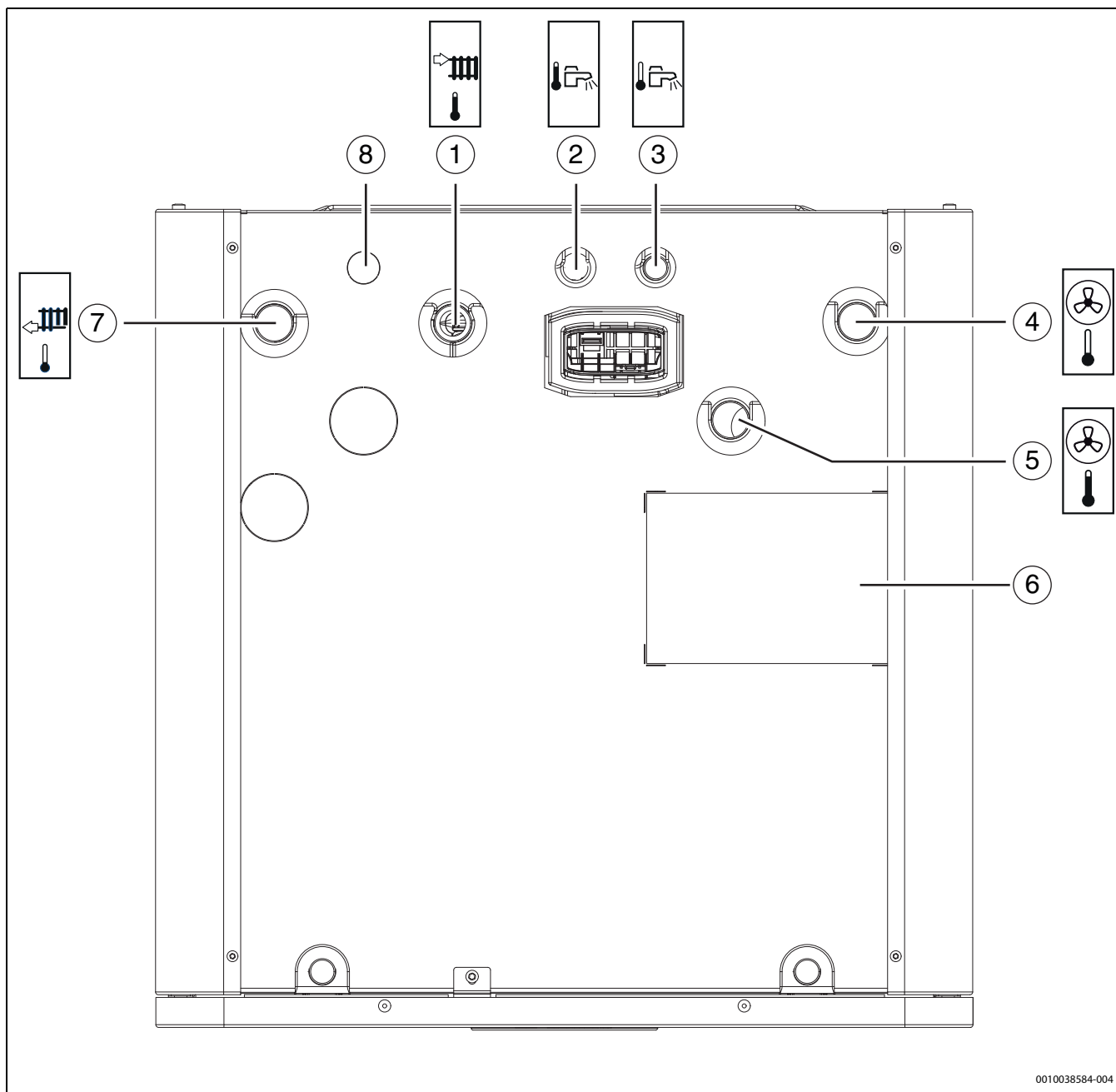
Bild 6 Produktübersicht – Draufsicht
