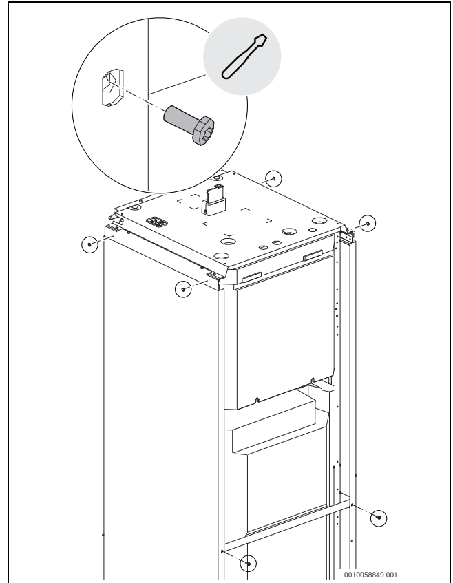
Bild 16 Schrauben für die Seitenwände
