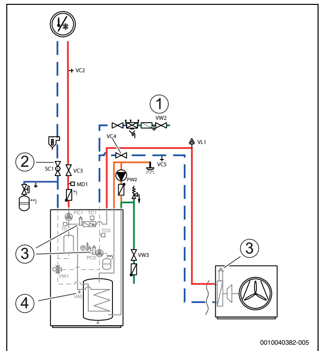
Bild 30 Inneneinheit, Wärmepumpe und Heizungsanlage
