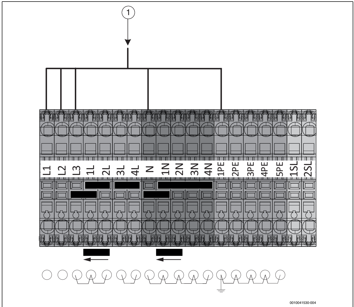
Bild 40 Elektrische Anschlüsse ohne EVU-Sperre
