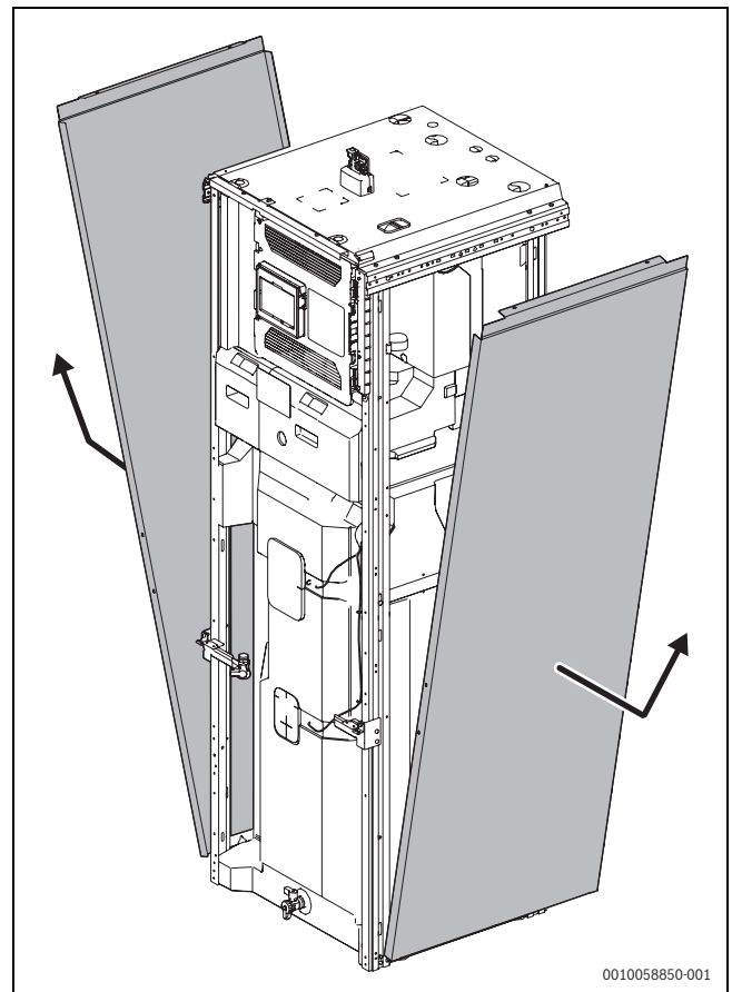
Bild 17 Seitenwände
