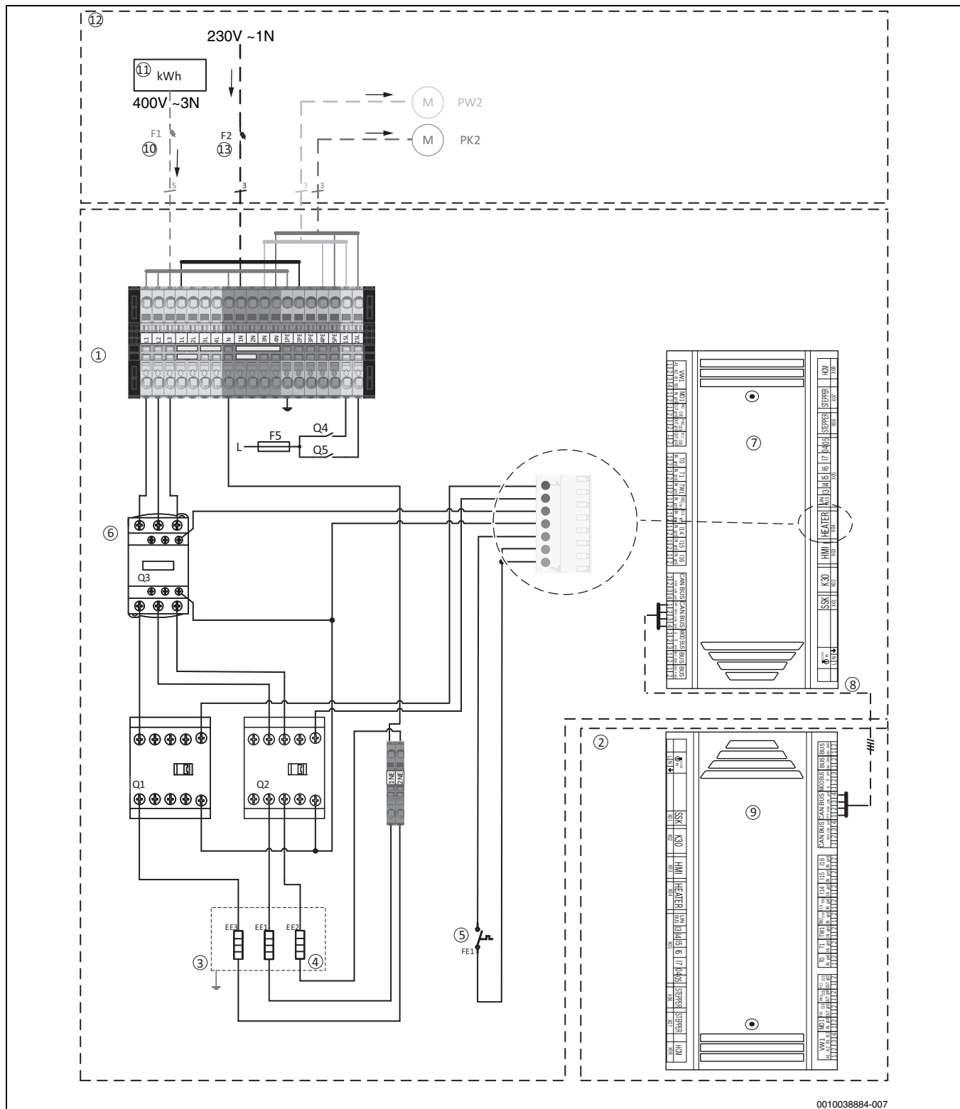
Bild 56 Spannungsversorgung Inneneinheit
