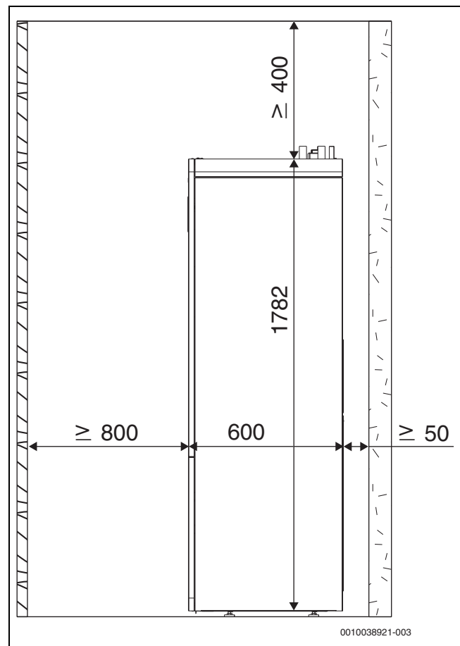
Bild 2 Mindestabstand (mm)
