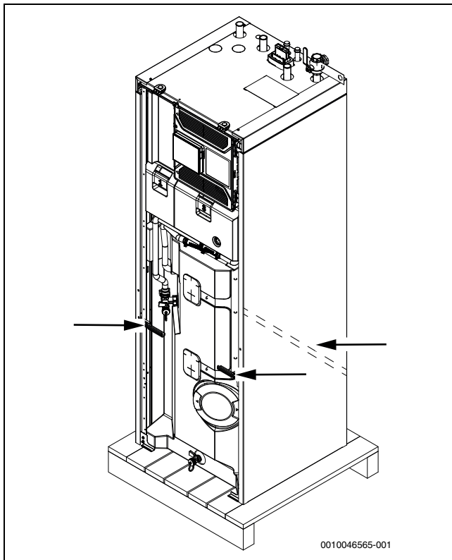
Bild 10 Transportbügel
