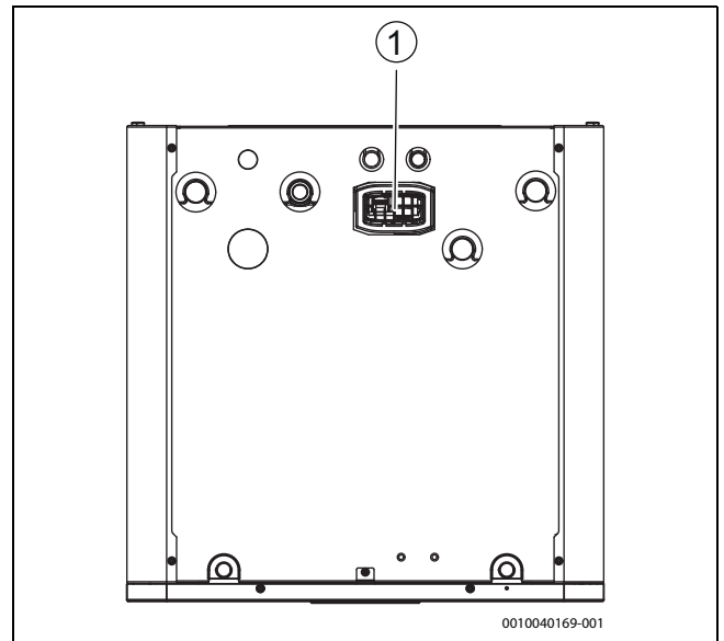
Bild 21 Connect-Key platzieren
