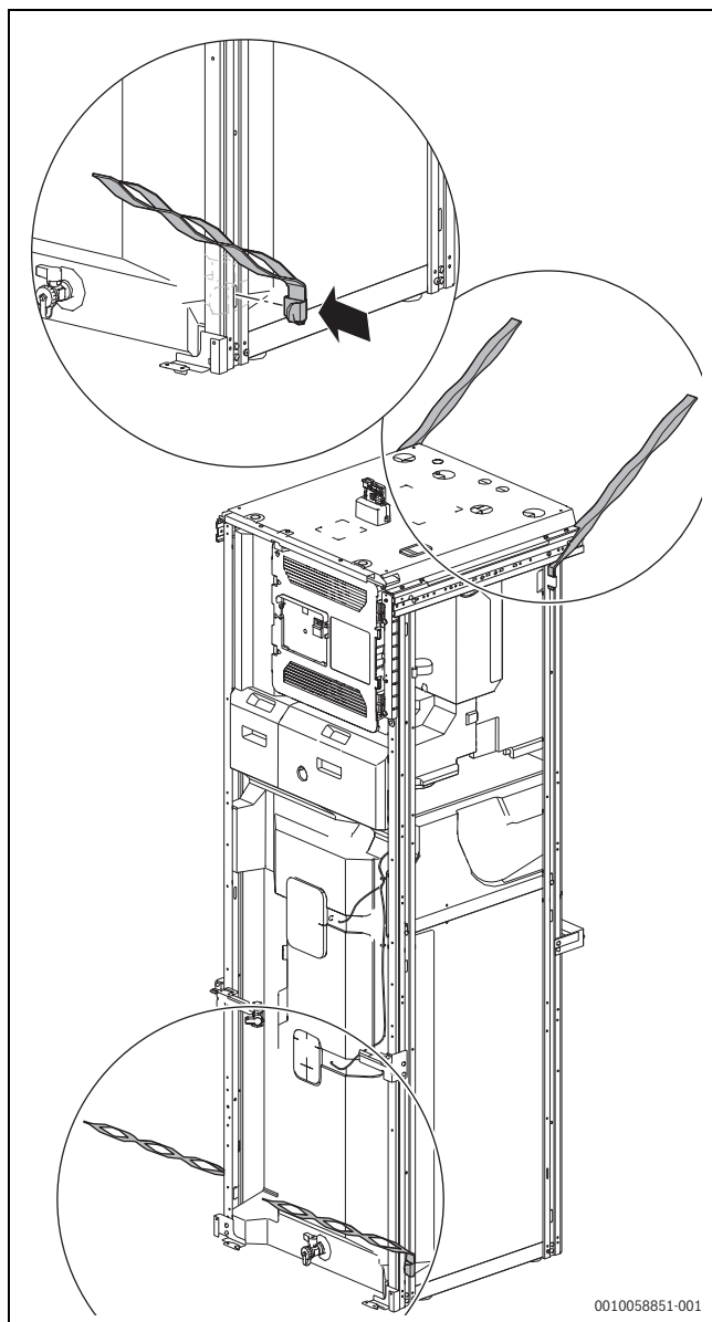
Bild 18 Transportgurte
