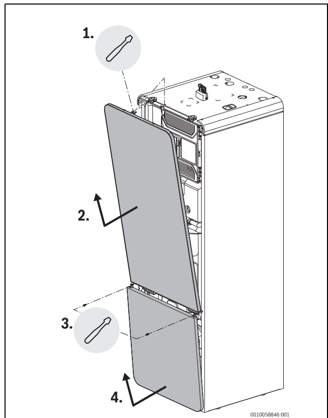
Bild 13 Frontplatte
