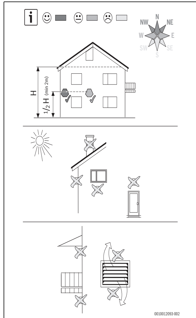
Bild 35 Position des Außentemperaturfühlers
