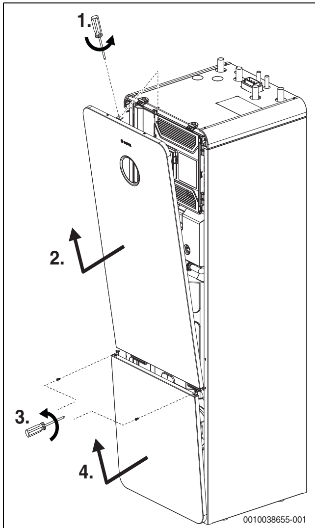
Bild 20 Front abnehmen
