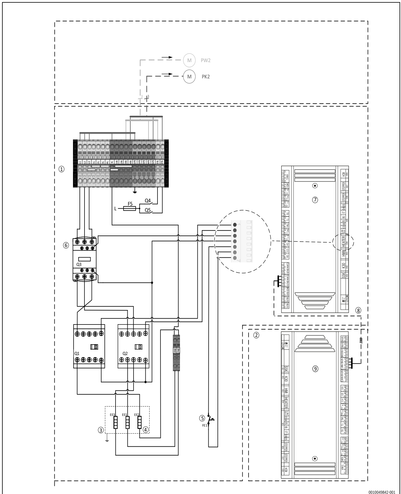
Bild 57 Spannungsversorgung Inneneinheit
