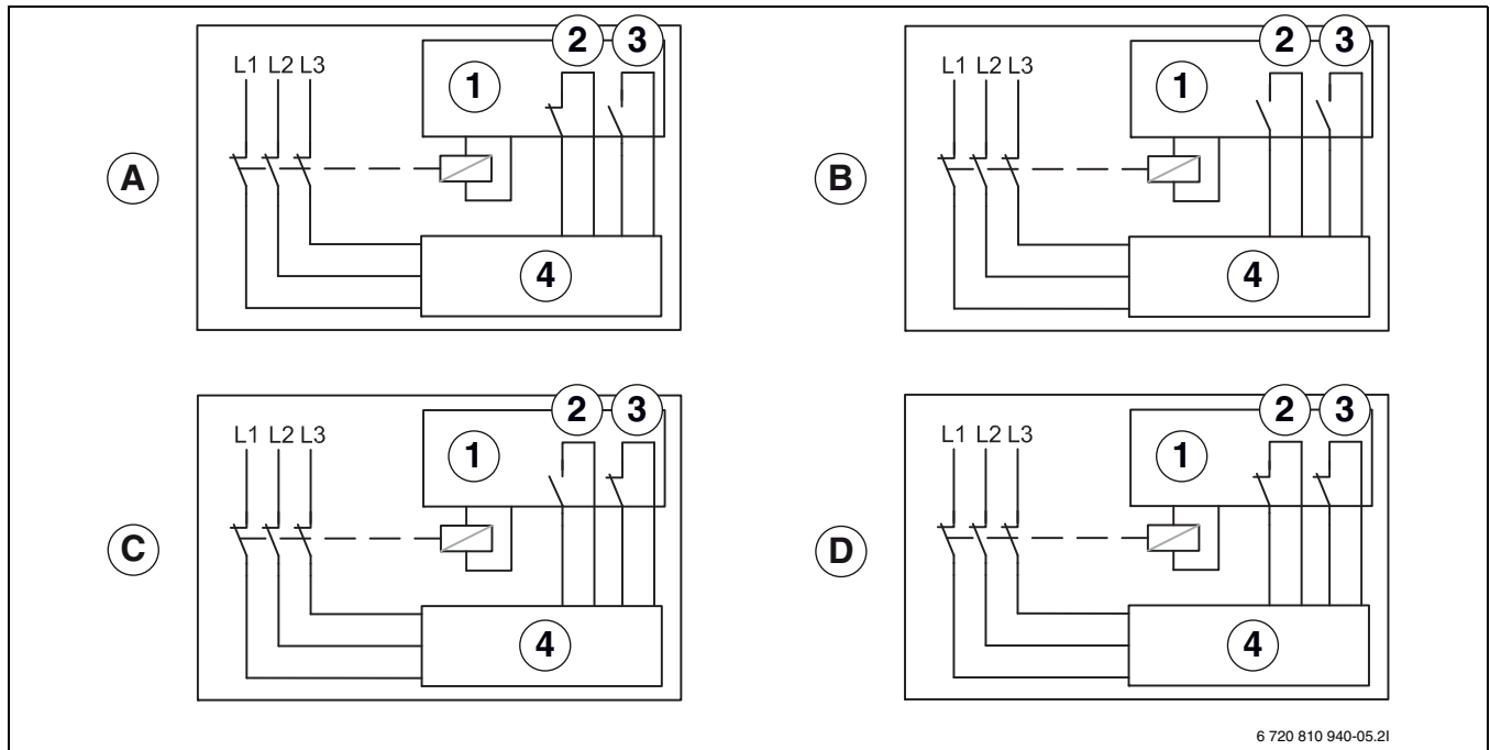
Bild 46 Anschlussplan für EVU-Sperre/SG
