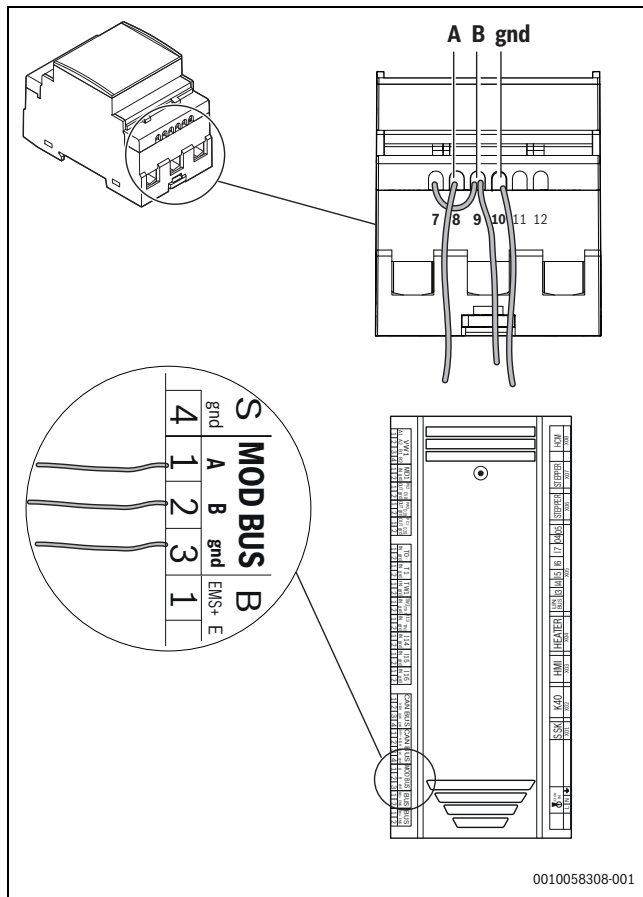
Bild 22 Power Meter 5000 an die Inneneinheit anschließen
