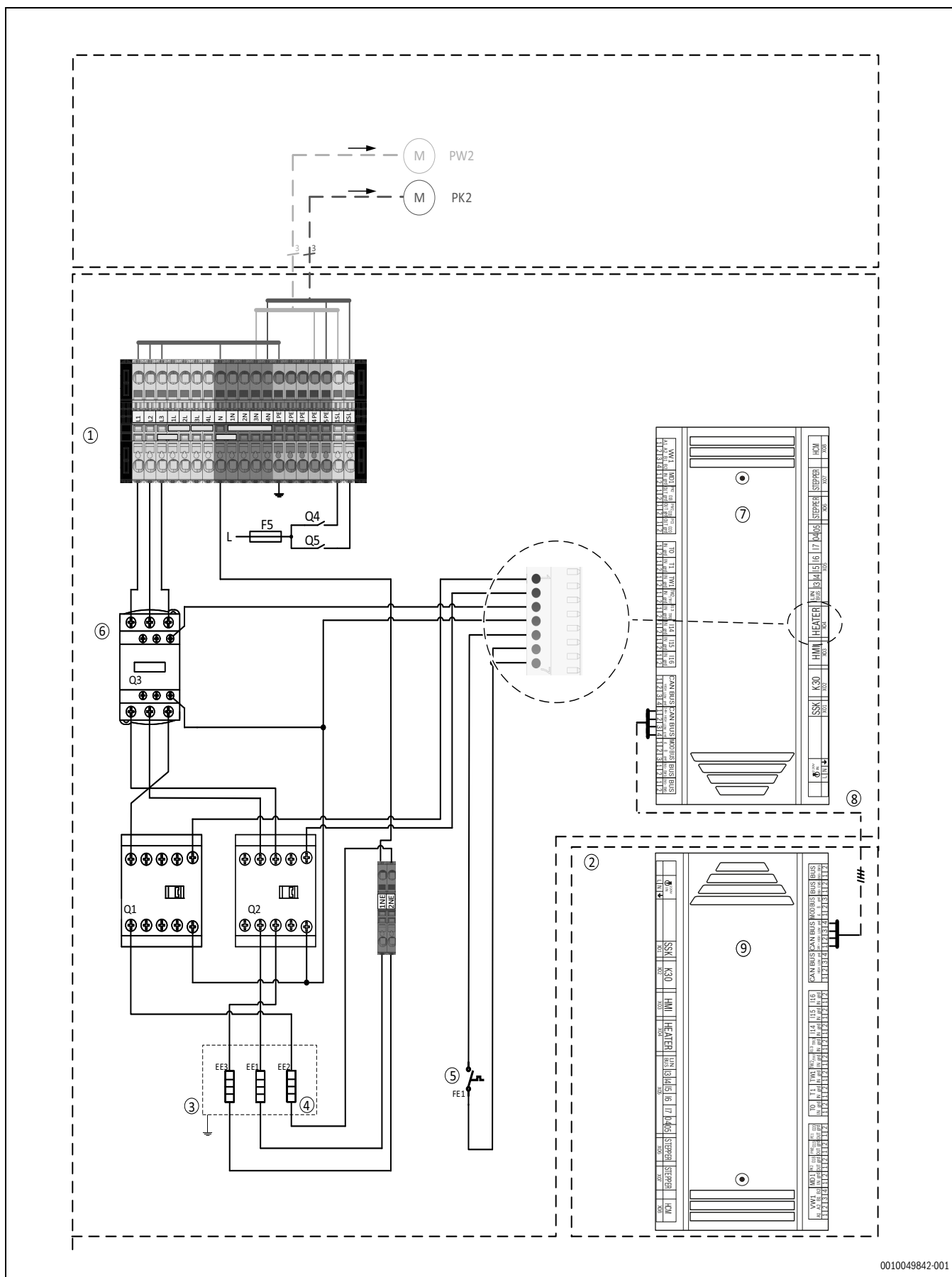
Bild 50 Spannungsversorgung Inneneinheit
