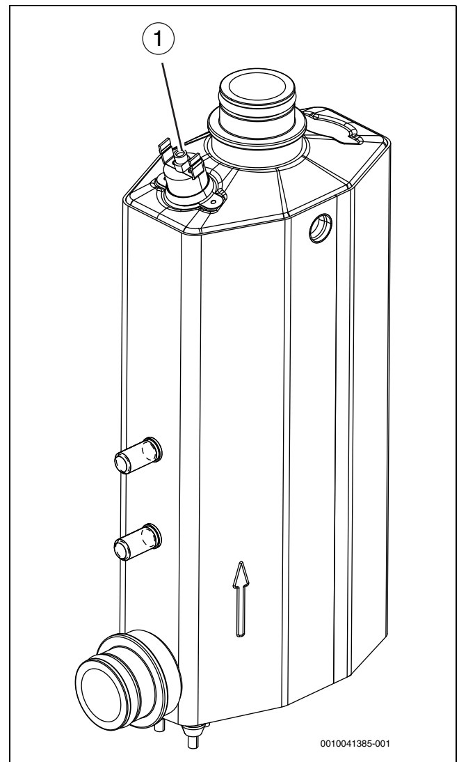
Bild 42 Elektrischer Zuheizer
