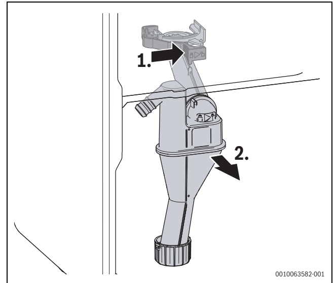
Bild 55 Siphon demontieren
