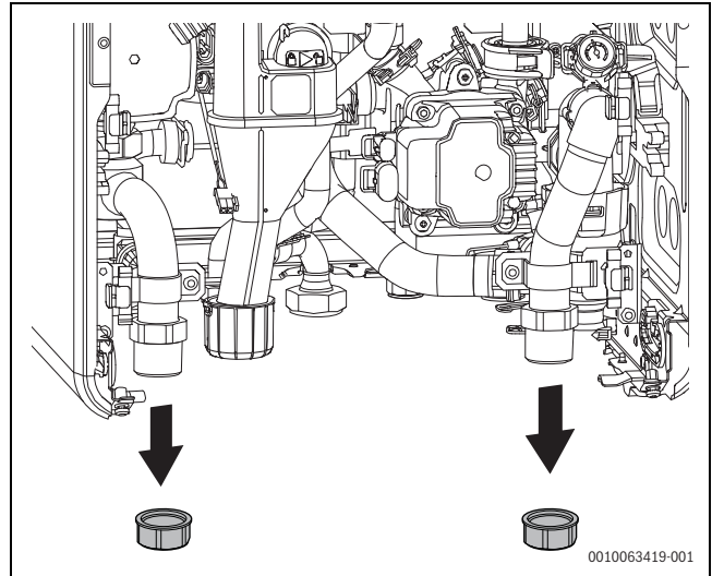
Bild 44 Kappen abnehmen
