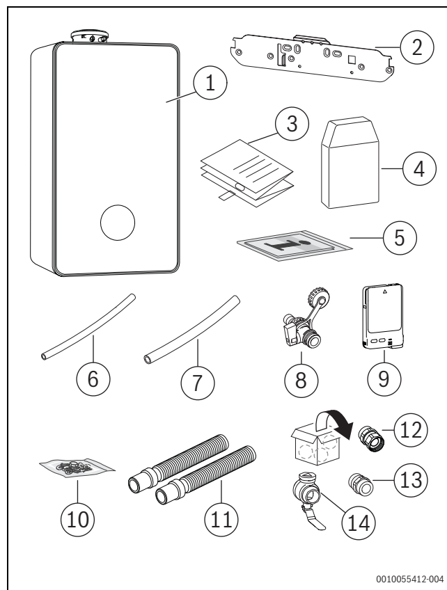
Bild 1 Lieferumfang
