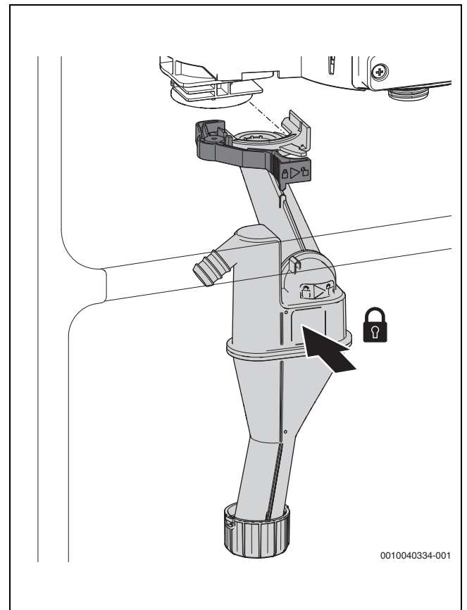
Bild 56 Siphon installieren
