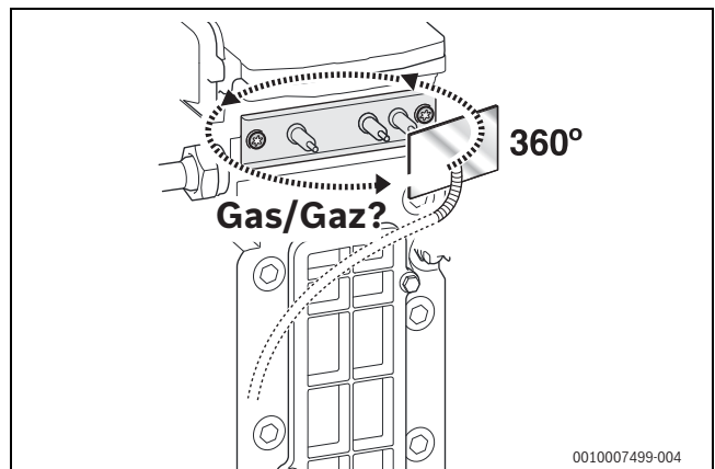
Bild 79 Dichtheit prüfen
