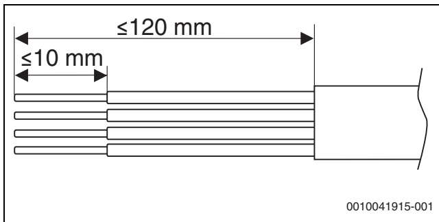
Bild 53 Abisolierung CAN-BUS
