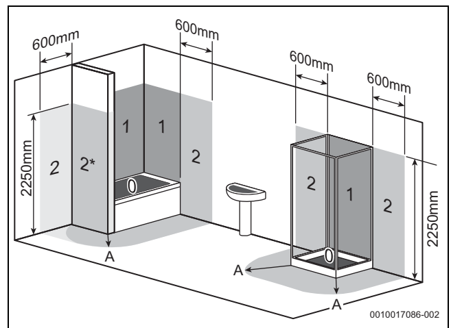
Bild 37 Schutzbereiche (Beispieldarstellung)
