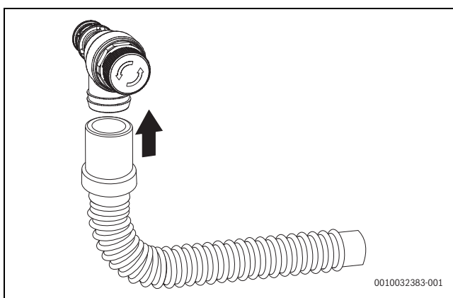
Bild 54 Schlauch am Sicherheitsventil (Heizung) montieren
