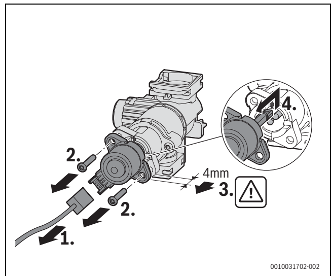
Bild 98 Motor am 3-Wege-Ventil ausbauen (Variante mit Schrauben)
