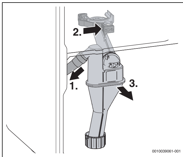
Bild 92 Siphon demontieren
