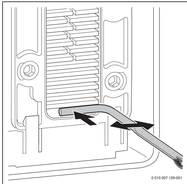
Bild 91 Kondensatwanne reinigen
