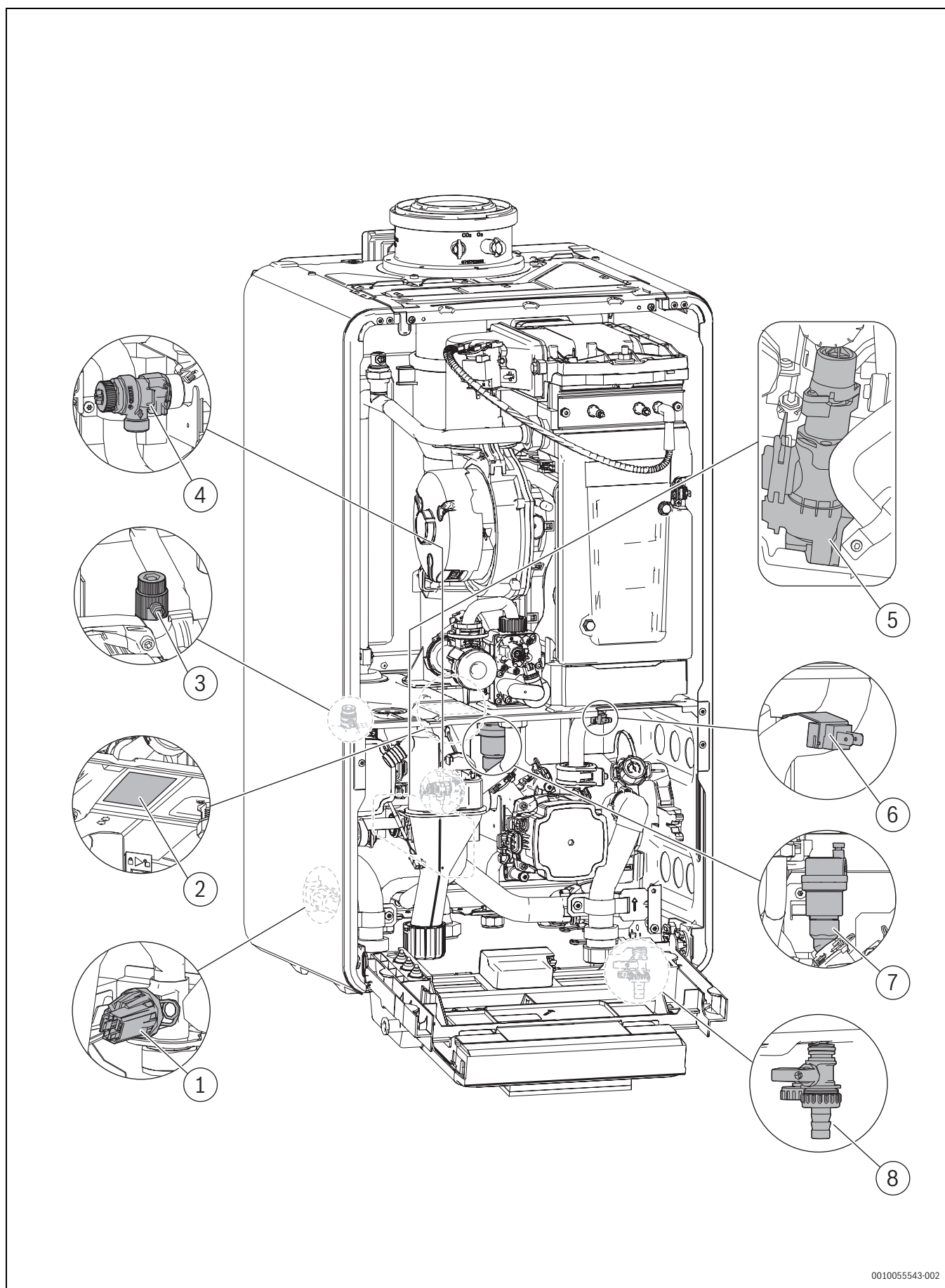
Bild 6 Produktübersicht (verdeckte Bauteile)
