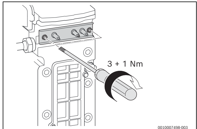
Bild 78 Elektroden-Set montieren
