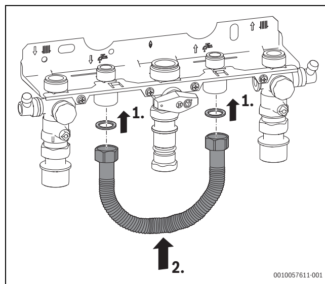
Bild 50 Warmwasser-Bypassleitung (7107800) installieren
