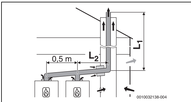
Bild 29 Kaskade mit 2 Geräten: Starre Abgasführung im Schacht nach B 53p mit raumluftabhängiger Luftzufuhr am Gerät und einwandiger Abgasleitung im Aufstellraum; Hinterlüftungsöffnung im Schacht
