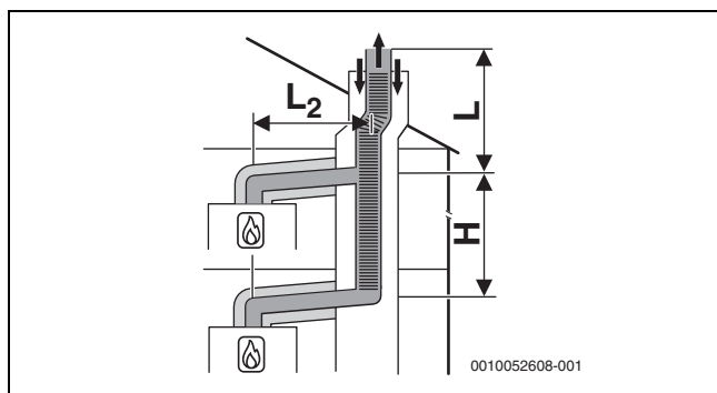
Bild 28 Mehrfachbelegung nach C_{(14)3x} mit kollektiver flexibler Abgasführung und konzentrischer Luft-Abgas-Führung im Aufstellraum
