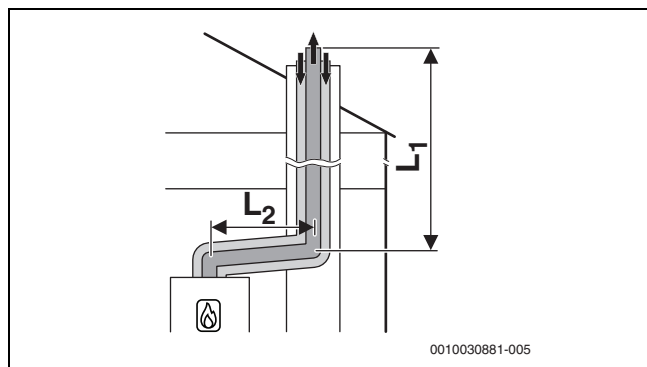
Bild 10 Konzentrische Luft-Abgas-Führung nach C 33x im Schacht
