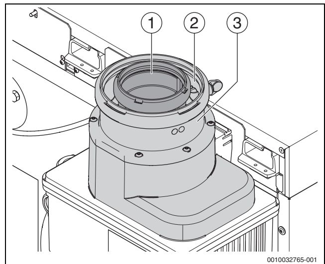
Bild 15 Abgasanschluss montieren
