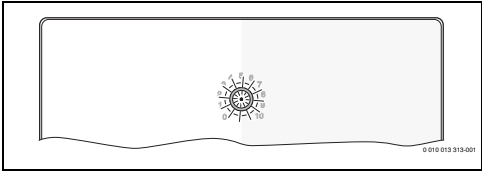
Obr. 5 Kódovací spínač
