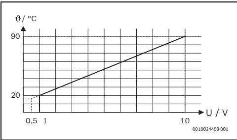
Bild 2 Linearer Zusammenhang zwischen 0-10V-Signal (U in V) und angeforderter Vorlauftemperatur (θ in °C)
