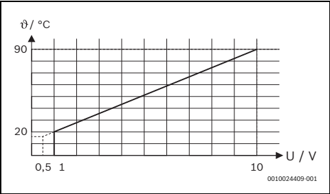
Obr. 2 Lineární závislost mezi signálem 0-10 V (U ve V) a požadovanou teplotou na výstupu (9 ve °C)
