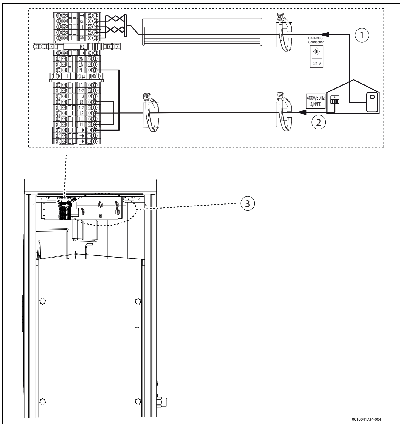
Bild 38 Anschlussklemmen im Anschlussbereich der Installation
