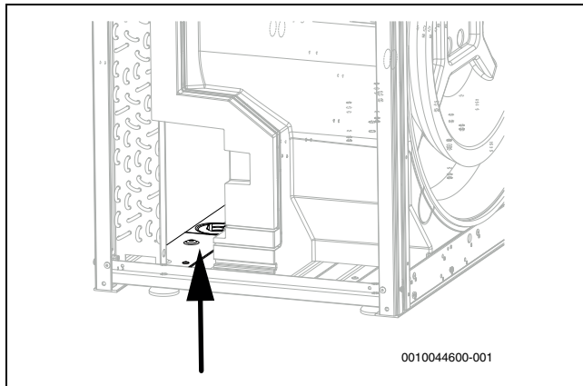
Bild 42 Tropfschale reinigen
