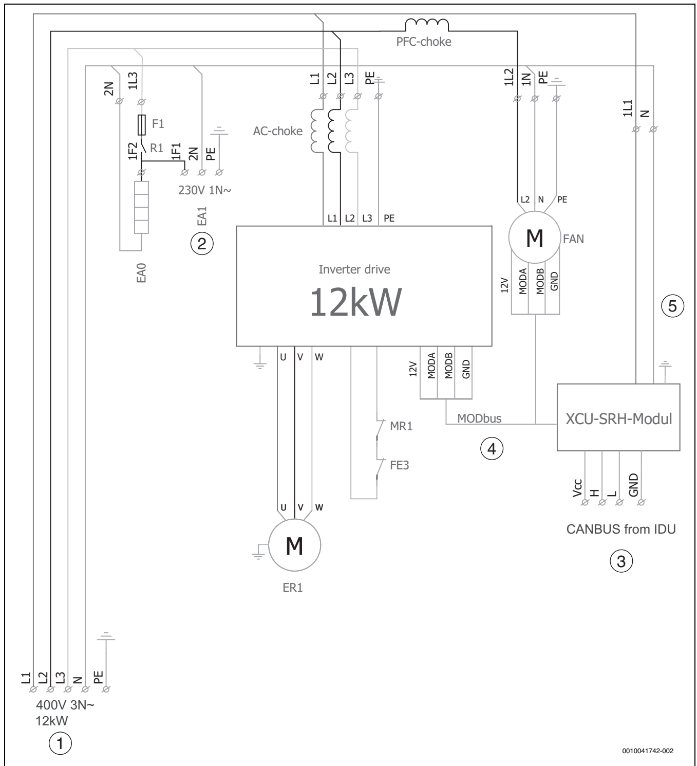
Bild 47 Schaltplan
