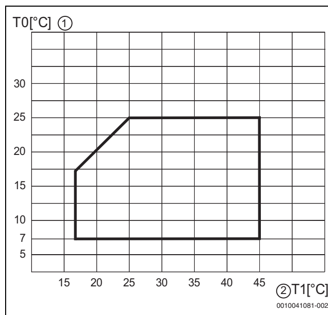
Bild 45 Wärmepumpe im Kühlbetrieb
