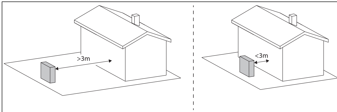
Bild 43 Abstand zur Wand
