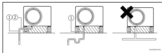
Bild 29 Kondensatableitung in die Kanalisation/den Regenablauf
