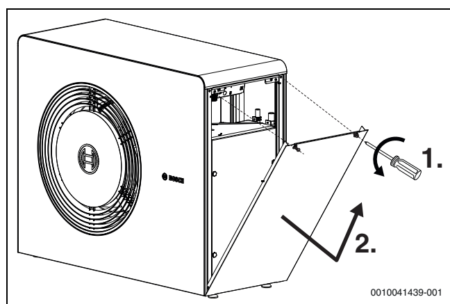
Bild 31 Seitliche Abdeckung
