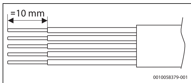
Bild 37 Kabel für den Netzanschluss abisolieren
