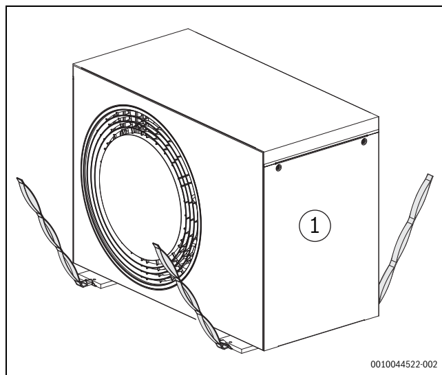
Bild 11 Beim Transportieren der Wärmepumpe ohne Verpackung die Gurte verwenden
