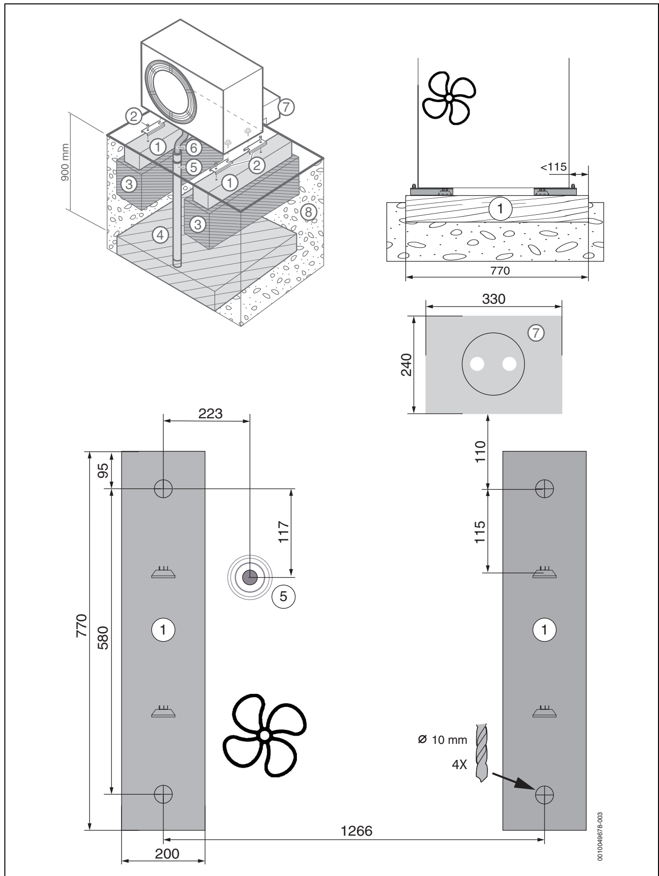
Bild 24 Fundamentplan, Alternative 1
