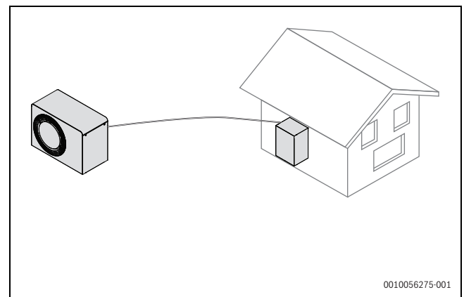
Bild 35 CAN-BUS-Verbindung zwischen Innen- und Außeneinheit
