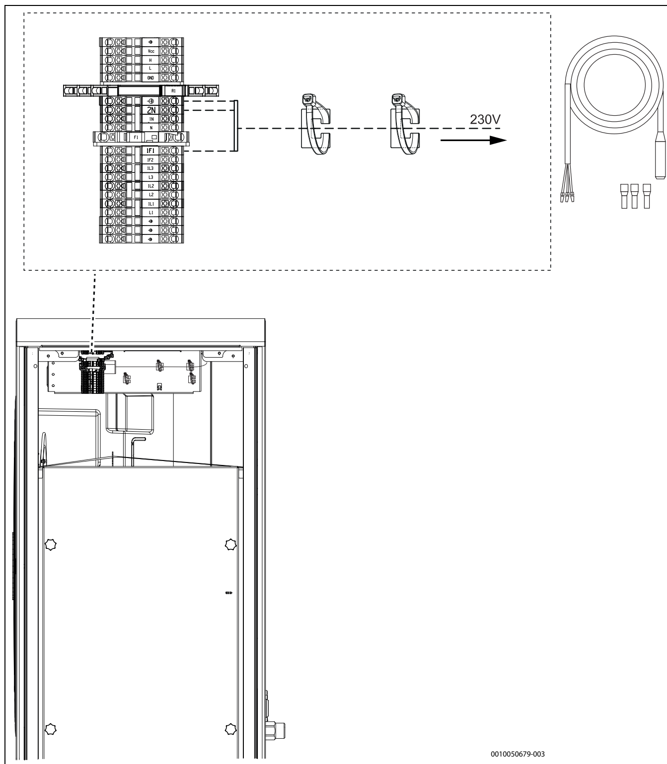
Bild 39 Heizkabelanschluss (Zubehör)
