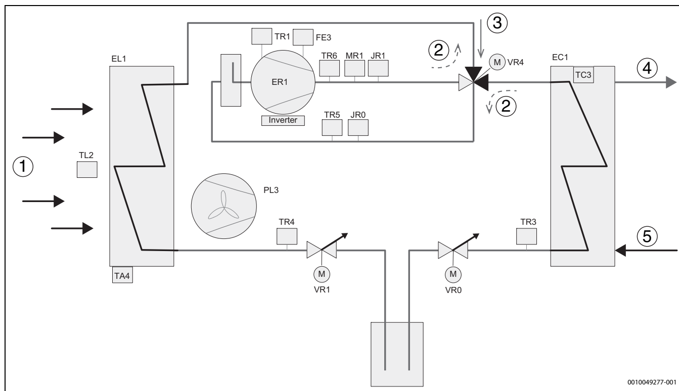
Bild 46 Kältekreis
