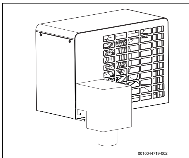
Bild 22 Installationspaket (INPA) mit Dämmschalen, bodenstehende Montage
